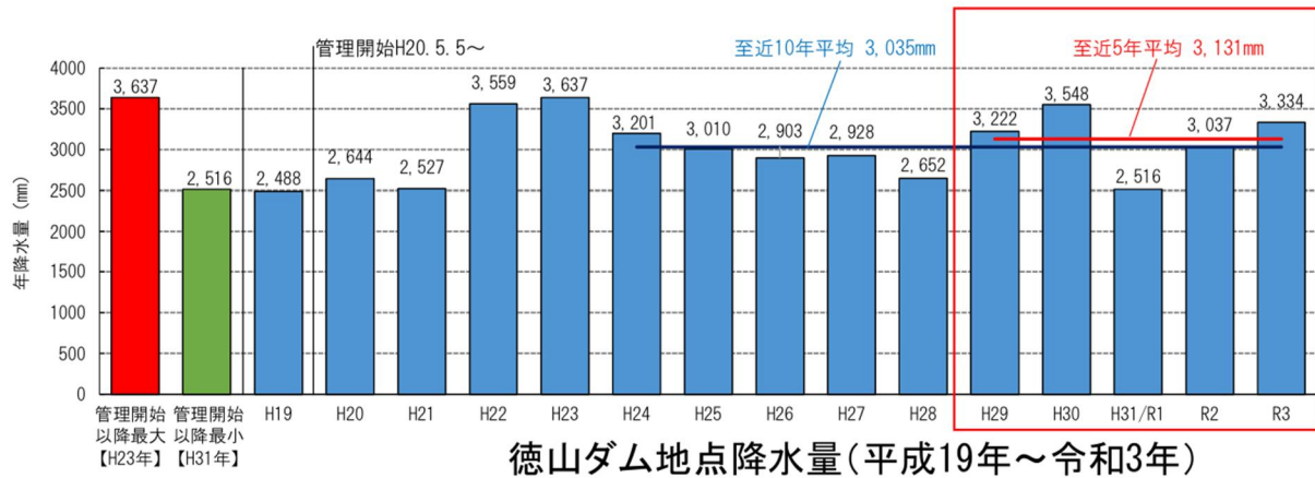
図 100 年降水量の経年変化（徳山ダム地点）
