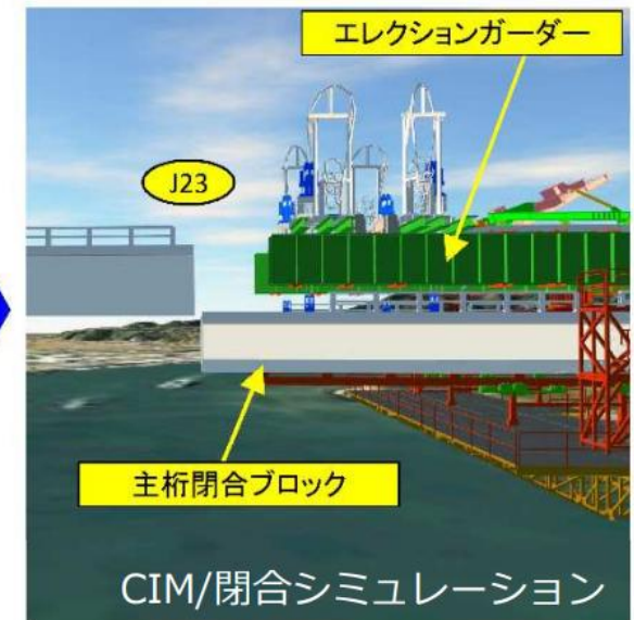
主桁の直下吊り架設～閉合シミュレーション (施工計画審査の質向上)
