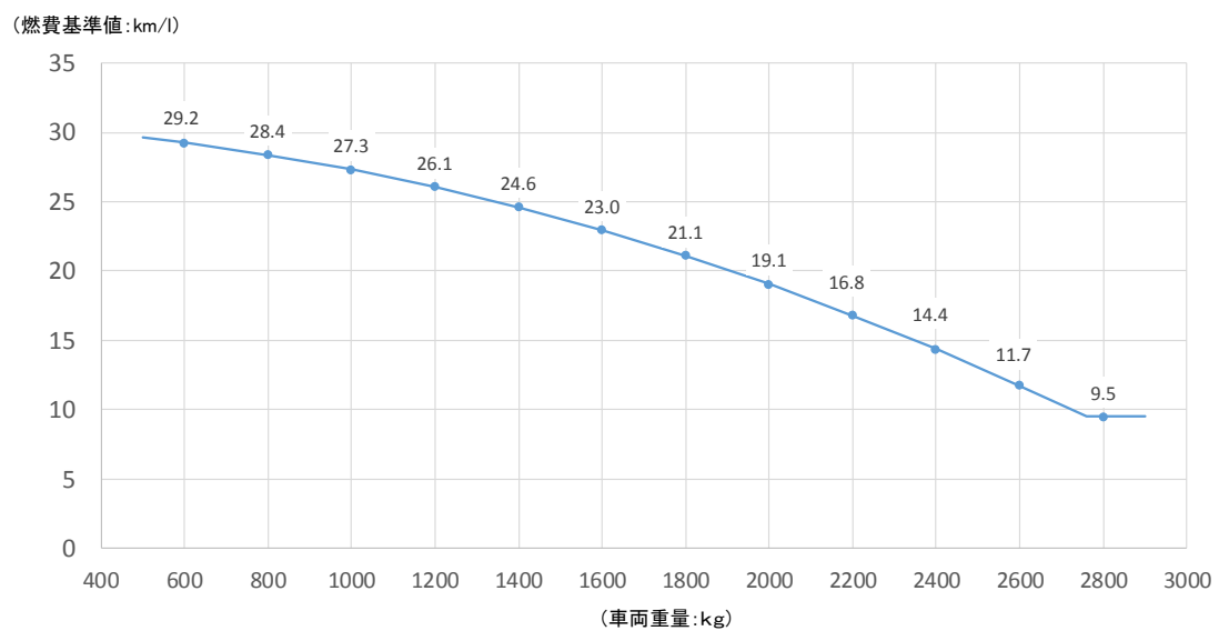
図4－2 燃費基準値の関係式
