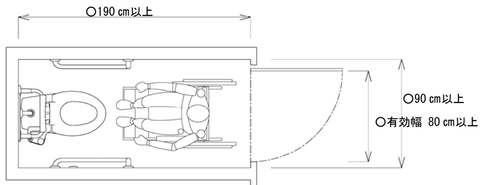
簡易型多機能便房の構造（平面図）
