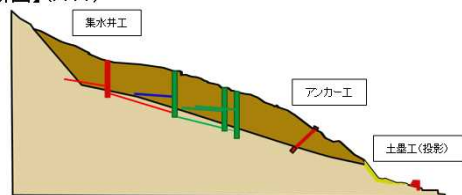
【横断面図】(A-A')
