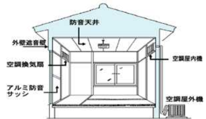
住宅の防音工事施工例
