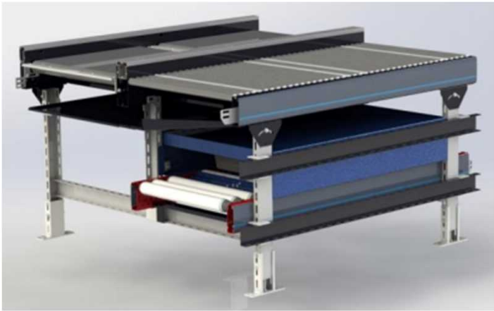
保安検査トレイ用UV殺菌装置
