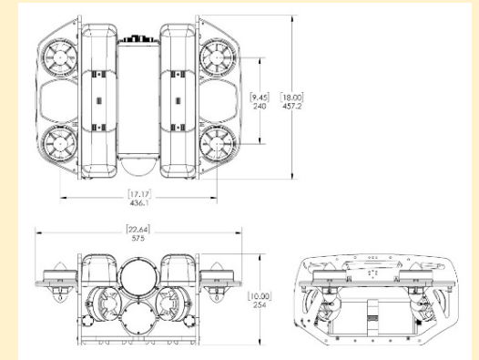
Blue ROV2
