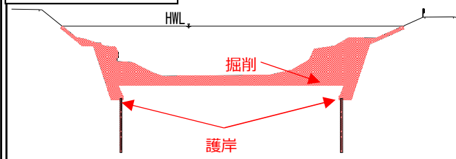
標準横断図
