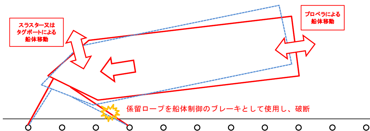
図：係留ロープ切断事例
