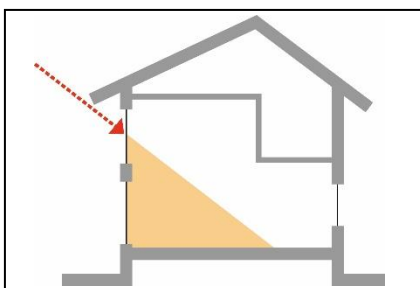
南面大開口と吹抜けの組合による日射導入
