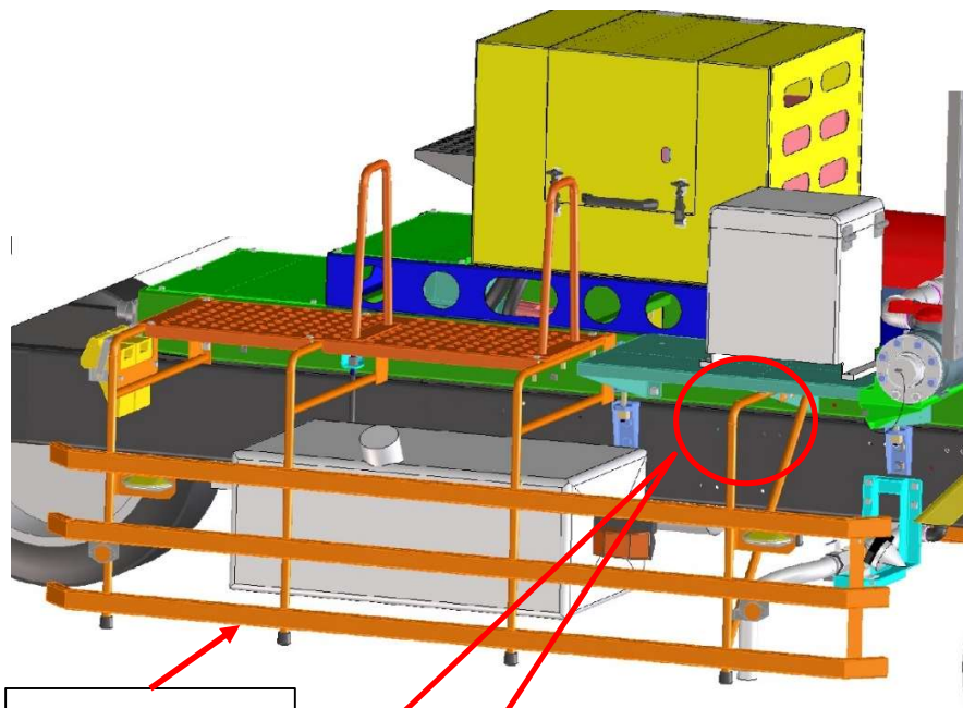
巻込防止装置
