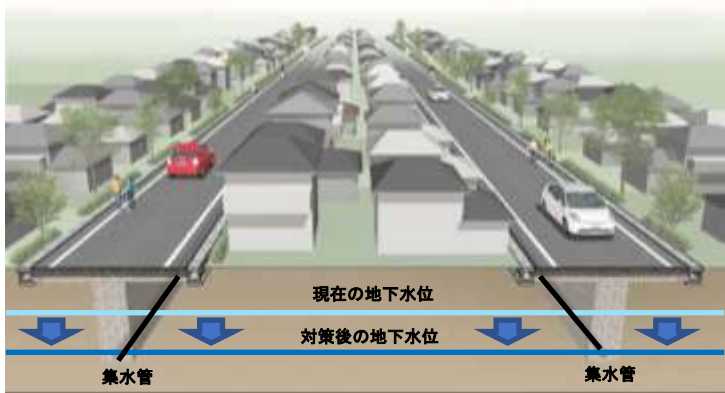
液状化対策のイメージ(地下水位低下工法)
