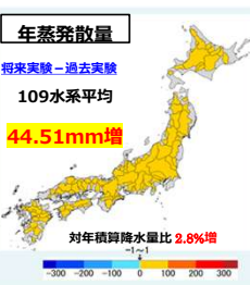
図 3.4 年蒸発散量の変化（将来実験－過去実験）[2]
