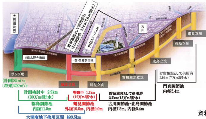
一級河川淀川水系寝屋川北部地下河川 整備の概要
