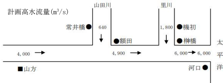
図 4-4 平成 20 年 久慈川水系河川整備基本方針の流量配分図
