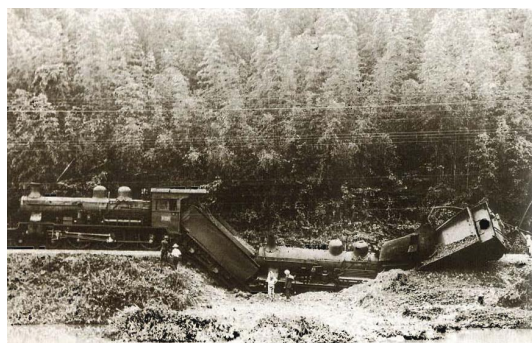
破堤し道床が流出したため、脱線した機関車 (常陸大宮市山方)
