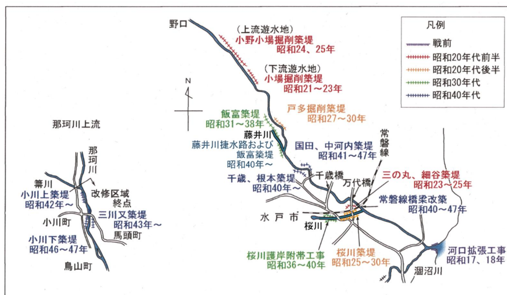
図 4-5 改修工事の変遷
