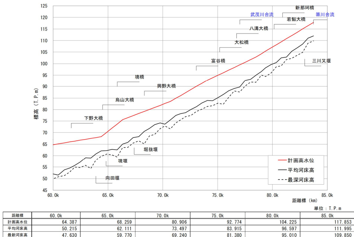
図 8-2(3) 那珂川現況河道縦断面図 (大臣管理区間 60.0k~85.0k)
