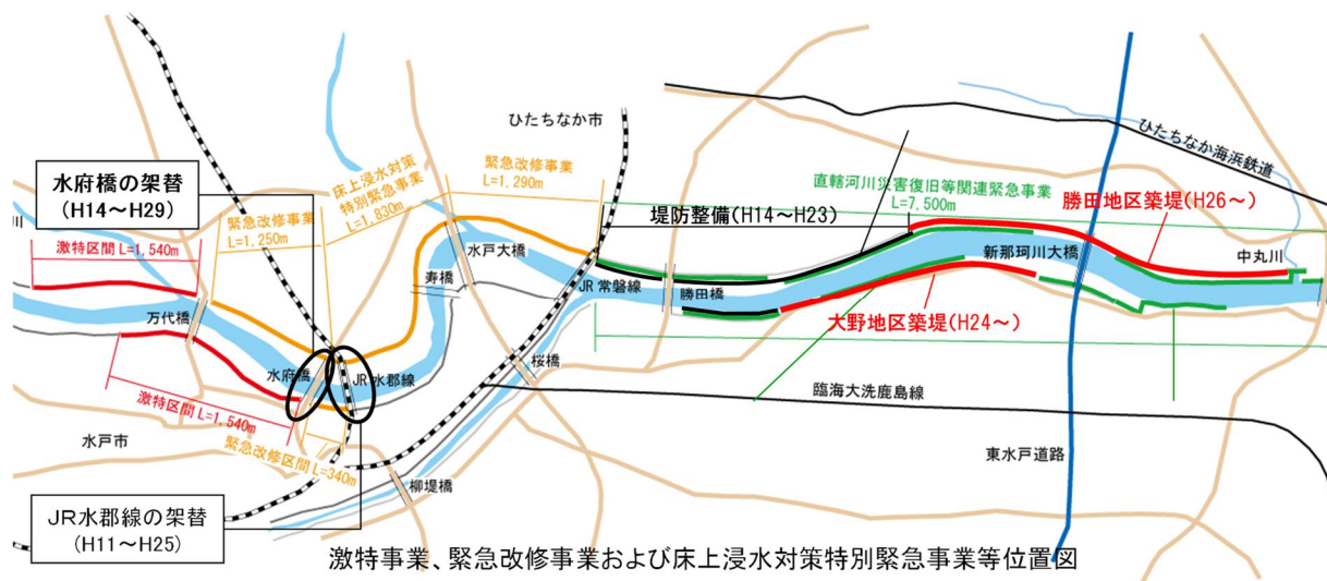
図 4-11 近年行われた那珂川下流部の治水事業の状況
