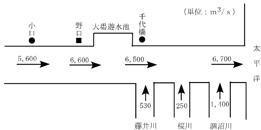
平成5年工事実施基本計画改定流量配分図（現計画） 図 4-6 那珂川大臣管理区間流量配分の変遷
