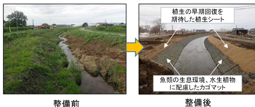
図 4-12 農業排水路の整備事例
