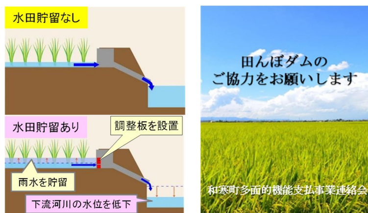
図 4-11 田んぼダムのイメージ及び普及活動
