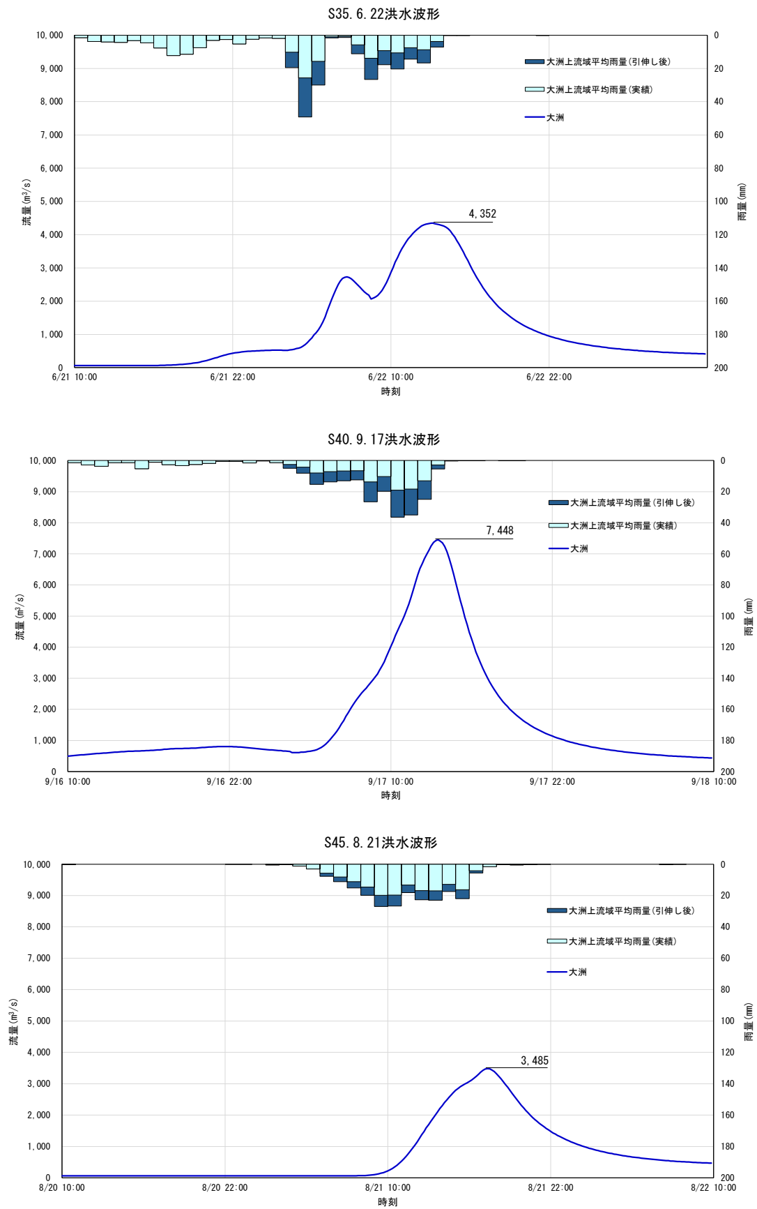
図 1.37(1) 基本高水ハイドログラフ（基準地点大洲）
