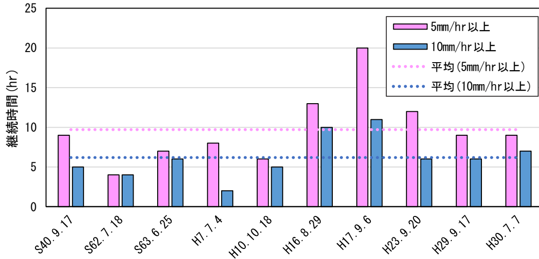
図 1.32 大洲第二地点における実績ピーク流量上位 10 洪水の 5mm/hr・10mm/hr 継続時間
