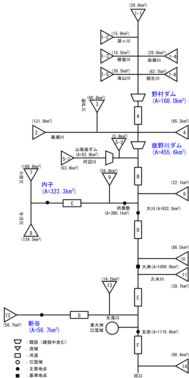
図 1.8 肱川流出モデル図と f1 \cdot Rsa 解析地点
