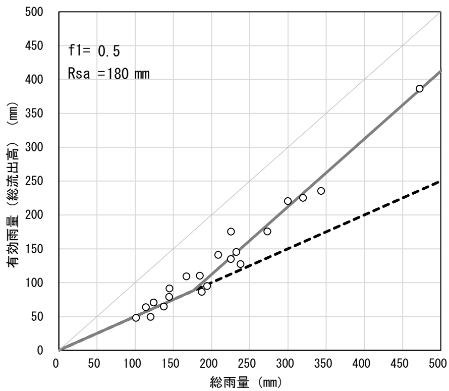
図 1.12(2) 総雨量～総流出高の関係（野村ダム～鹿野川ダム残流域）
