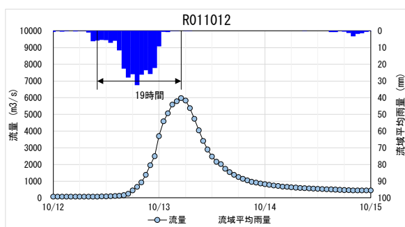
図 1-16 Kinematic Wave 法による洪水到達時間（基準地点：野口）（2/2）
