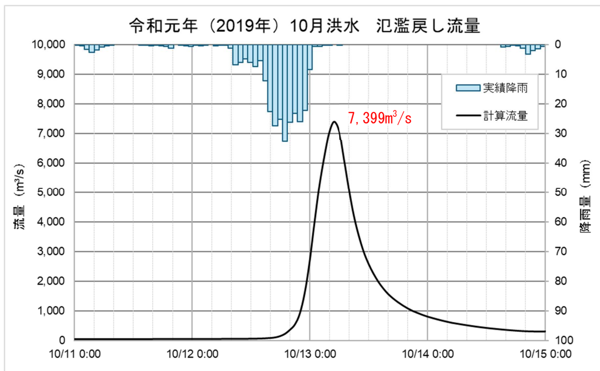
図 1-44 令和元年（2019 年）10 月洪水の氾濫戻し流量（基準地点野口）
