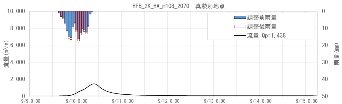
図 1-150 抽出した予測降雨波形のハイドログラフ(真勲別地点)
