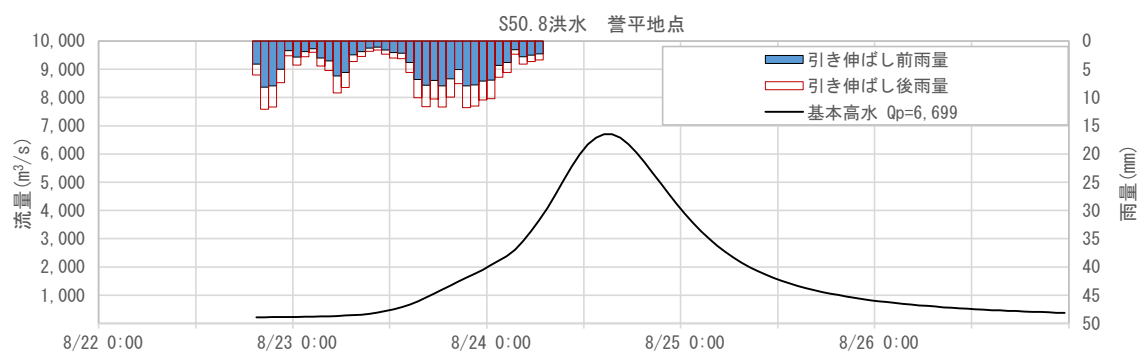
図 1-59 基本高水ハイドログラフ (昭和 50 年 8 月洪水 誉平地点)
