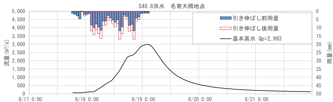
図 1-69 基本高水ハイドログラフ（昭和 48 年 8 月洪水 名寄大橋地点）
