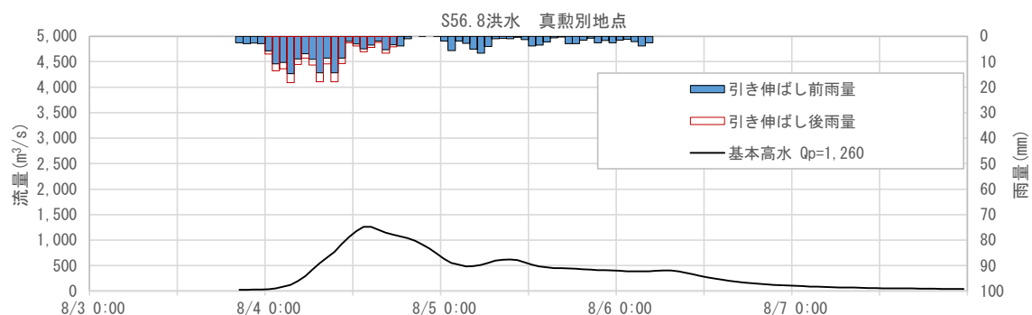
図 1-84 基本高水ハイドログラフ（昭和 56 年 8 月洪水 真勲別地点）
