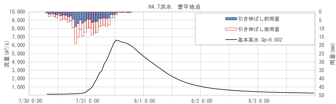
図 1-61 基本高水ハイドログラフ (平成 4 年 7 月洪水 誉平地点)
