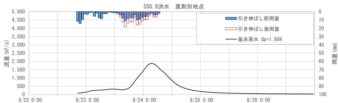
図 1-83 基本高水ハイドログラフ（昭和 50 年 8 月洪水 真勲別地点）
