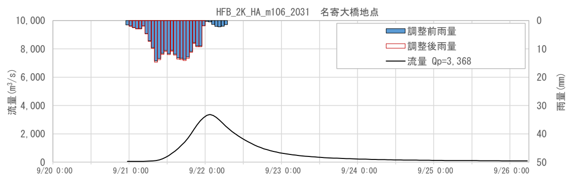
図 1-124 抽出した予測降雨波形のハイドログラフ(名寄大橋地点)
