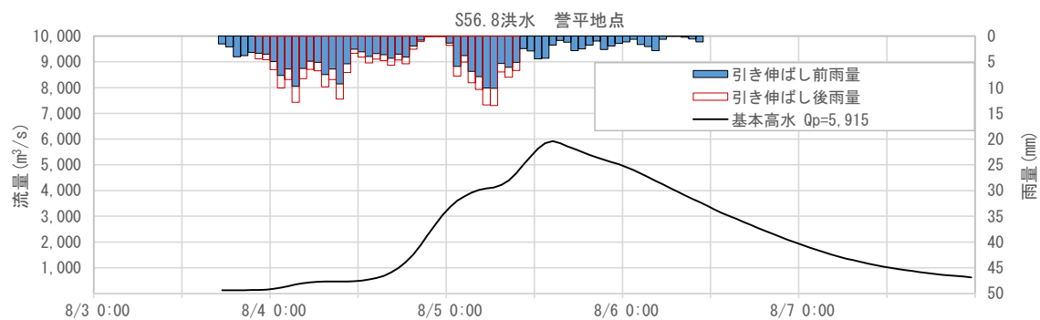
図 1-60 基本高水ハイドログラフ (昭和 56 年 8 月洪水 誉平地点)
