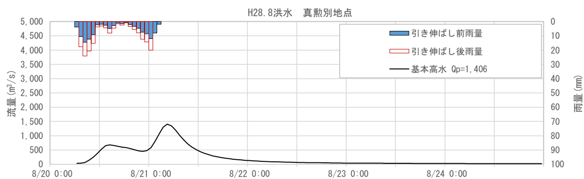
図 1-95 基本高水ハイドログラフ (平成 28 年 8 月洪水 真勲別地点)
