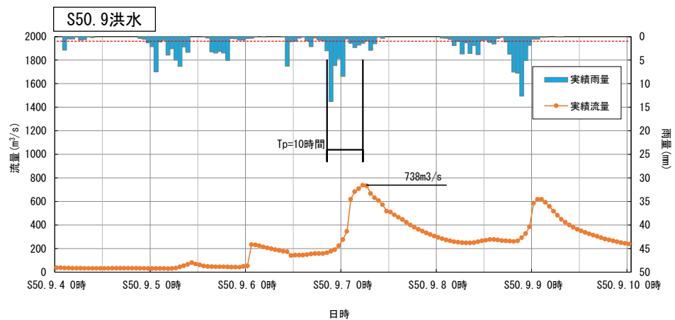
図 1-36 Kinematic Wave 法による洪水到達時間(真敷別地点)
