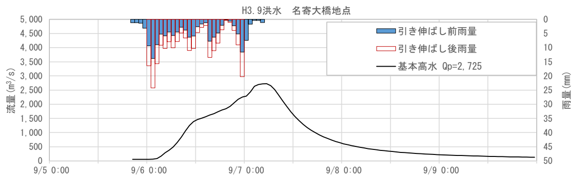
図 1-73 基本高水ハイドログラフ（平成 3 年 9 月洪水 名寄大橋地点）
