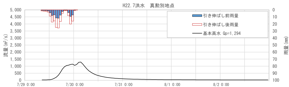
図 1-91 基本高水ハイドログラフ（平成 22 年 7 月洪水 真勲別地点）
