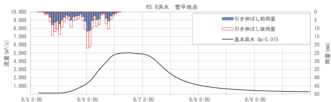
図 1-67 基本高水ハイドログラフ (令和 5 年 8 月洪水 誉平地点)
