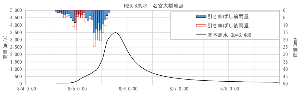
図 1-79 基本高水ハイドログラフ（平成 26 年 8 月洪水 名寄大橋地点）
