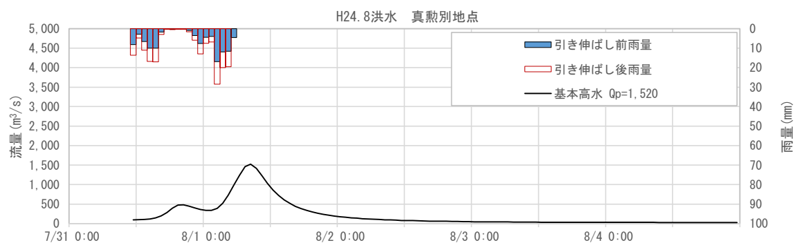
図 1-93 基本高水ハイドログラフ (平成 24 年 7 月洪水 真勲別地点)
