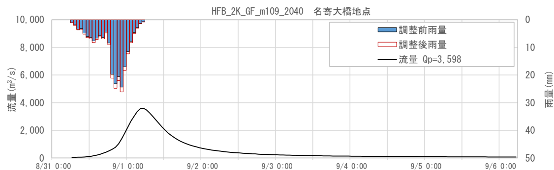
図 1-126 抽出した予測降雨波形のハイドログラフ(名寄大橋地点)
