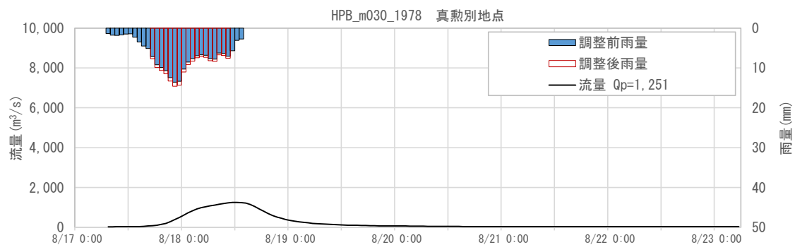
図 1-157 抽出した予測降雨波形のハイドログラフ(真敷別地点)
