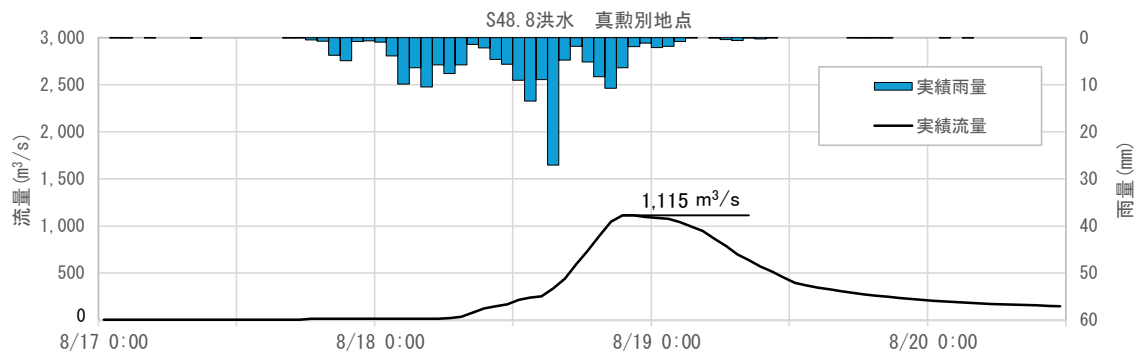
図 1-167 昭和 48 年 8 月洪水の推定結果(真勲別地点)
