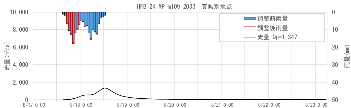
図 1-143 抽出した予測降雨波形のハイドログラフ(真敷別地点)
