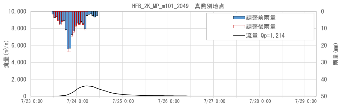
図 1-149 抽出した予測降雨波形のハイドログラフ(真勲別地点)
