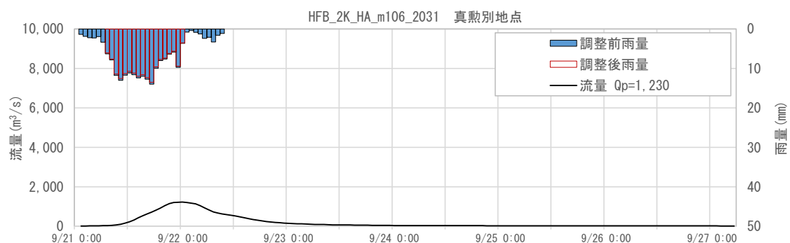
図 1-144 抽出した予測降雨波形のハイドログラフ(真敷別地点)
