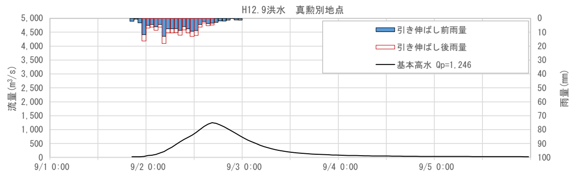
図 1-88 基本高水ハイドログラフ (平成12年9月洪水 真敷別地点)
