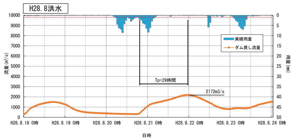
図 1-31 Kinematic Wave 法による洪水到達時間(誉平地点)
