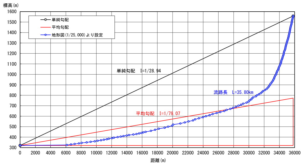
図 1-21 河道延長、平均勾配算定結果（岩尾内ダム）
