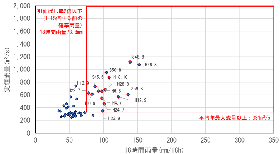
図 1-56 対象洪水の選定結果(真勲別地点)
