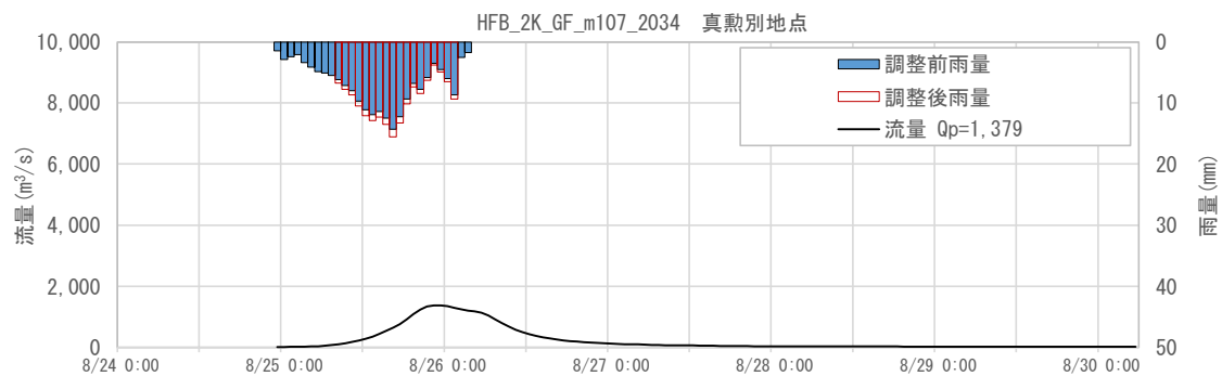
図 1-151 抽出した予測降雨波形のハイドログラフ(真熟別地点)
