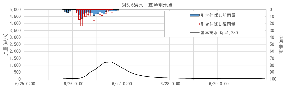
図 1-81 基本高水ハイドログラフ（昭和 45 年 6 月洪水 真勲別地点）
