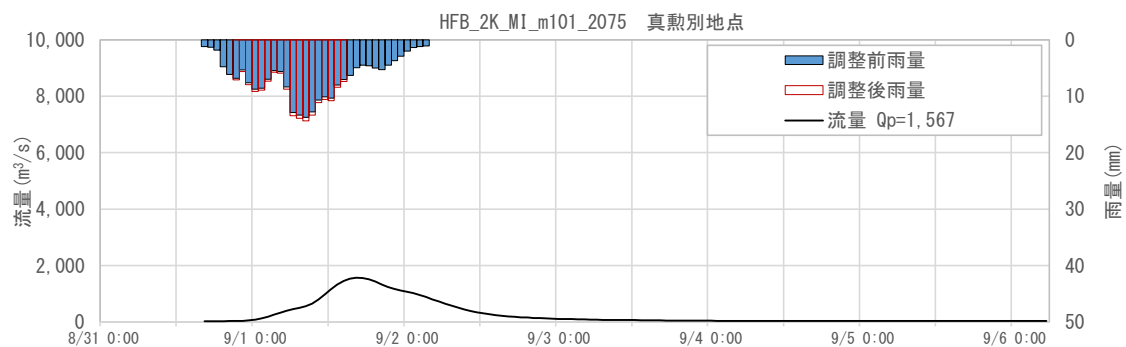
図 1-145 抽出した予測降雨波形のハイドログラフ(真敷別地点)
