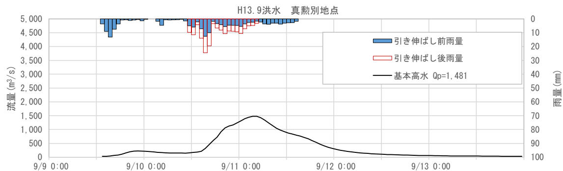
図 1-89 基本高水ハイドログラフ（平成 13 年 9 月洪水 真勲別地点）
