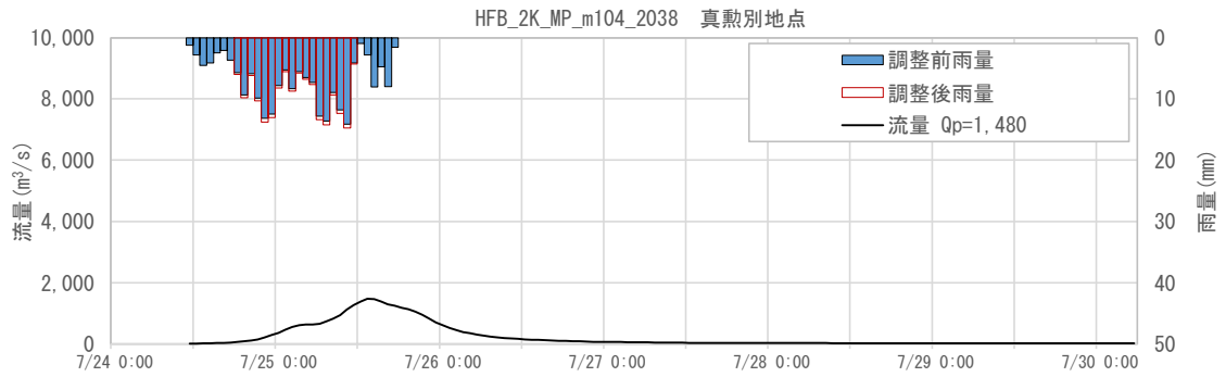
図 1-147 抽出した予測降雨波形のハイドログラフ(真勲別地点)
