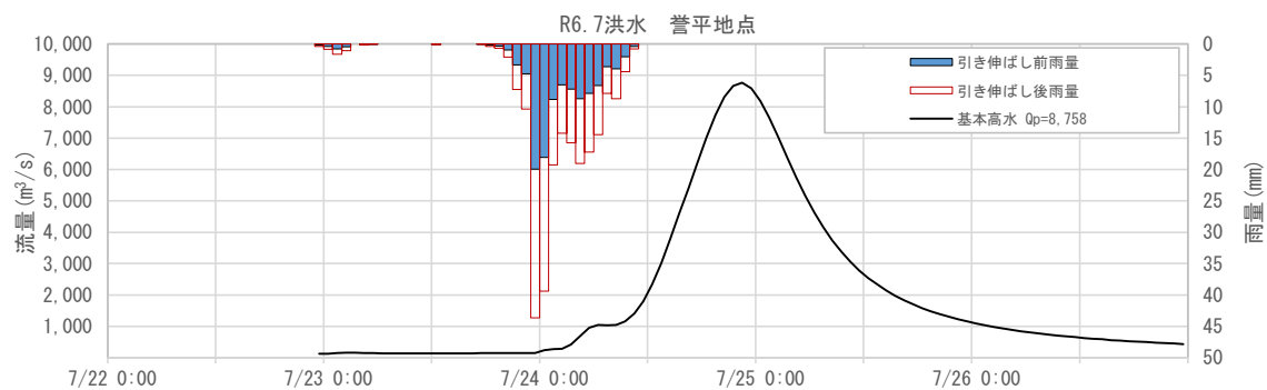
図 1-68 基本高水ハイドログラフ (令和 6 年 7 月洪水 誉平地点)
