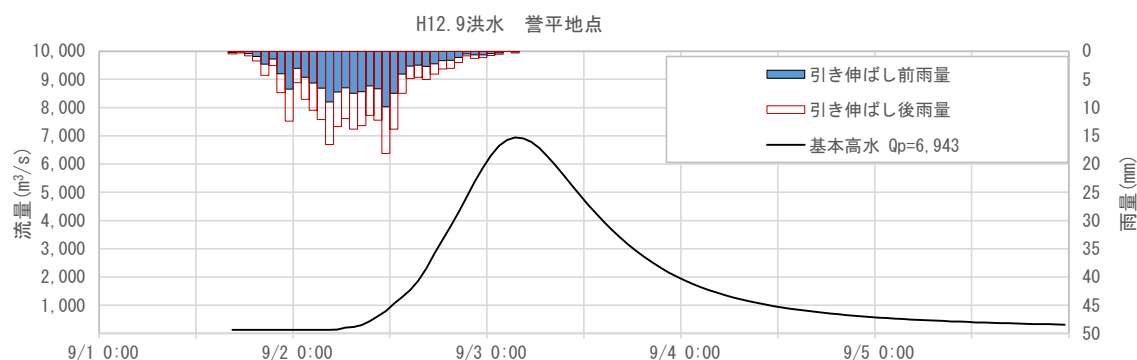
図 1-169 基本高水のピーク流量ハイドログラフ(平成 12 年 9 月洪水 誉平地点)
