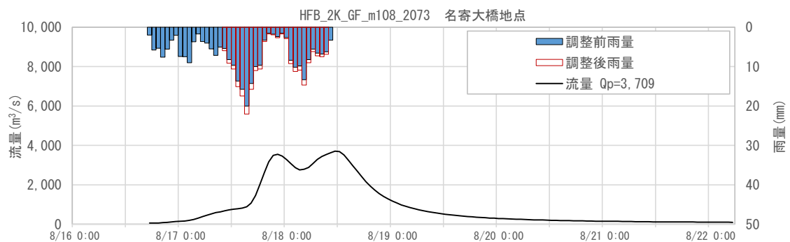
図 1-128 抽出した予測降雨波形のハイドログラフ(名寄大橋地点)
