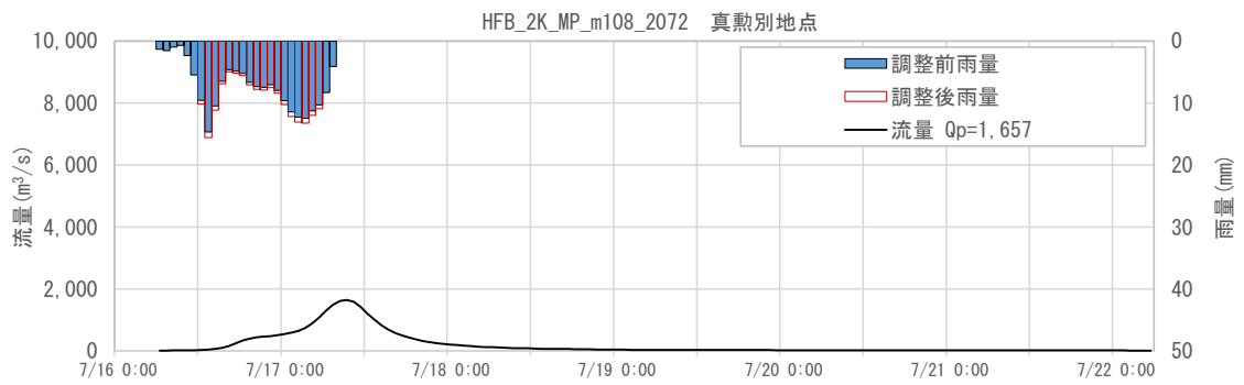
図 1-148 抽出した予測降雨波形のハイドログラフ(真勲別地点)
