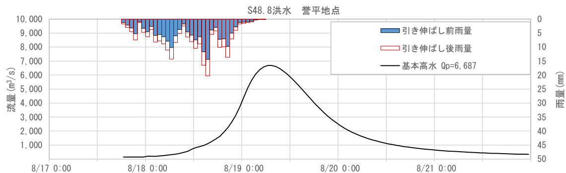
図 1-58 基本高水ハイドログラフ (昭和 48 年 8 月洪水 誉平地点)
