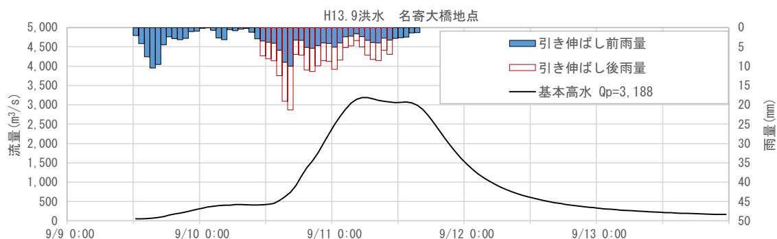
図 1-76 基本高水ハイドログラフ（平成 13 年 9 月洪水 名寄大橋地点）
