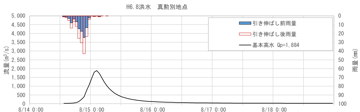
図 1-173 基本高水のピーク流量ハイドログラフ(平成 6 年 8 月洪水 真勲別地点)
