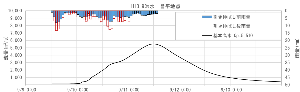
図 1-63 基本高水ハイドログラフ (平成 13 年 9 月洪水 誉平地点)
