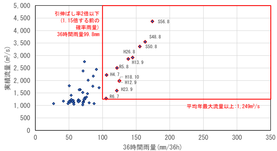
図 1-54 対象洪水の選定結果(菅平地点)
