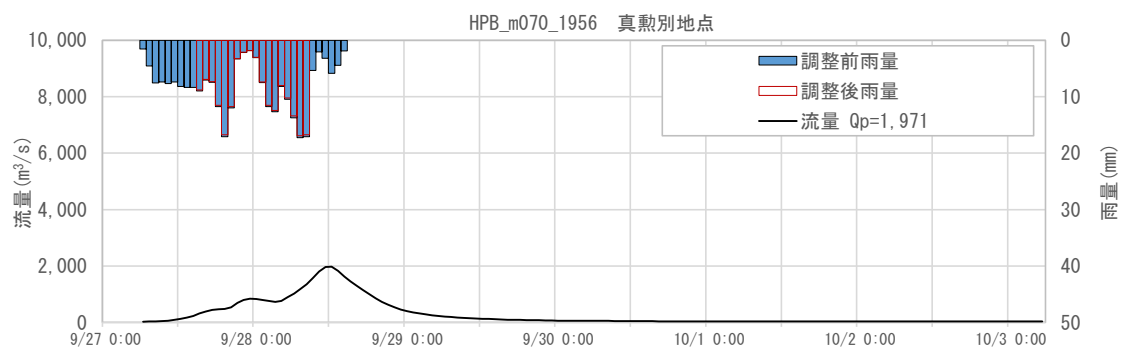
図 1-154 抽出した予測降雨波形のハイドログラフ(真熟別地点)
