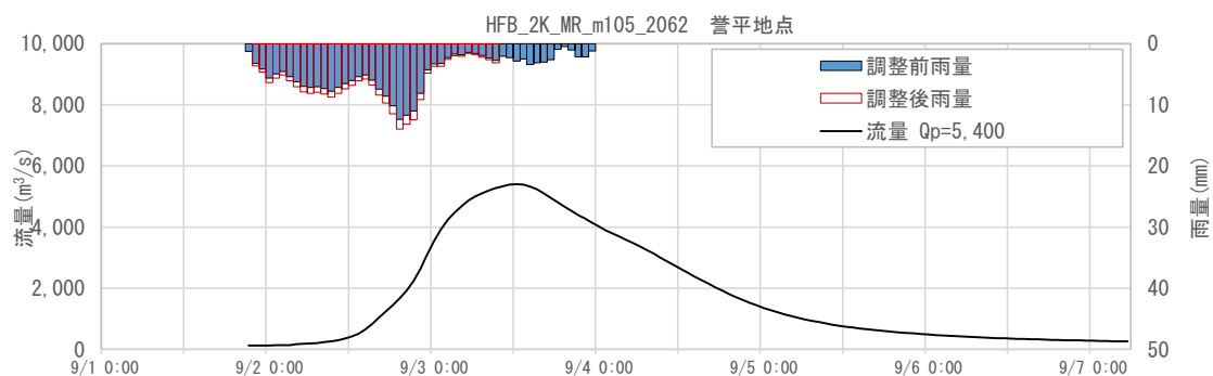
図 1-110 抽出した予測降雨波形のハイドログラフ(誉平地点)
