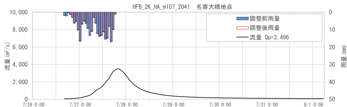
図 1-125 抽出した予測降雨波形のハイドログラフ(名寄大橋地点)
