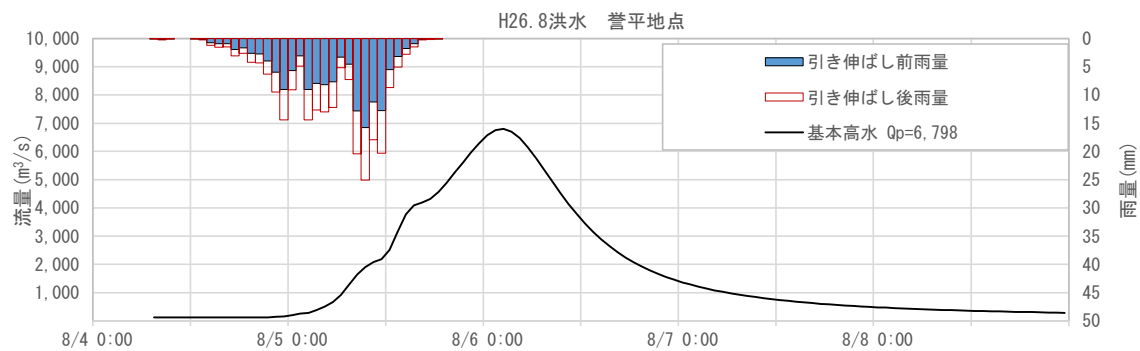
図 1-66 基本高水ハイドログラフ (平成 26 年 8 月洪水 誉平地点)
