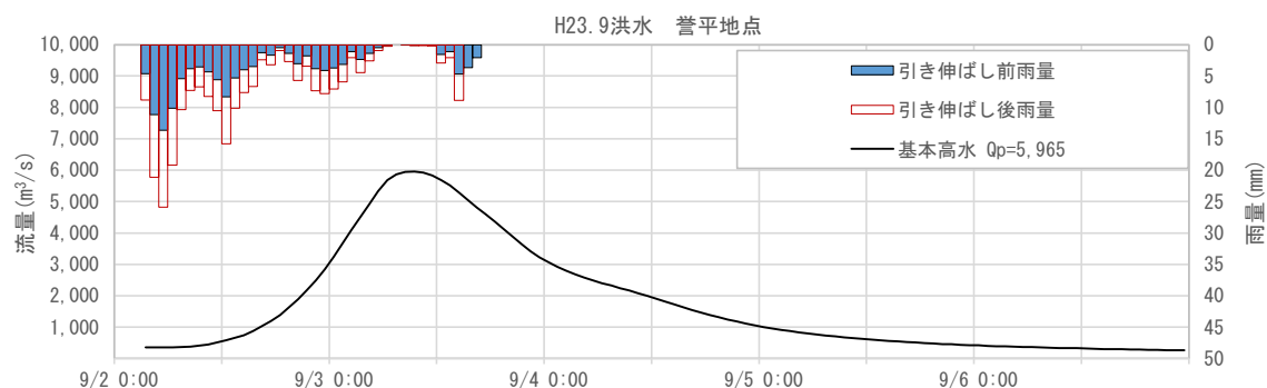
図 1-65 基本高水ハイドログラフ (平成 23 年 9 月洪水 誉平地点)
