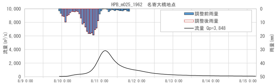
図 1-131 抽出した予測降雨波形のハイドログラフ(名寄大橋地点)
