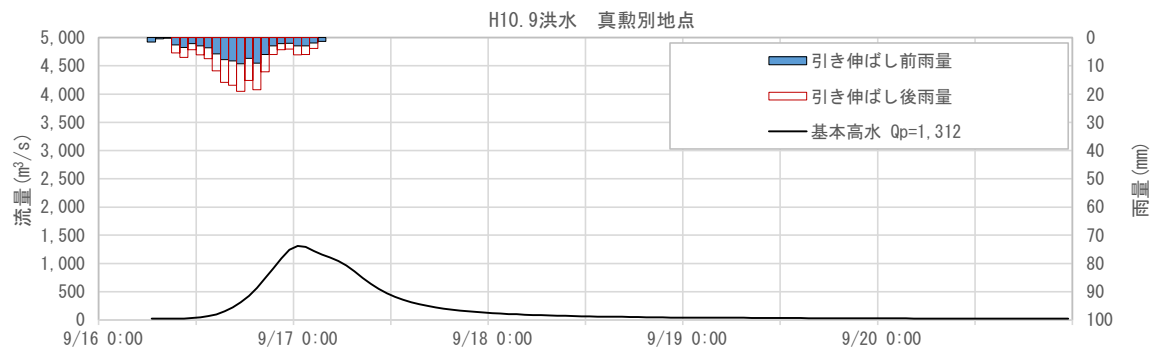
図 1-87 基本高水ハイドログラフ (平成10年9月洪水 真敷別地点)
