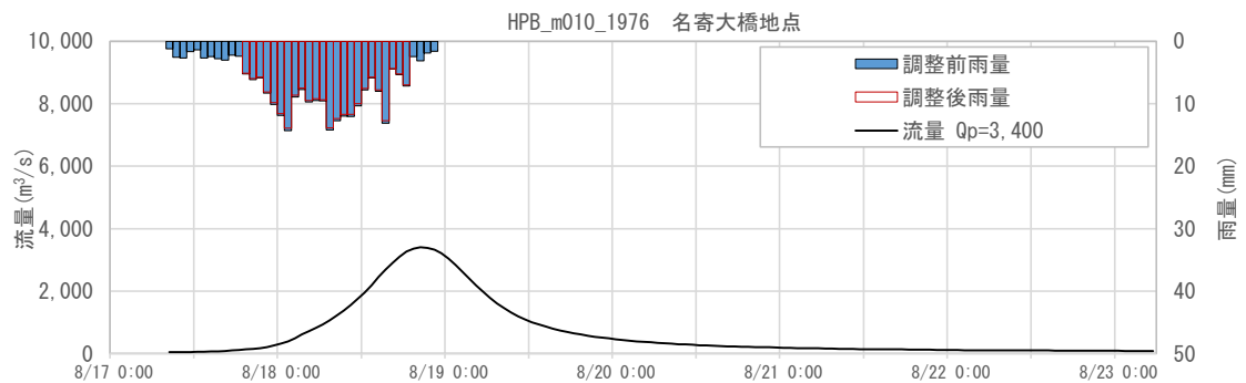
図 1-134 抽出した予測降雨波形のハイドログラフ(名寄大橋地点)
