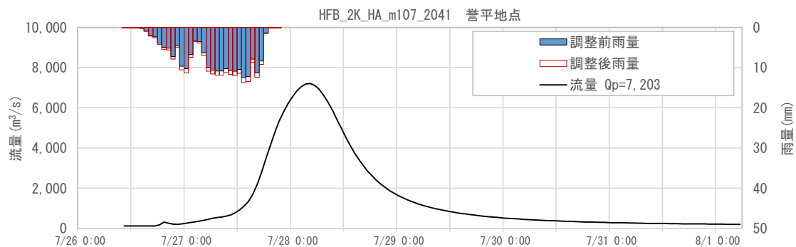
図 1-107 抽出した予測降雨波形のハイドログラフ(誉平地点)
