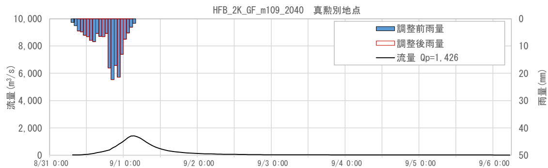
図 1-139 抽出した予測降雨波形のハイドログラフ(真勲別地点)
