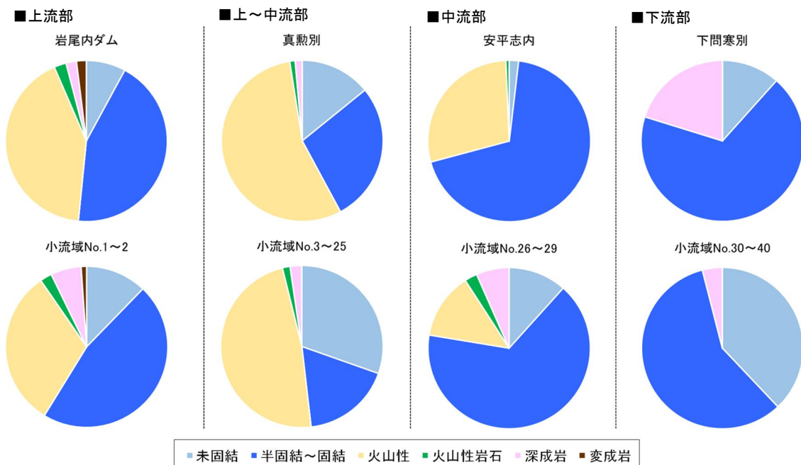
図 1-25 各流域の地質分布
