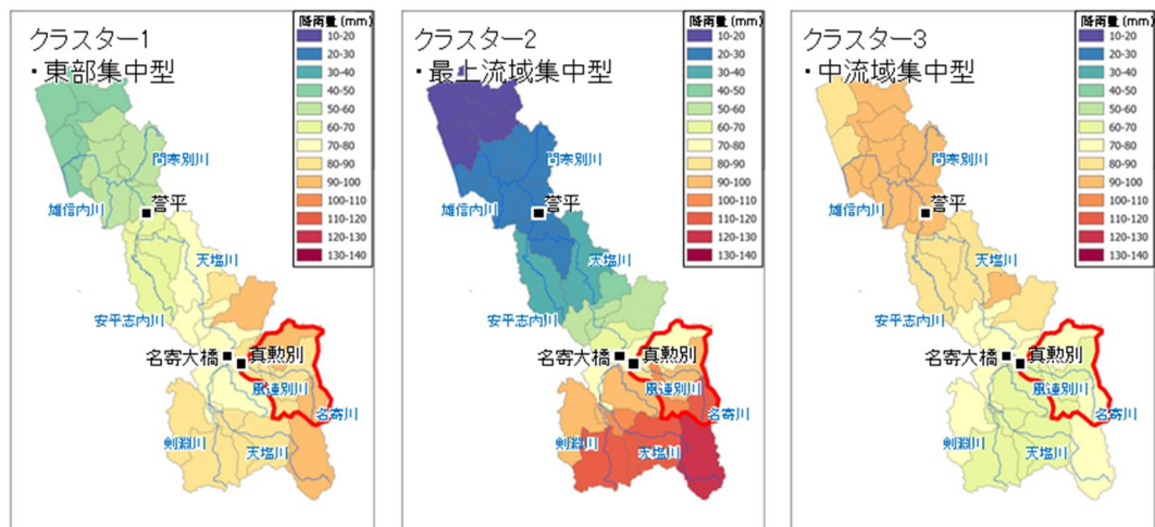
図 1-163 真熟別地点における将来実験アンサンブル予測降雨のクラスター分析結果
