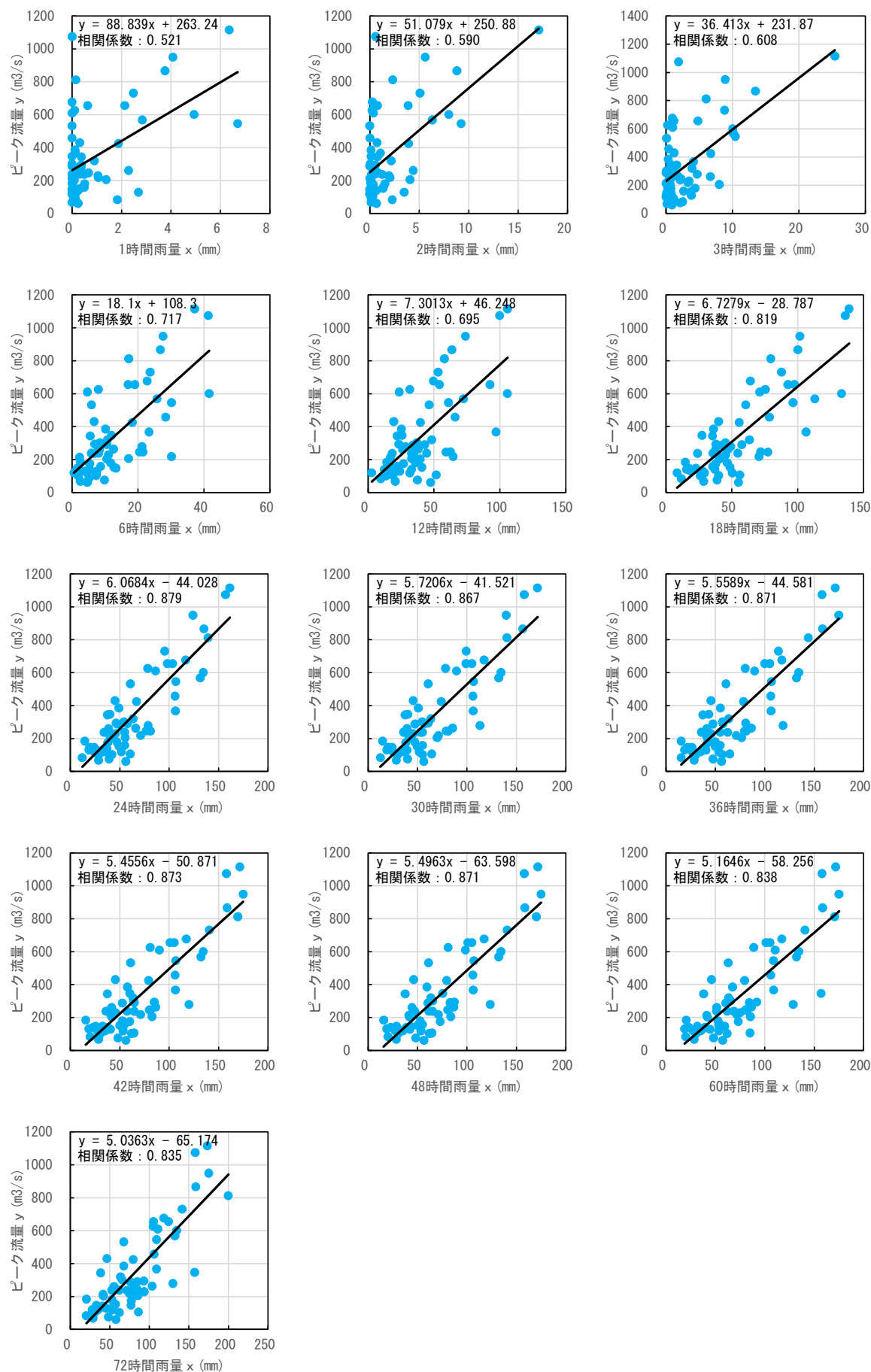
図 1-47 ピーク流量と流域平均時間雨量の相関図【定義②】（真熟別地点）
