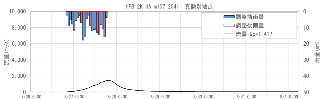
図 1-146 抽出した予測降雨波形のハイドログラフ(真敷別地点)
