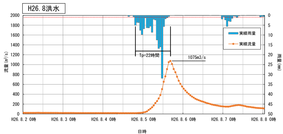
図 1-37 Kinematic Wave 法による洪水到達時間(真熟別地点)
