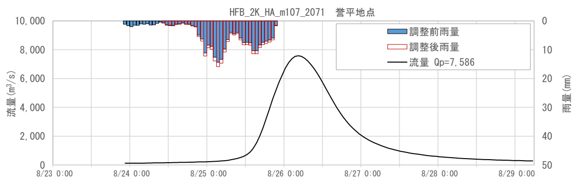
図 1-108 抽出した予測降雨波形のハイドログラフ(誉平地点)
