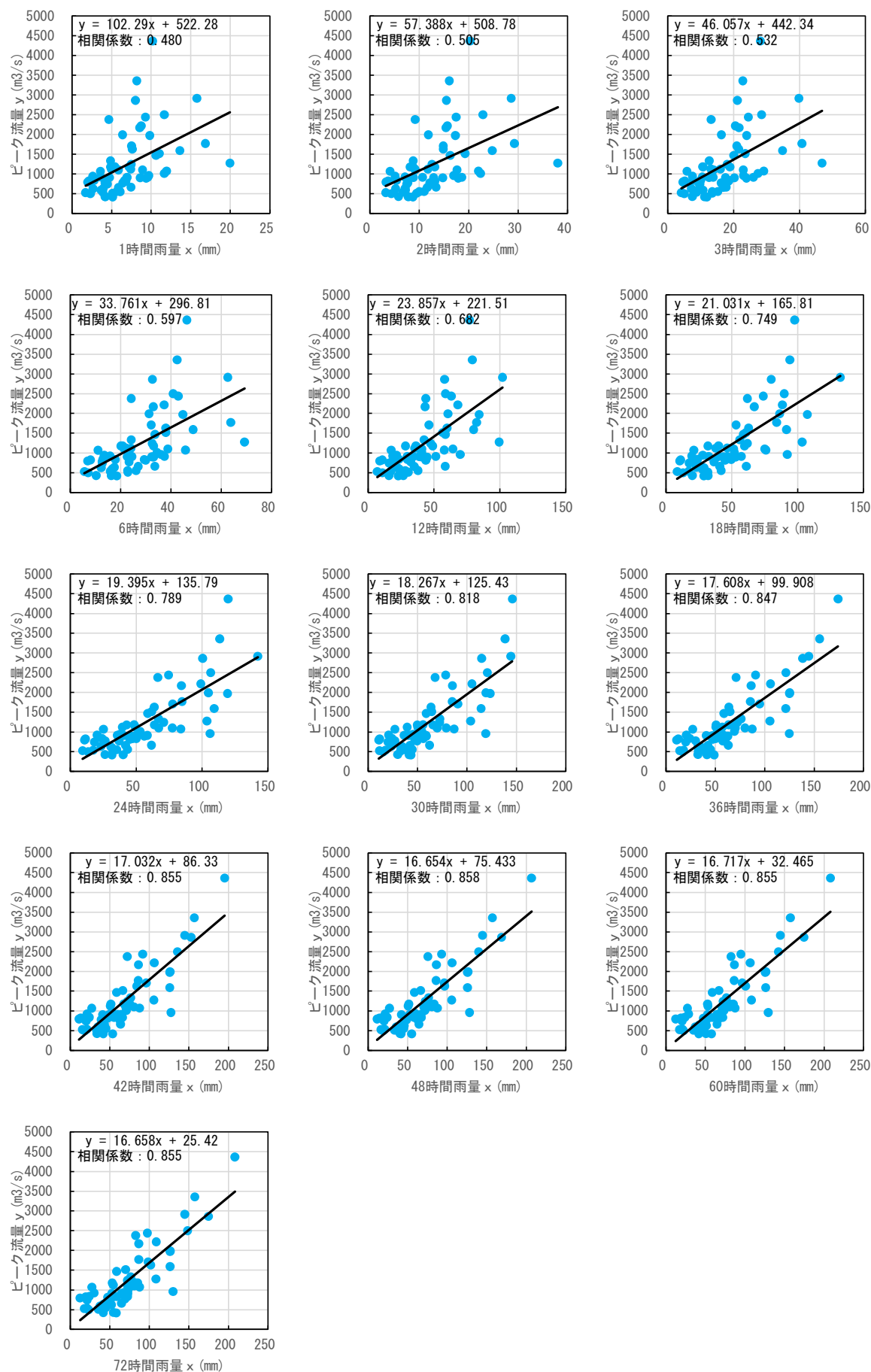
図 1-42 ピーク流量と流域平均時間雨量の相関図【定義①】（誉平地点）
