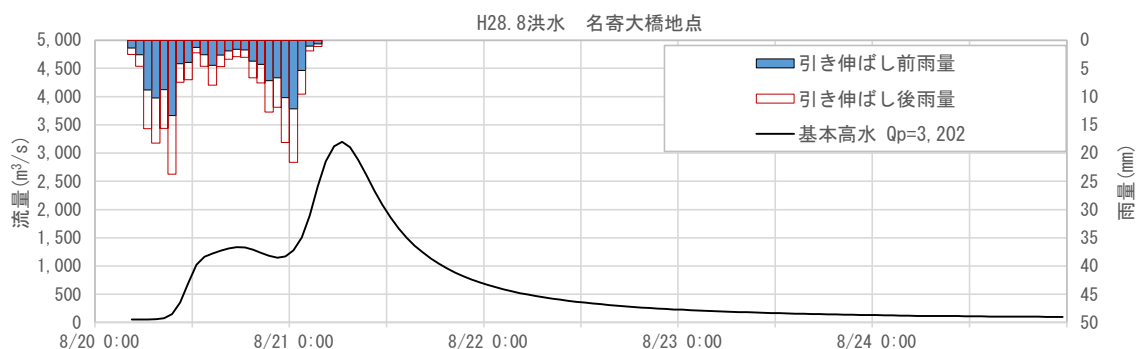
図 1-80 基本高水ハイドログラフ（平成 28 年 8 月洪水 名寄大橋地点）
