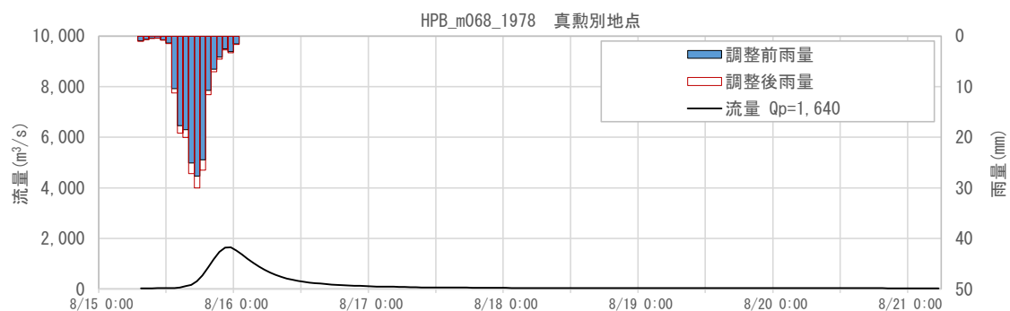
図 1-158 抽出した予測降雨波形のハイドログラフ(真敷別地点)
