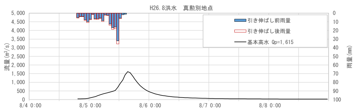
図 1-94 基本高水ハイドログラフ (平成 26 年 8 月洪水 真勲別地点)
