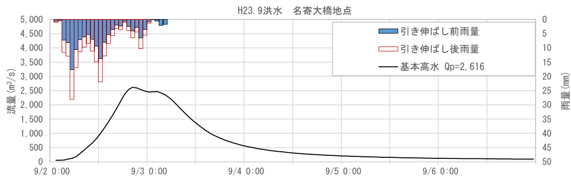
図 1-77 基本高水ハイドログラフ（平成 23 年 9 月洪水 名寄大橋地点）
