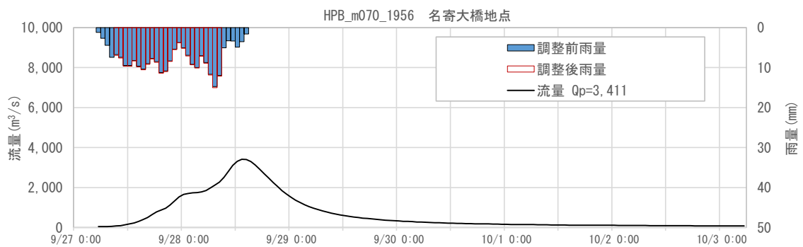
図 1-132 抽出した予測降雨波形のハイドログラフ(名寄大橋地点)
