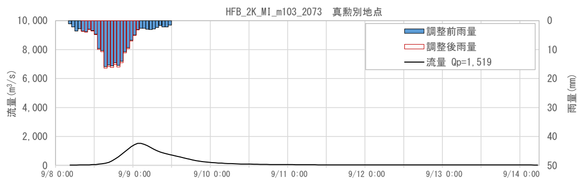
図 1-142 抽出した予測降雨波形のハイドログラフ(真勲別地点)
