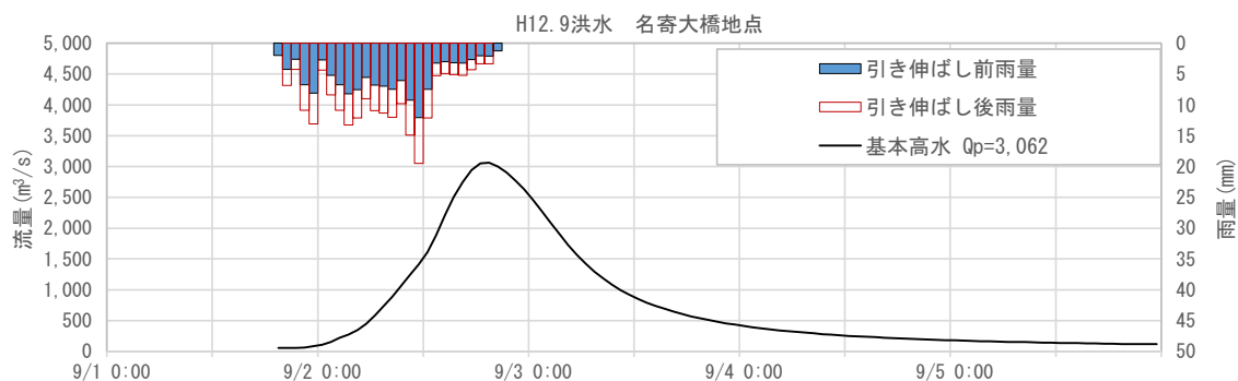
図 1-75 基本高水ハイドログラフ（平成 12 年 9 月洪水 名寄大橋地点）
