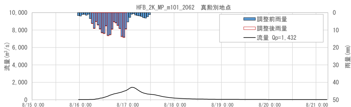
図 1-140 抽出した予測降雨波形のハイドログラフ(真勲別地点)
