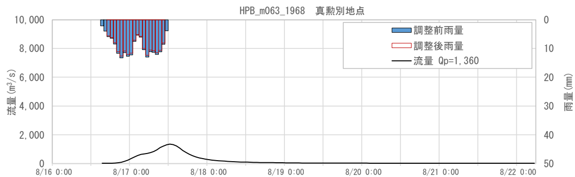
図 1-155 抽出した予測降雨波形のハイドログラフ(真敷別地点)
