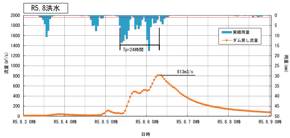
図 1-38 Kinematic Wave 法による洪水到達時間(真熟別地点)
