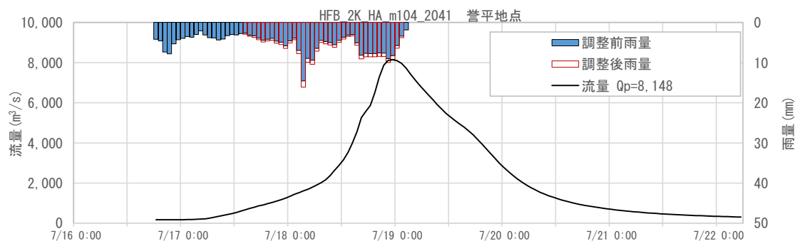
図 1-109 抽出した予測降雨波形のハイドログラフ(誉平地点)
