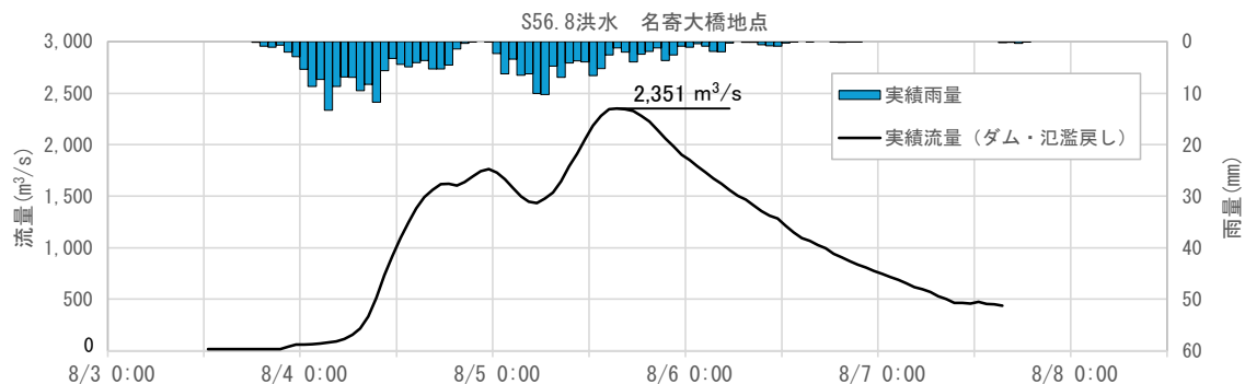
図 1-166 昭和 56 年 8 月洪水の推定結果(名寄大橋地点)
