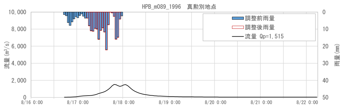
図 1-153 抽出した予測降雨波形のハイドログラフ(真熟別地点)
