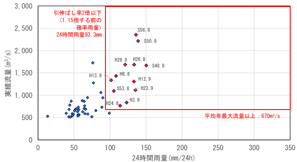
図 1-55 対象洪水の選定結果(名寄大橋地点)
