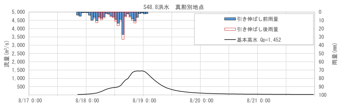
図 1-82 基本高水ハイドログラフ（昭和 48 年 8 月洪水 真勲別地点）
