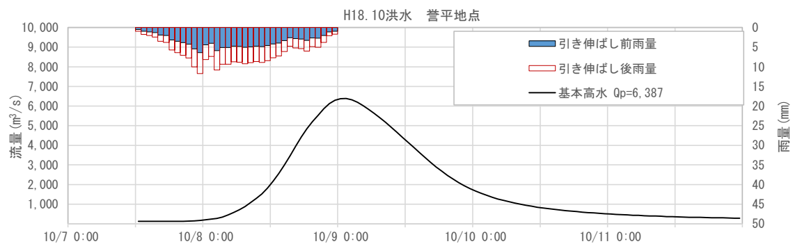
図 1-64 基本高水ハイドログラフ (平成 18 年 10 月洪水 誉平地点)
