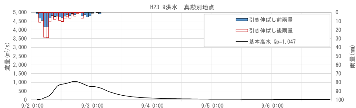
図 1-92 基本高水ハイドログラフ（平成 23 年 9 月洪水 真勲別地点）
