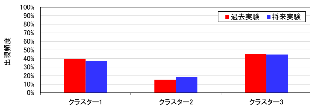
図 1-162 名寄大橋地点における将来実験アンサンブル予測降雨の出現頻度(クラスターごと)
