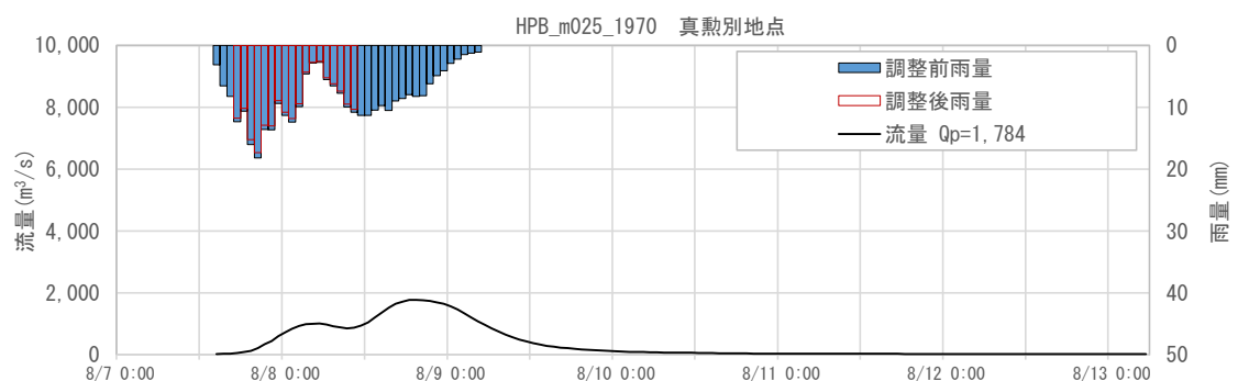
図 1-156 抽出した予測降雨波形のハイドログラフ(真敷別地点)
