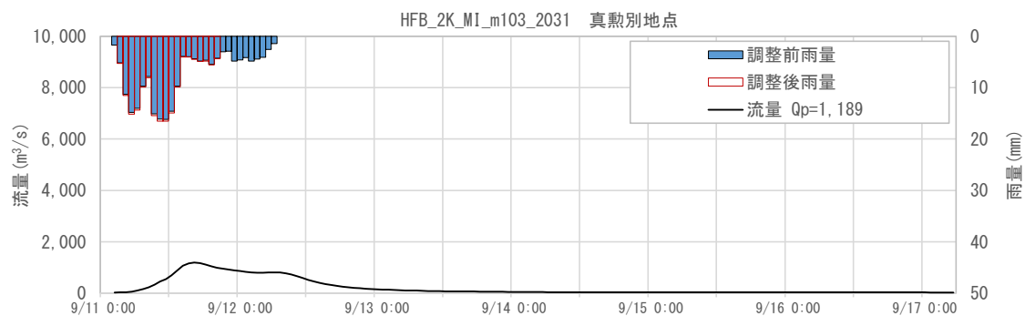
図 1-141 抽出した予測降雨波形のハイドログラフ(真勲別地点)
