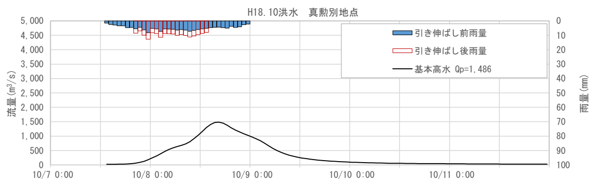
図 1-90 基本高水ハイドログラフ（平成 18 年 10 月洪水 真勲別地点）
