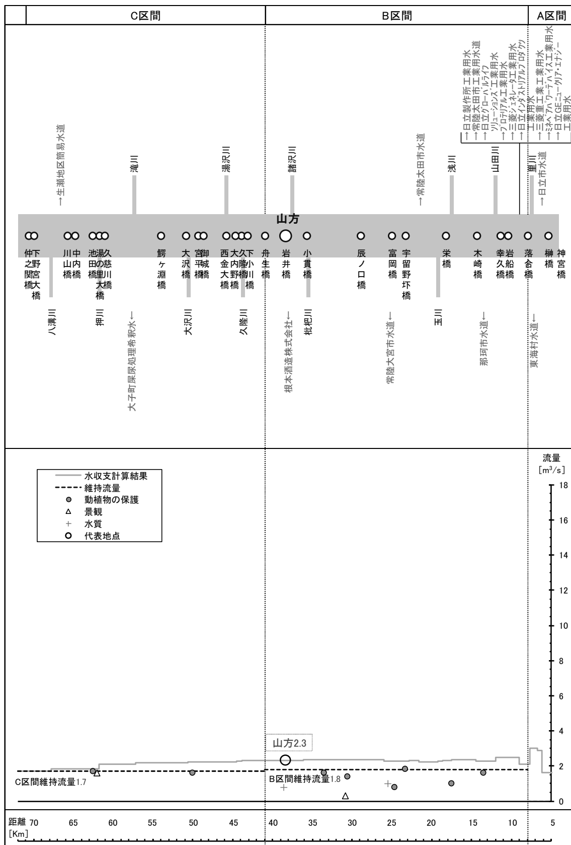
図 6-1(2) 久慈川 正常流量縦断図 (非かんがい期:9/11~3/31)
