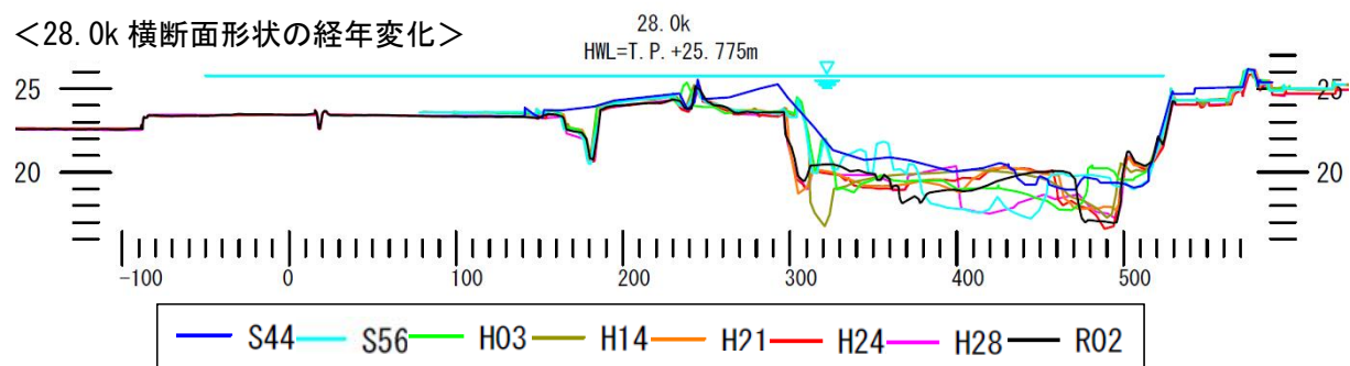
図 4-7 28.0k断面の横断形状(動的平衡状況)
