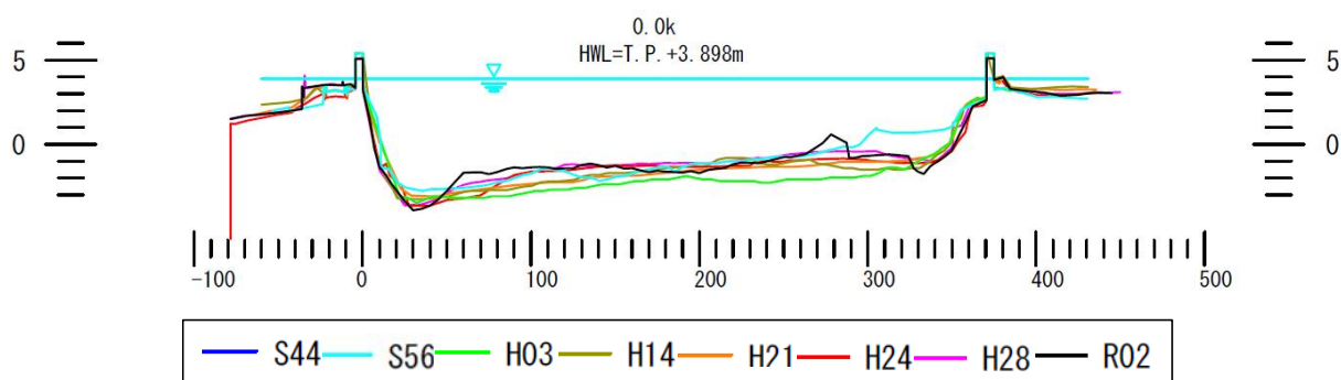
図 5-3 河口部の経年変化横断図
