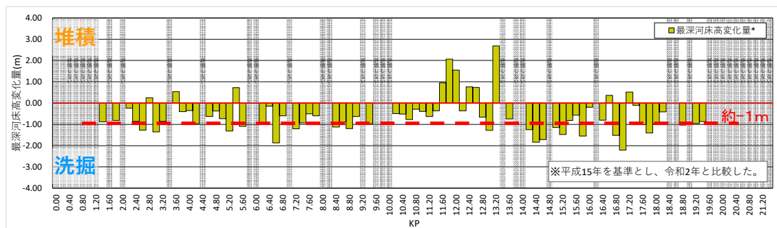
図 2-13 最深河床高比較図（18 年間（平成 15 年から令和 2 年）の変化）
