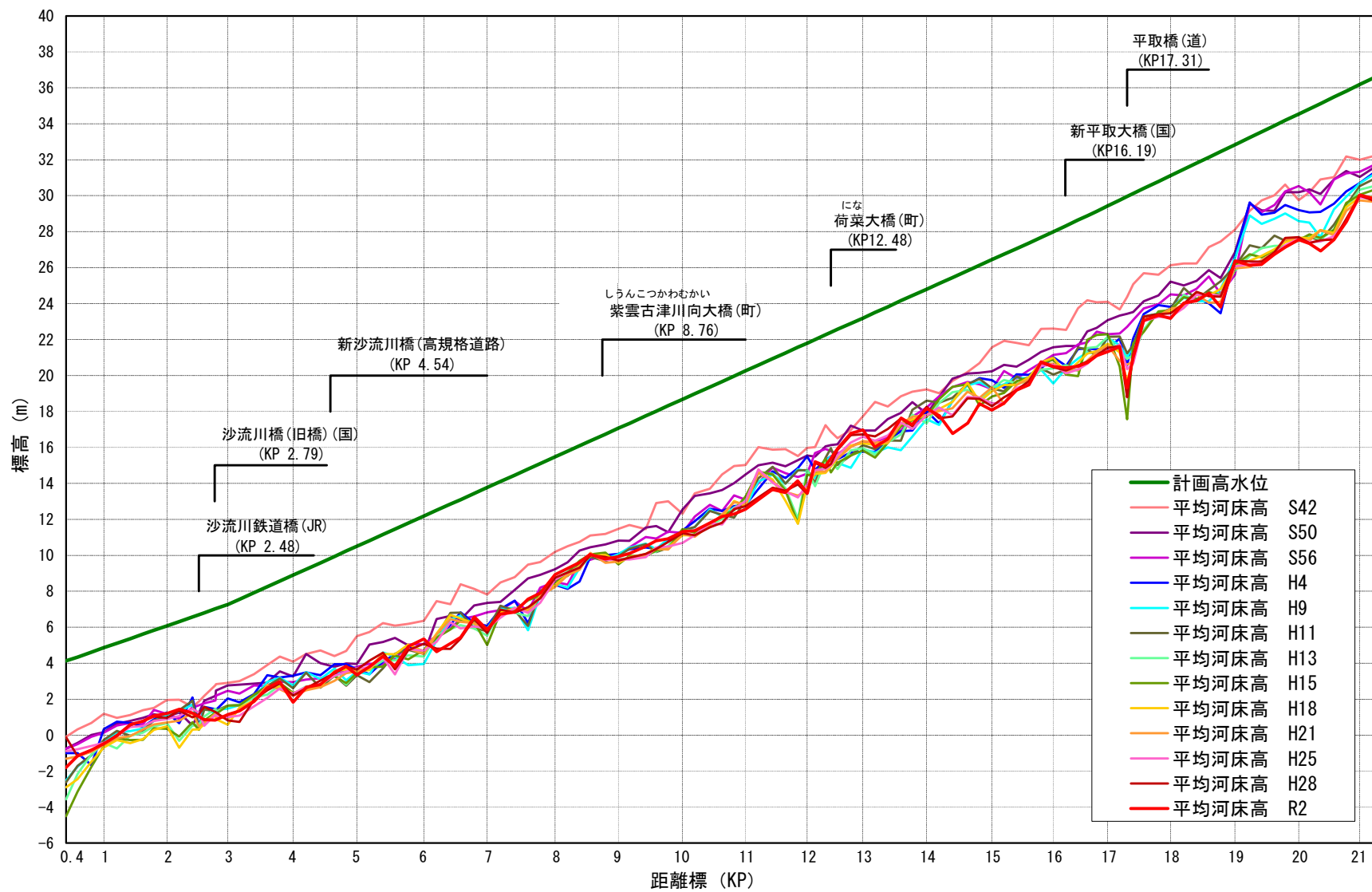
図 2-9 二風谷ダム下流区間の平均河床高経年変化縦断図
