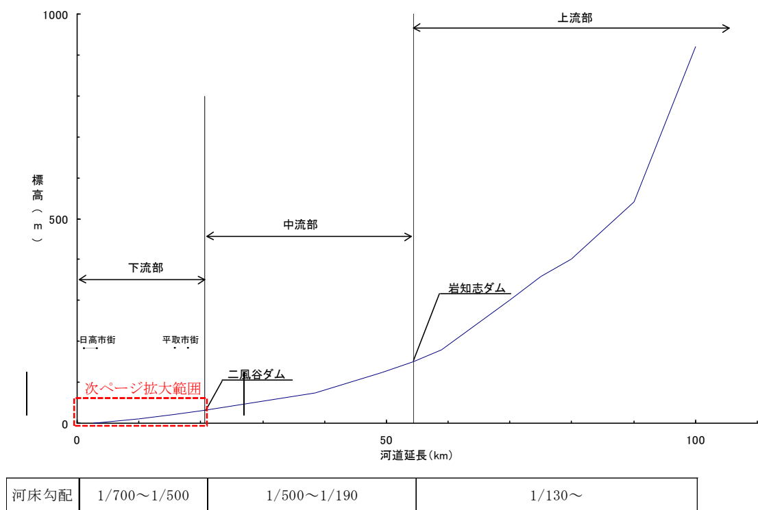
図 2-8 沙流川河床高縦断図
