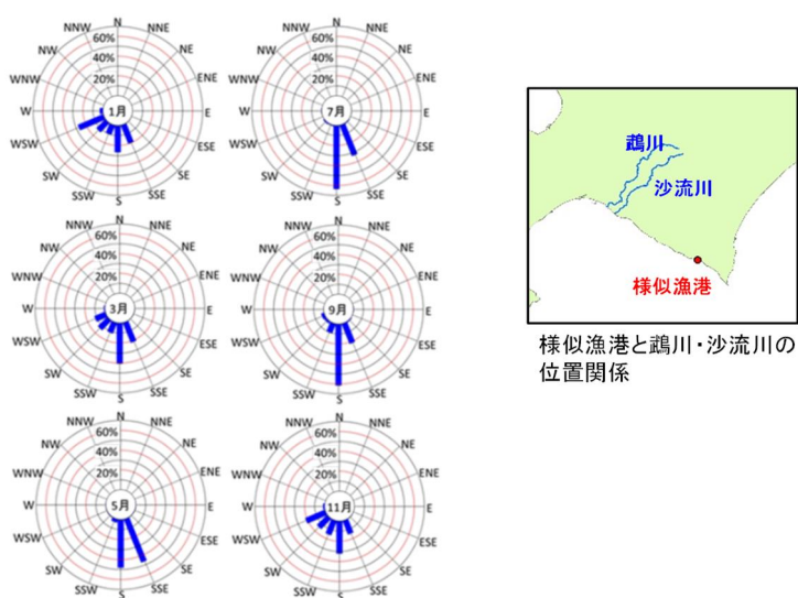
図 2-23 様似漁港沖における波向別の波浪エネルギーフラックスの割合
