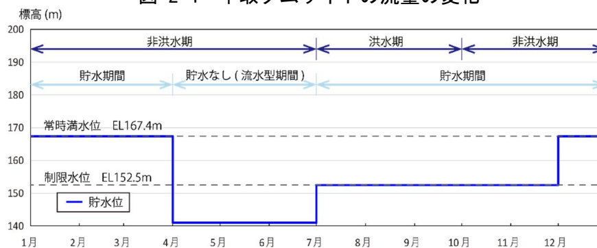
図 2-5 平取ダムの運用
