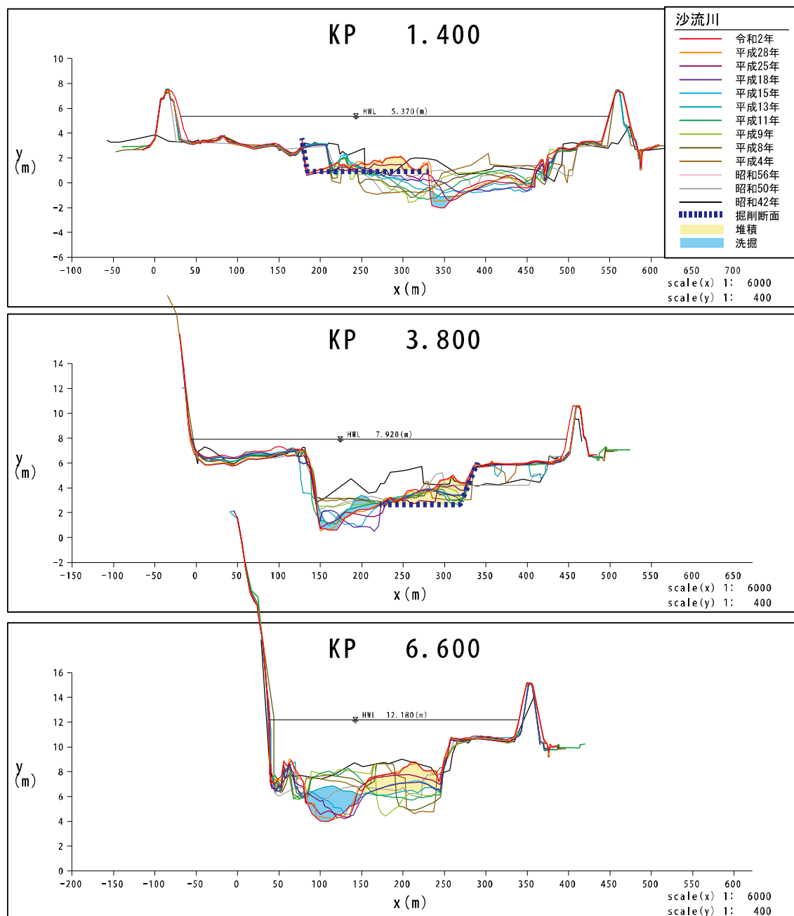
図 2-11 経年変化横断面図 (KP1.4~KP6.6)
