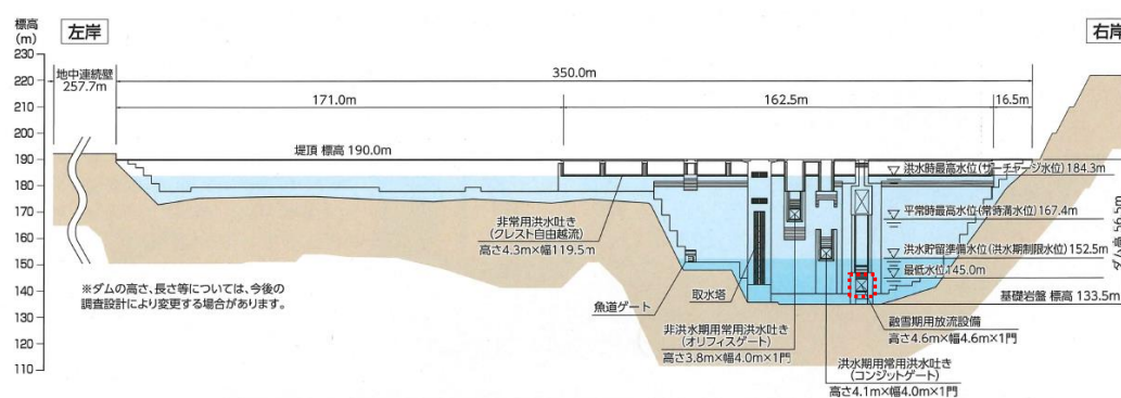
図 2-3 平取ダム上流面図
