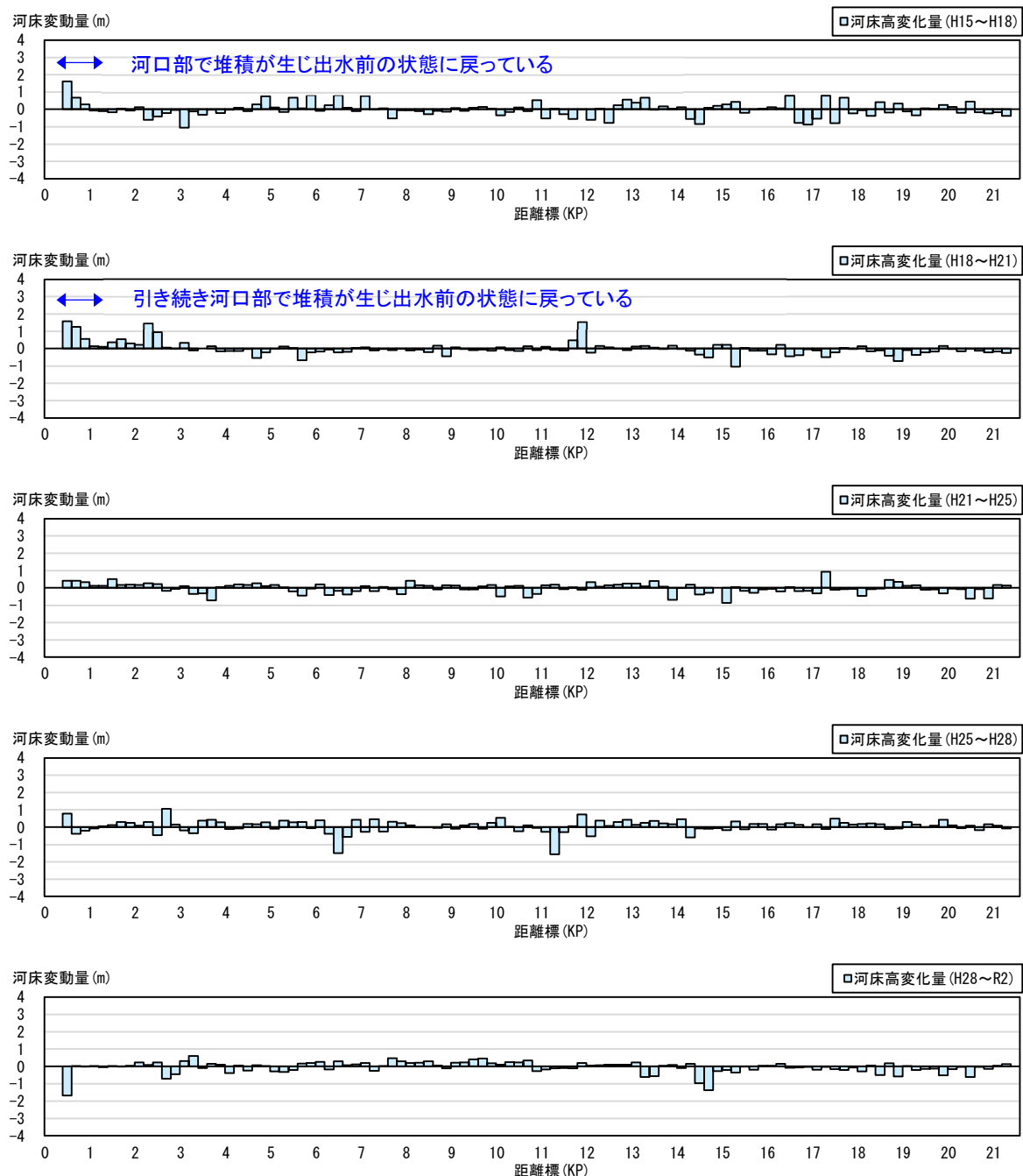
図 2-10 平均河床高の変化 (2)
