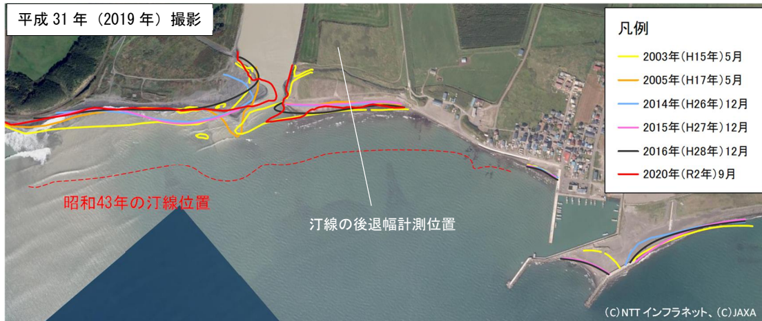
写真 2-13 河口部汀線測量
