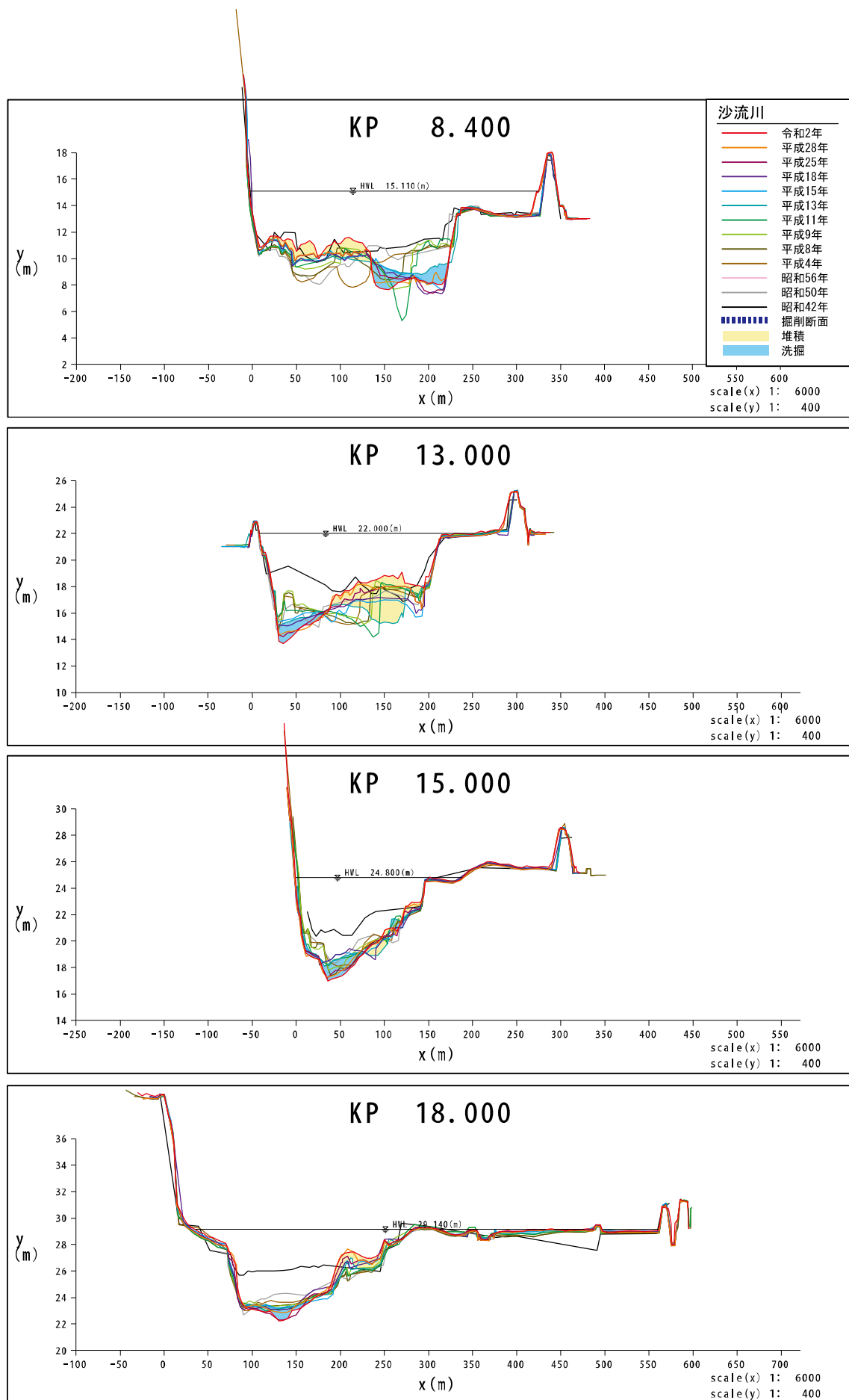
図 2-11 経年変化横断面図 (KP8.4~KP18.0)
