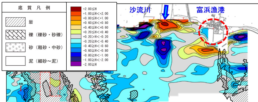
図 2-22 海底の高さの変化（平成 16 年→令和 3 年）
