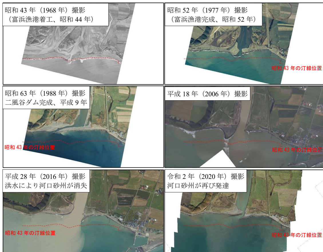
写真 2-14 河口部付近の汀線変化
