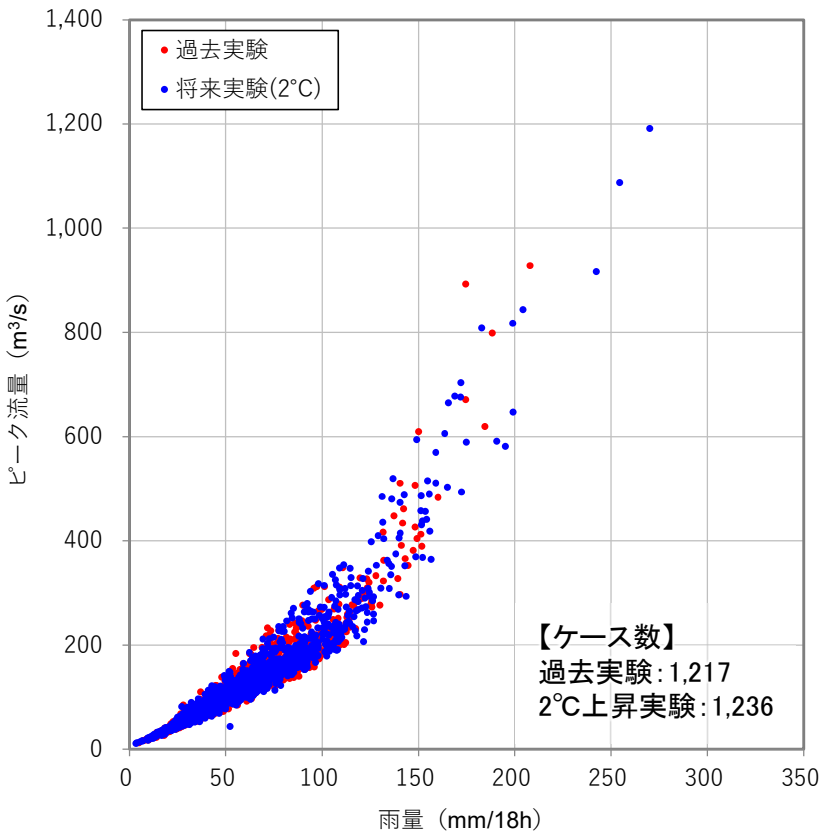
問寒別川(下問寒別) アンサンブル予測降雨 RQ図
