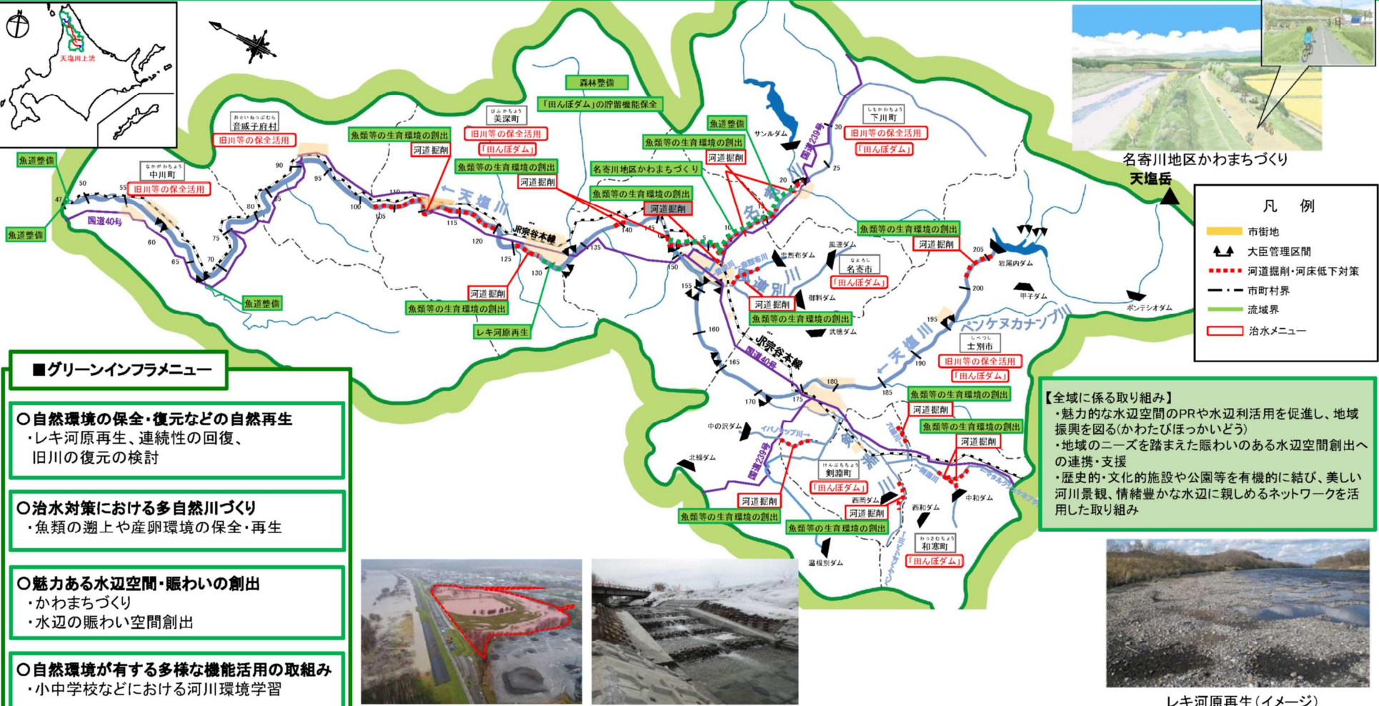
旧川等の保全活用 (士別市、下川町、美深町、音威子府村、中川町) 魚類の遡上や産卵環境の保全・再生 (中川町、下川町) レキ河原再生(イメージ) ※具体的な対策内容については、今後の調査・検討等により変更となる場合がある。
