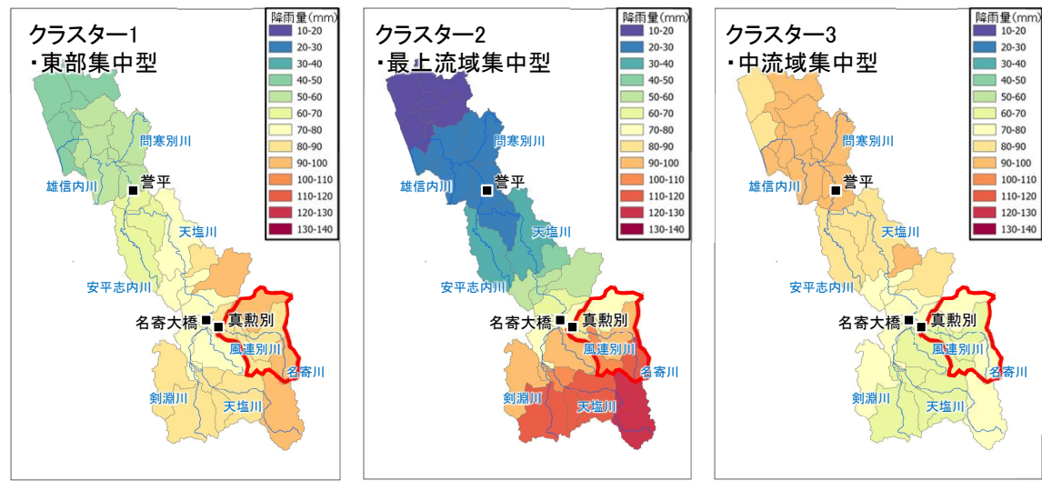
アンサンブル予測雨量による降雨分布のクラスター分析結果
