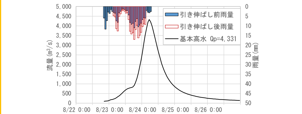
名寄大橋地点 昭和50年8月洪水波形
