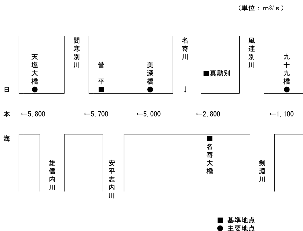
図一2 天塩川計画高水流量図
