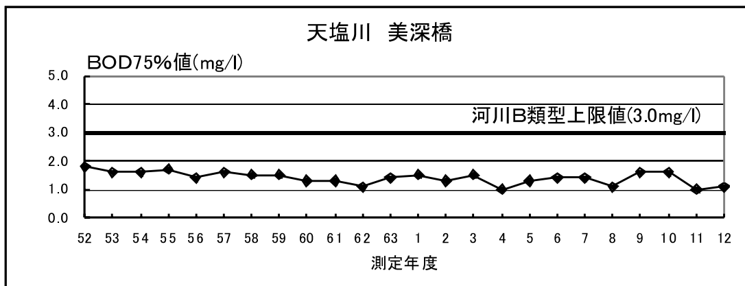
図－５（７） 美深橋地点における水質（ＢＯＤ75%値）の経年変化
