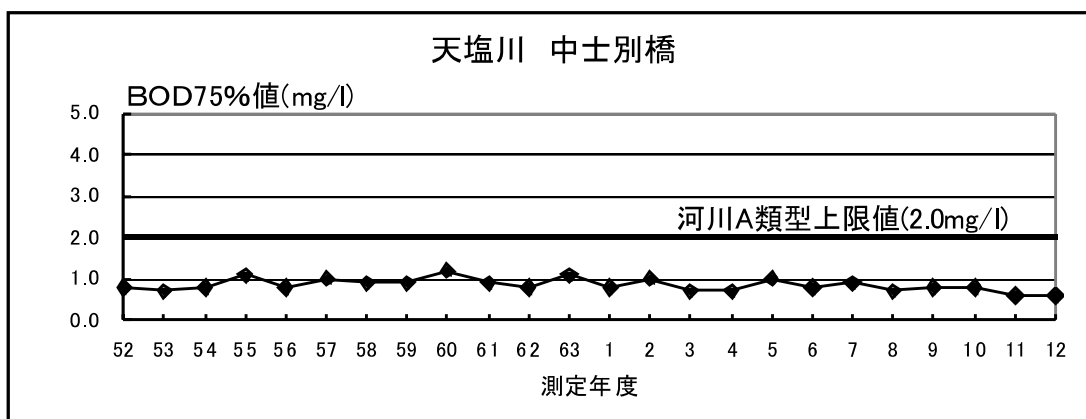
図－５（２） 中士別橋地点における水質（ＢＯＤ75%値）の経年変化
