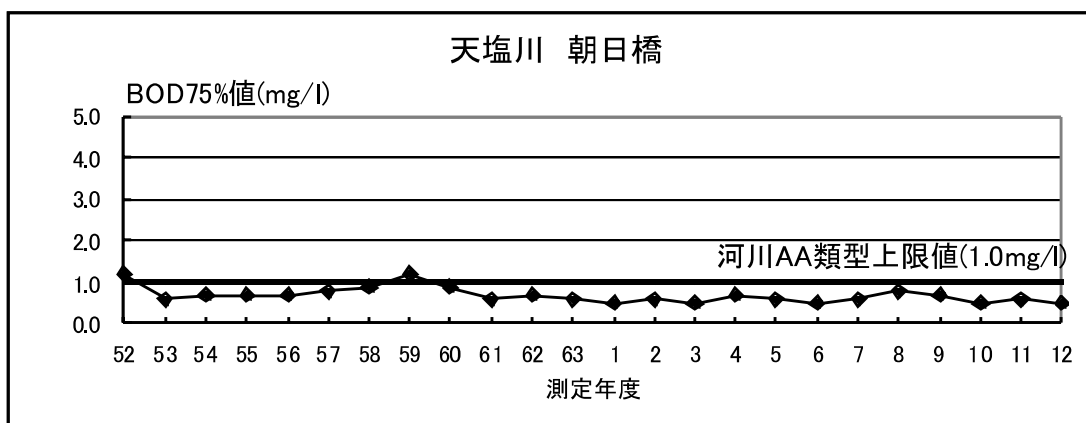
図－５（１） 朝日橋地点における水質（ＢＯＤ75%値）の経年変化
