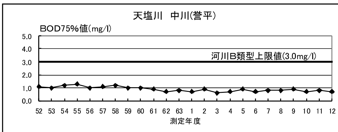
図－５（６） 中川（誉平）地点における水質（ＢＯＤ75%値）の経年変化
