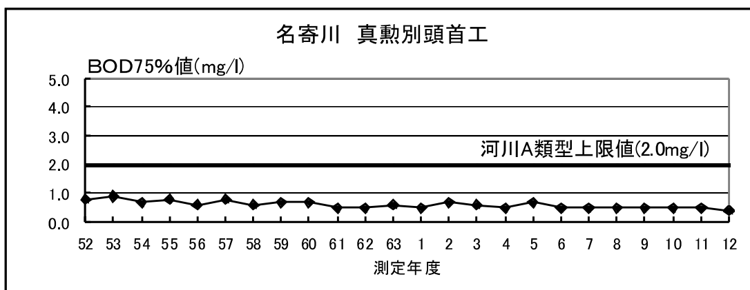
図－５（３） 真熟別頭首工地点における水質（ＢＯＤ75%値）の経年変化
