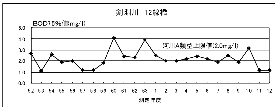
図－５（５） 剣淵川 12線橋における水質（ＢＯＤ75%値）の経年変化
