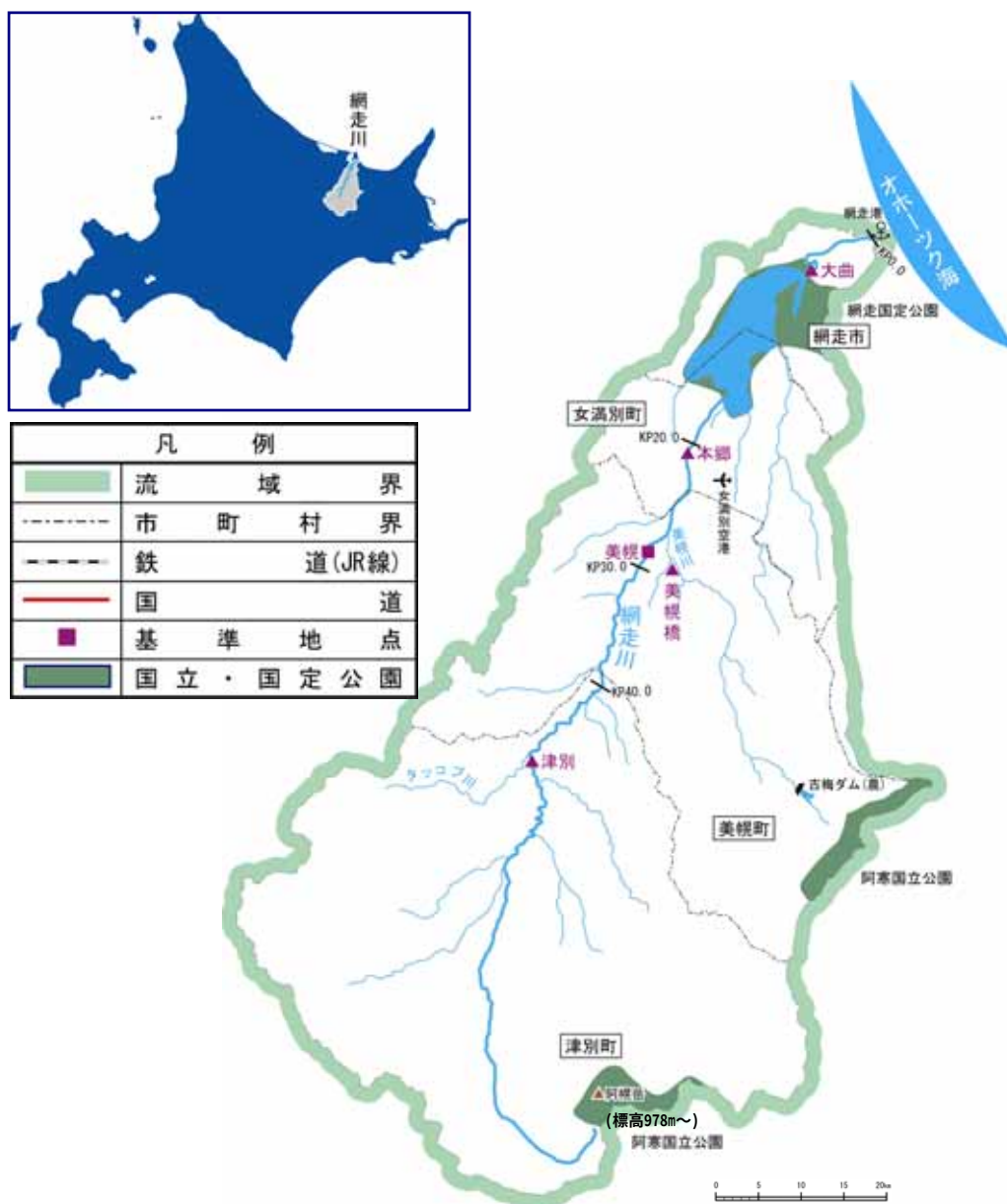
図 1-1 網走川水系図
