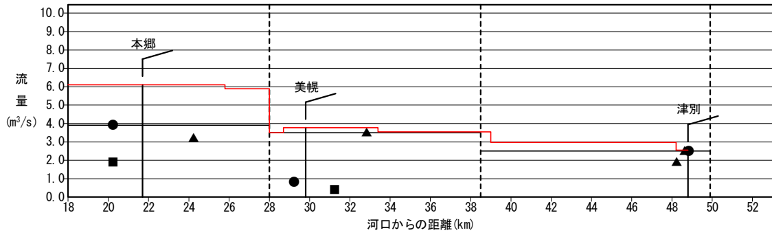
図 6.1 網走川 水収支縦断図(かんがい期、非かんがい期)
