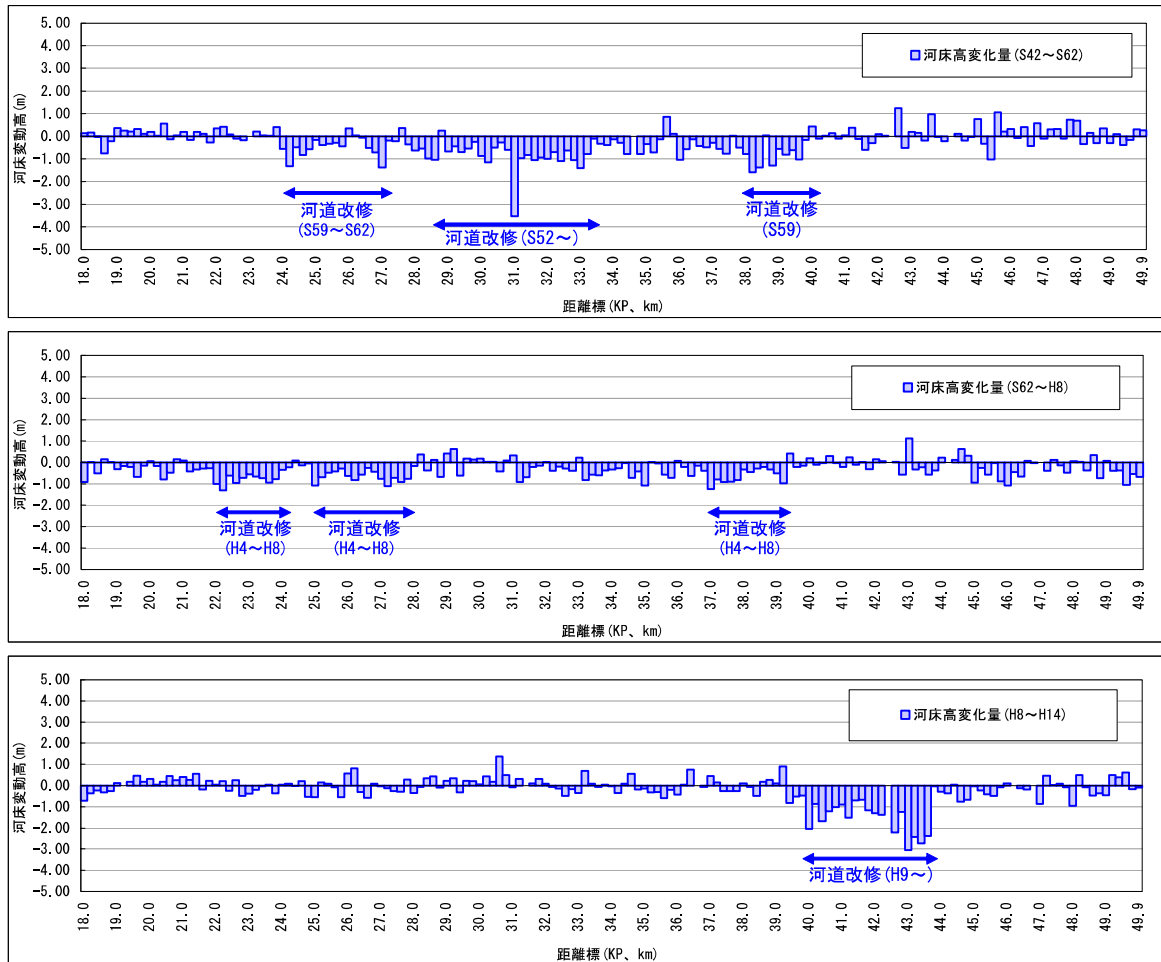
図 2-6 河床変動高経年変化縦断面図
