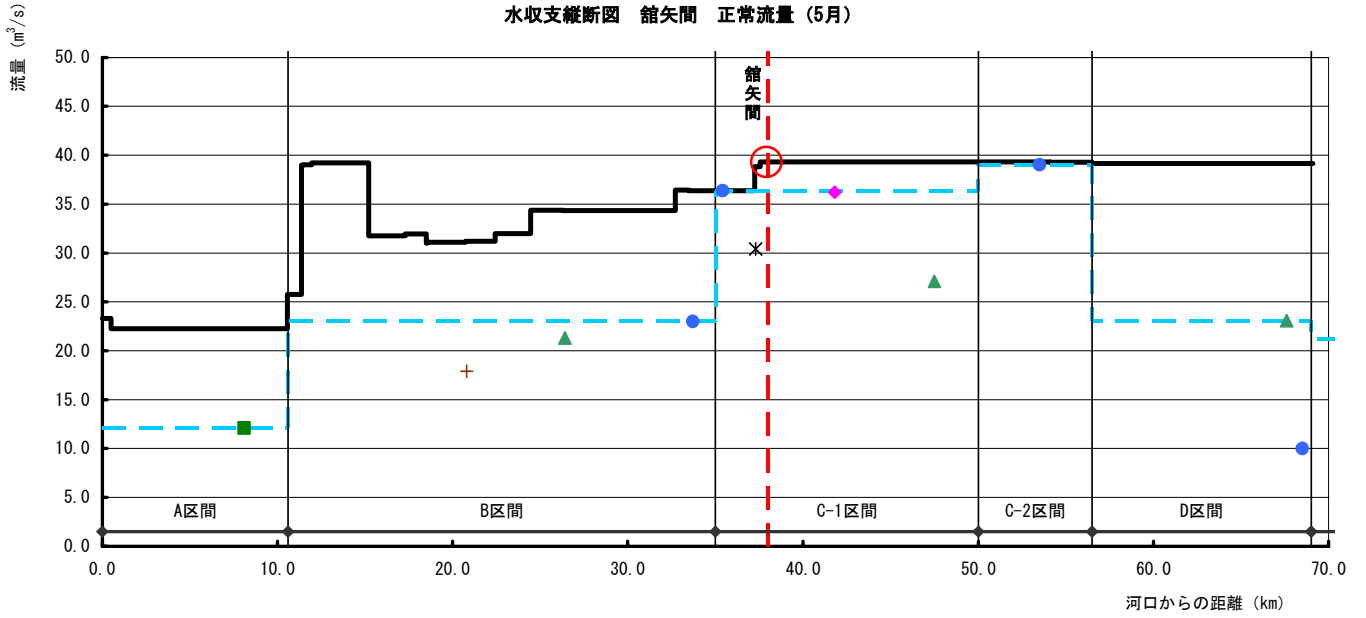
水収支縦断面図 館矢間 正常流量 (6月)
