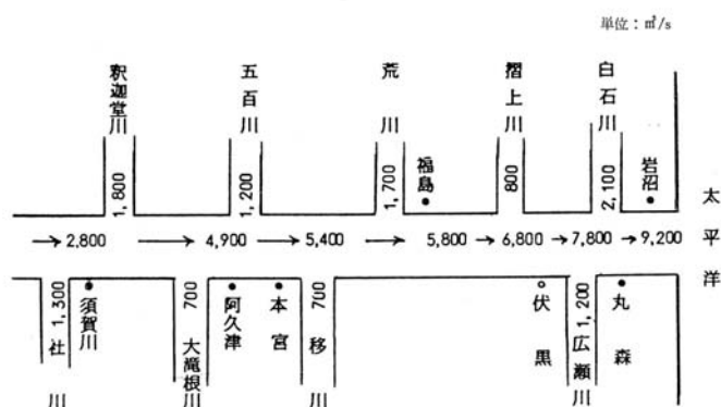
図 4-2-3 現行計画の計画高水流量
