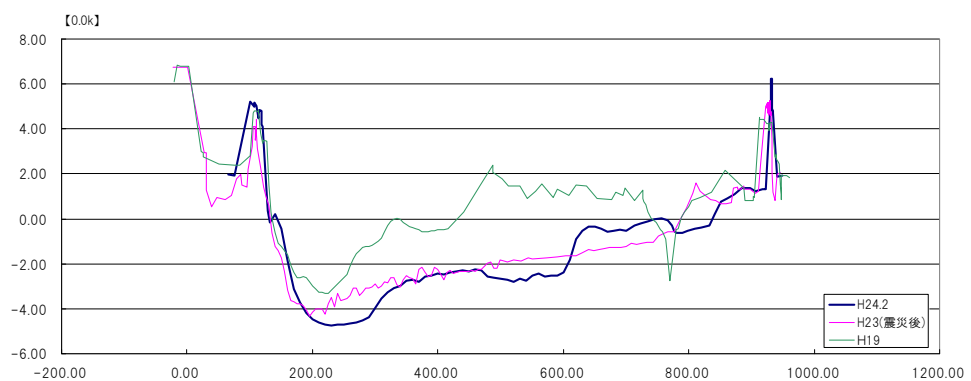
図 8-2-3 阿武隈川河口部の横断図
