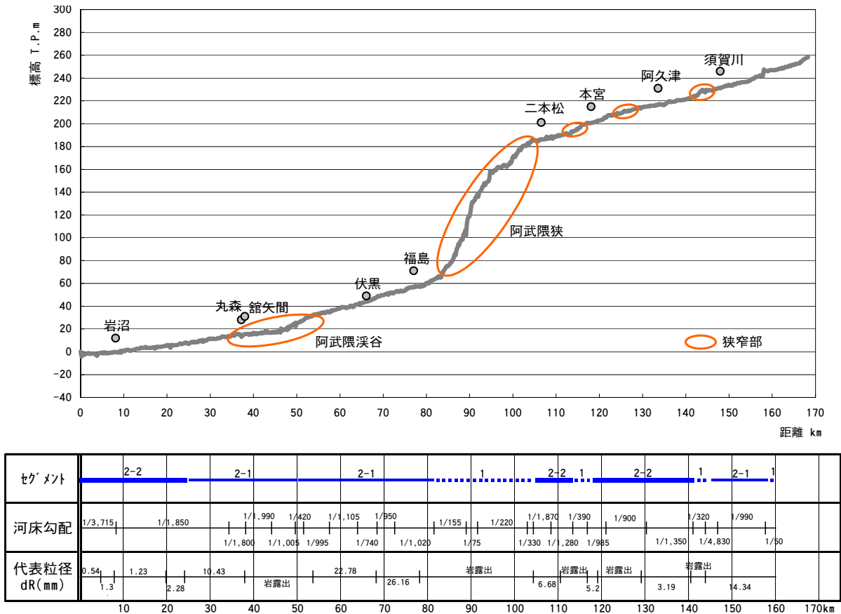
図 8-1-1 阿武隈川における平均河床高縦断図と河道特性図
