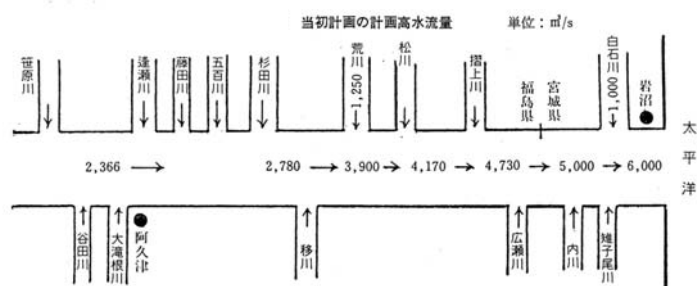
図 4-2-1 当初計画の計画高水流量
