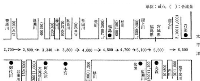
図 4-2-2 第二次改訂計画の計画高水流量
