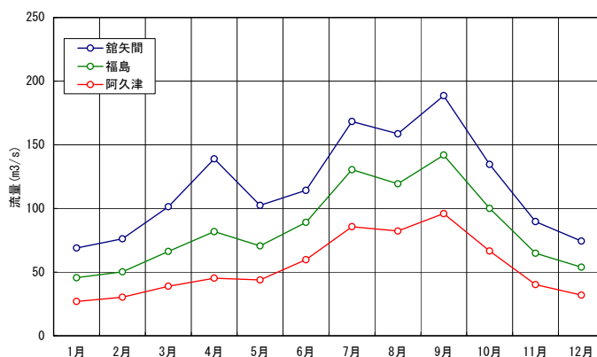
図 6-1-2 主要観測所地点の月別平均流量(S38~H22, 48 ヲ年)
