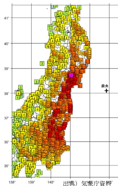
図 4-3-1 震度分布図
