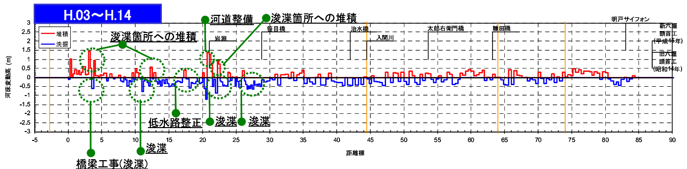
図 2-2 荒川平均河床高変動量
