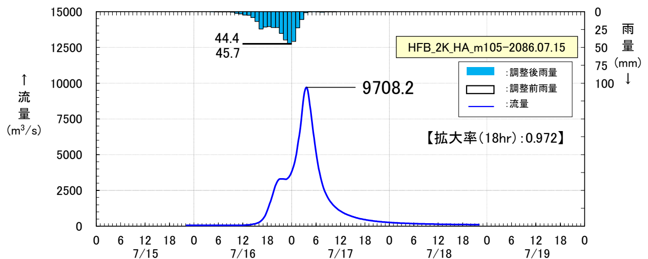
図 1-11-2(1) 抽出した予測降雨波形のハイドログラフ（荒瀬地点）
