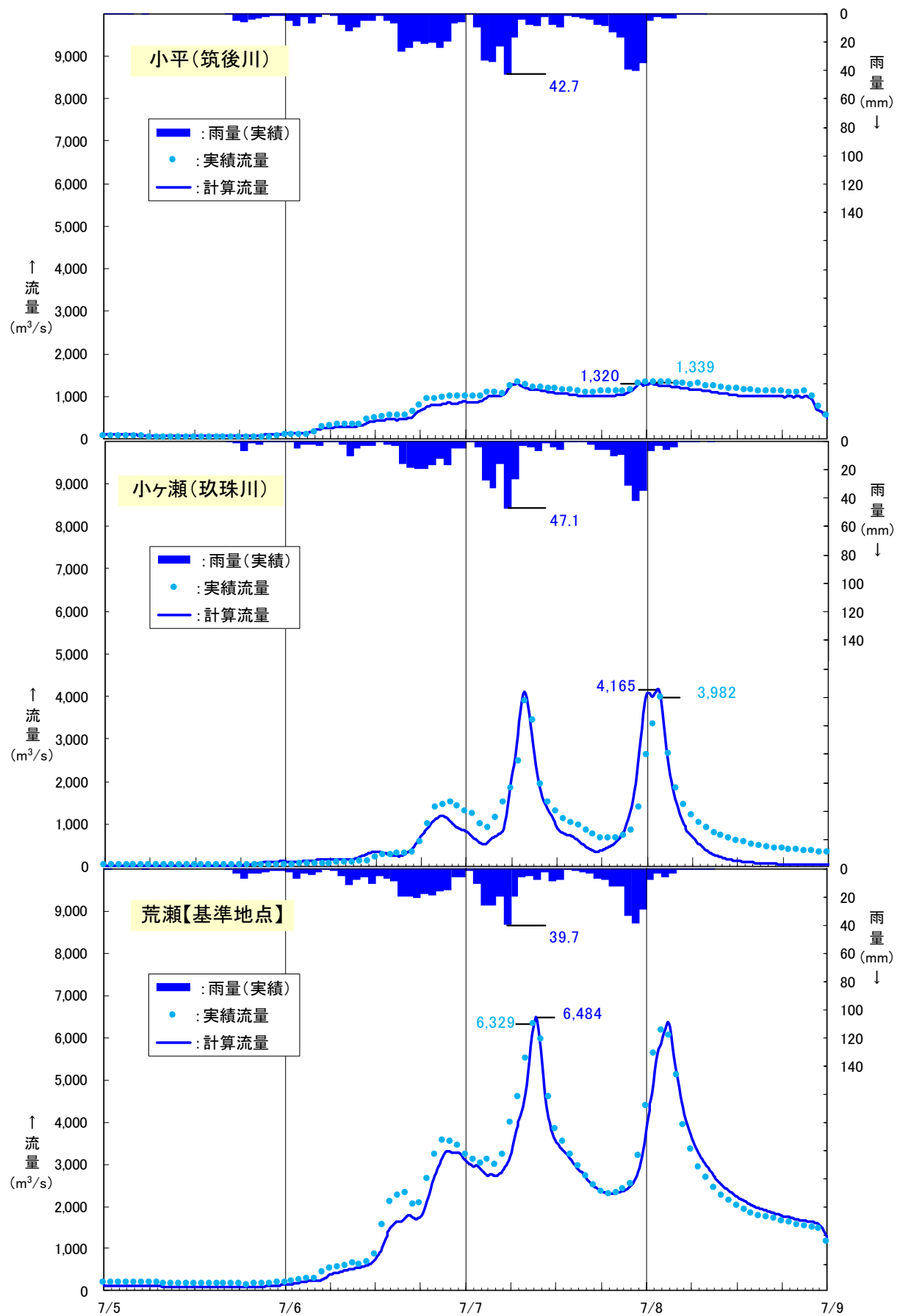
図 1-4-6 令和2年7月洪水再現計算結果
