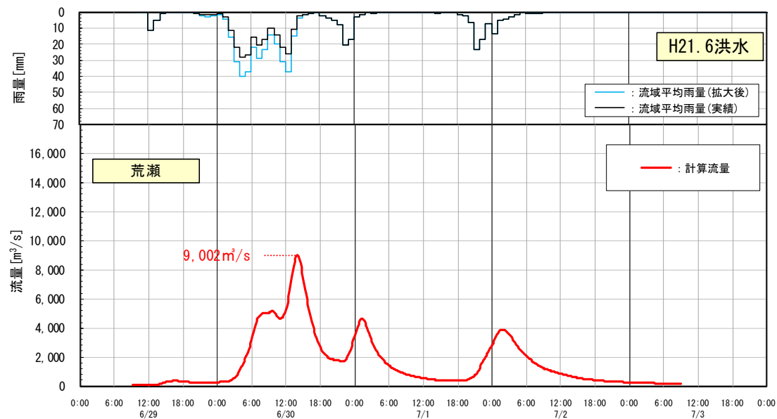
図 1-10-1 (5) 基本高水ハイドログラフ
