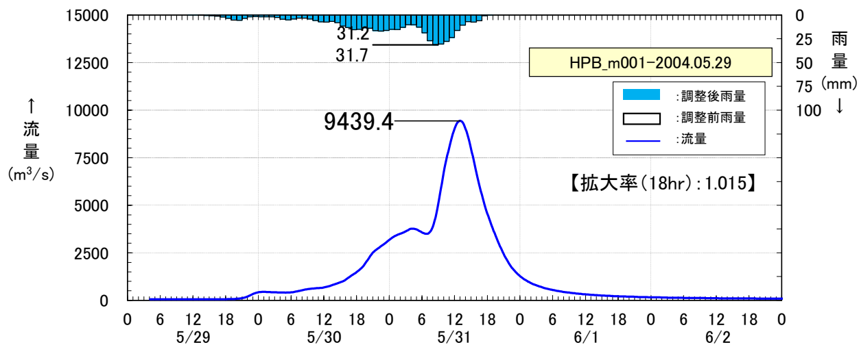
図 1-11-2 (3) 抽出した予測降雨波形のハイドログラフ (荒瀬地点)
