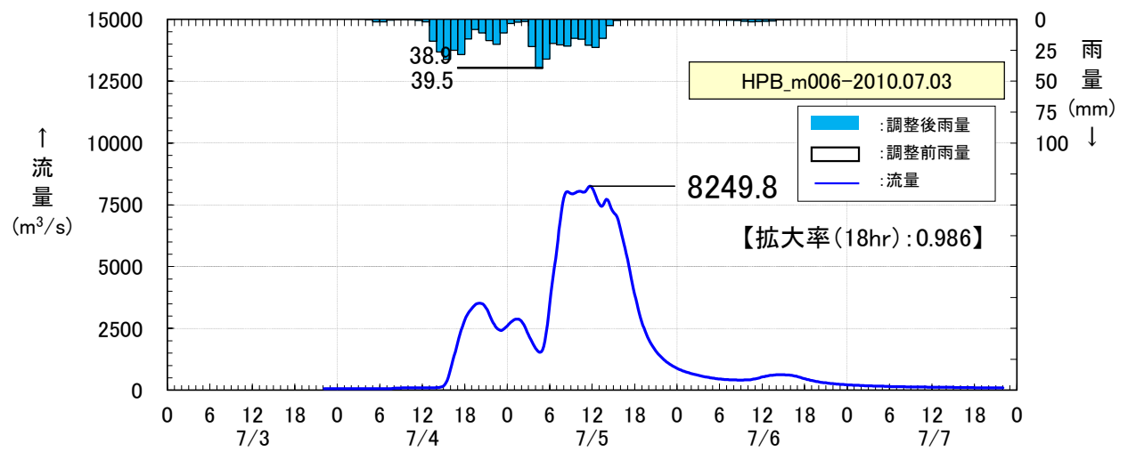
図 1-11-2 (4) 抽出した予測降雨波形のハイドログラフ (荒瀬地点)
