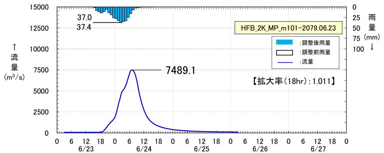
図 1-11-2(2) 抽出した予測降雨波形のハイドログラフ (荒瀬地点)
