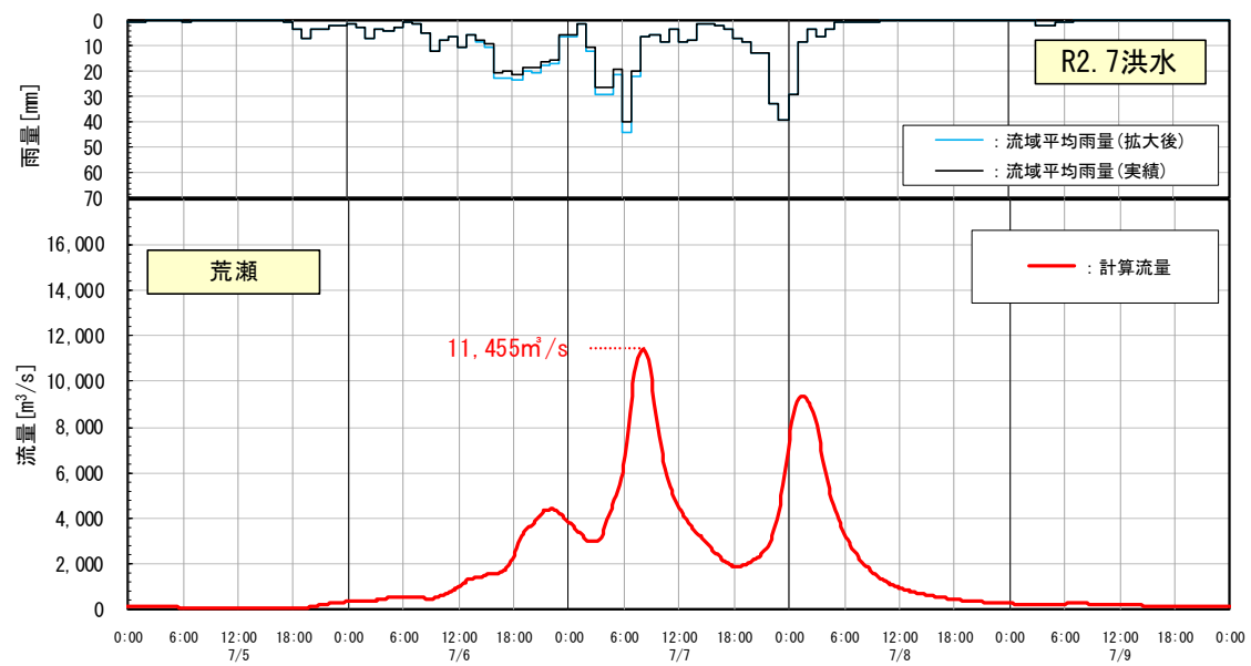
図 1-13-2 基本高水のピーク流量ハイドログラフ（令和2年（2020年）7月洪水）
