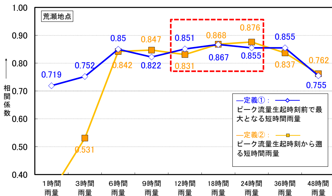
図 1-6-2 ピーク流量と相関の高い短時間雨量
