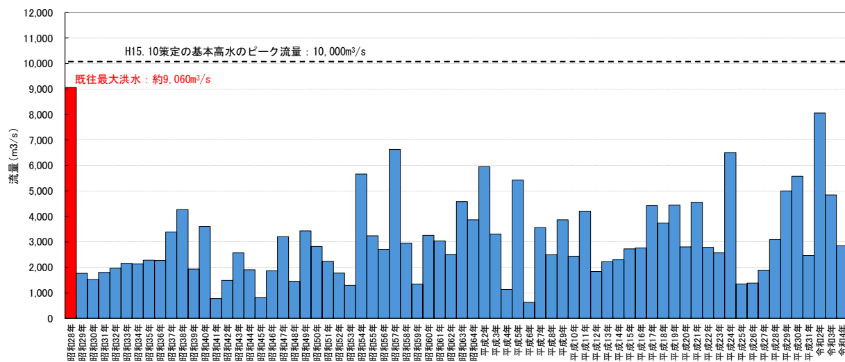
図 1-3-2 年最大流量（基準地点荒瀬）
