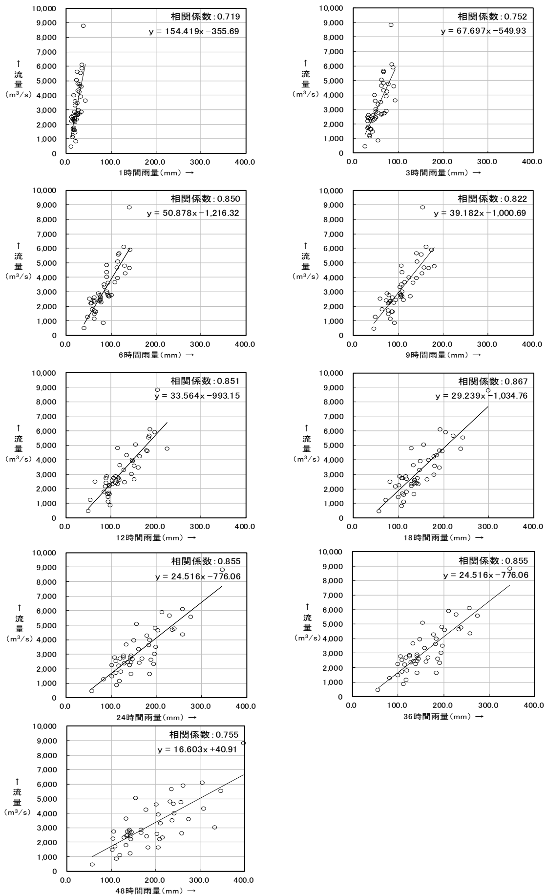
図 1-6-3 ピーク流量と流域平均時間雨量の相関図
