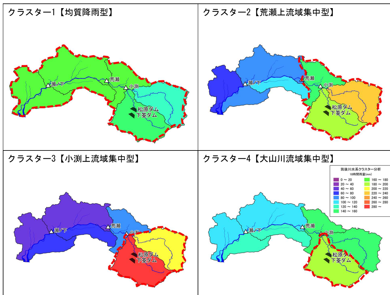
図 1-11-4 筑後川流域における将来実験アンサンブル予測降雨のクラスター分析結果
