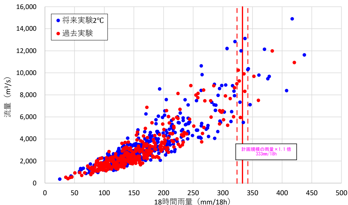
図 1-11-1 アンサンブル予測降雨波形からの抽出（基準地点荒瀬）
