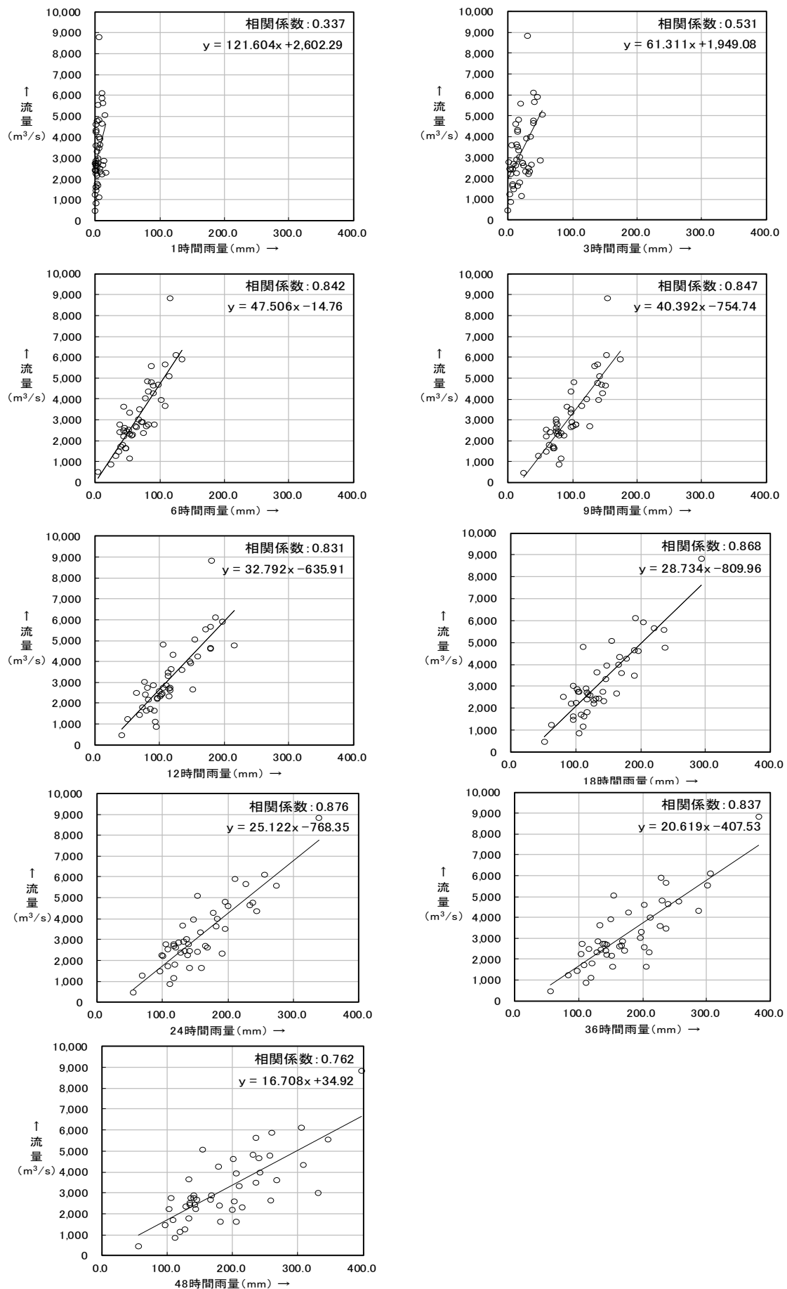
図 1-6-4 ピーク流量と流域平均時間雨量の相関図
