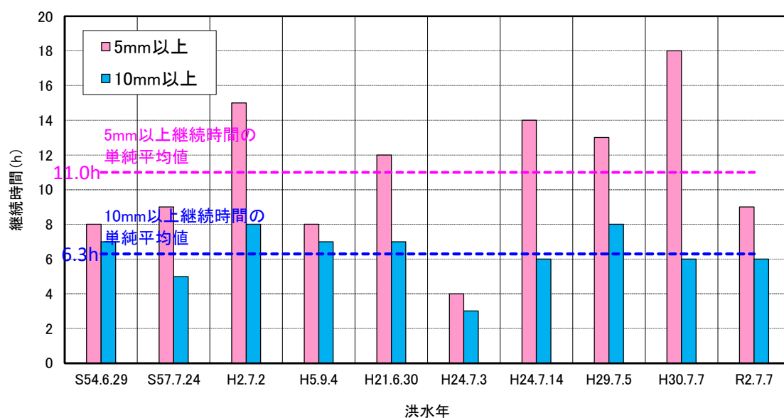
図 1-6-5 強い降雨強度の継続時間（基準地点荒瀬上流域平均雨量）
