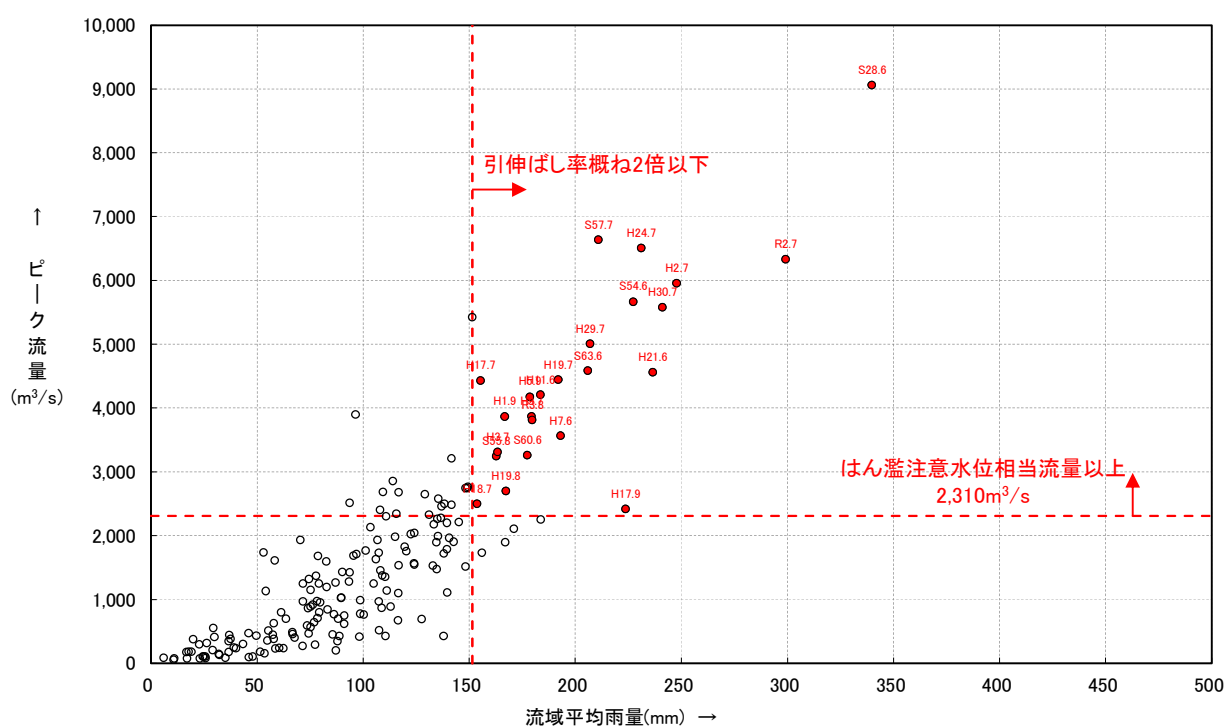
図 1-8-1 対象洪水の選定（基準地点荒瀬）
