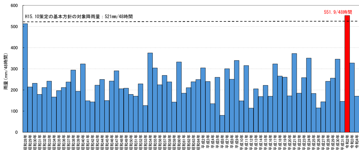
図 1-3-1 年最大降雨量（基準地点荒瀬上流域平均雨量）
