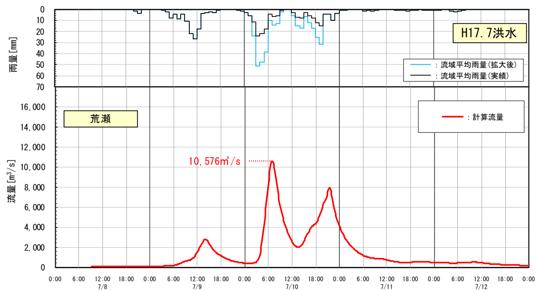
図 1-10-1 (4) 基本高水ハイドログラフ
