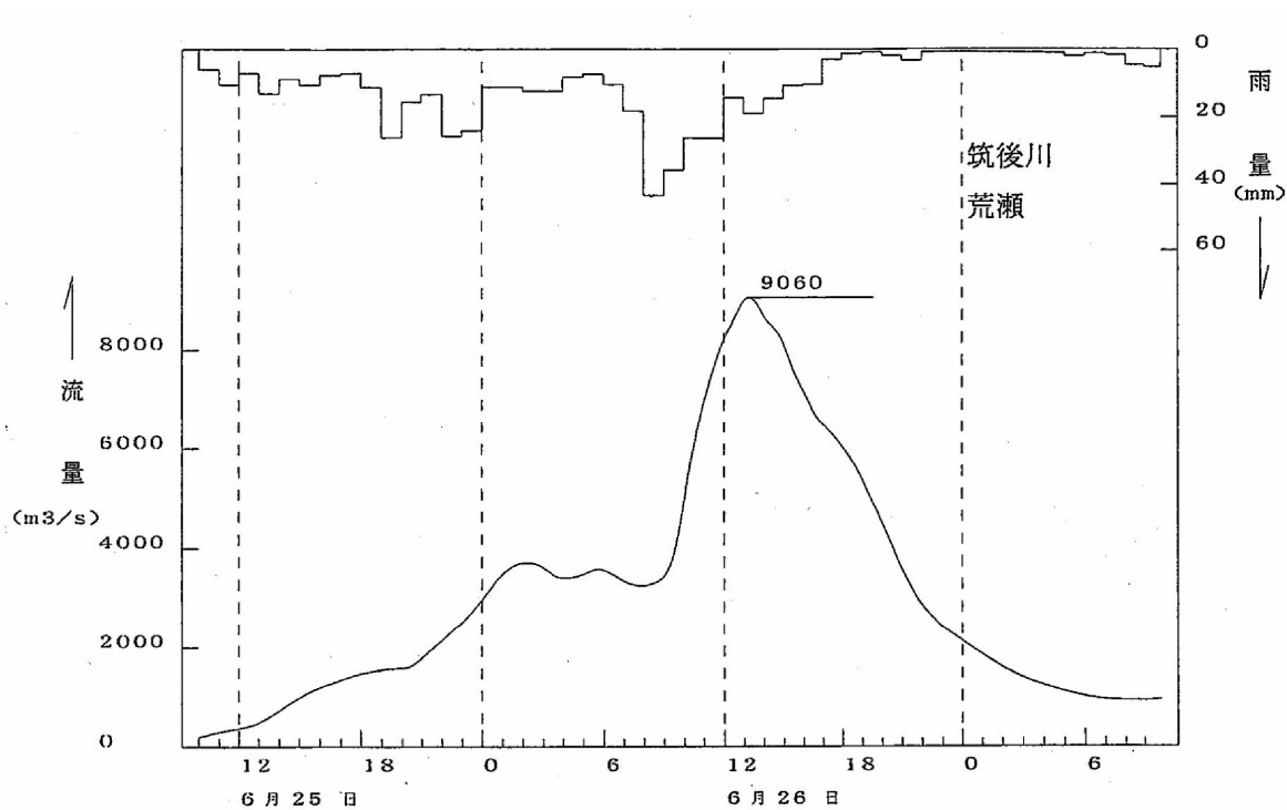
図 1-12-1 昭和28年6月洪水の推定結果（基準地点荒瀬）
