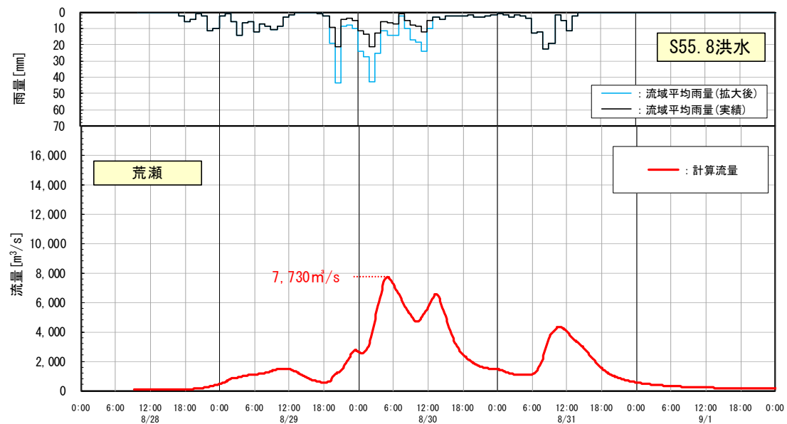
図 1-10-1 (1) 基本高水ハイドログラフ
