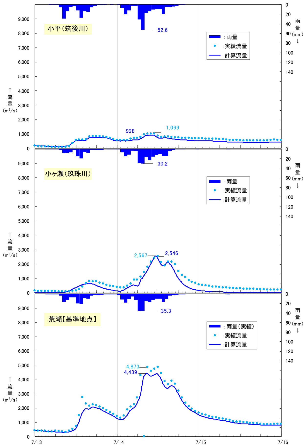
図 1-4-4 平成24年7月洪水再現計算結果
