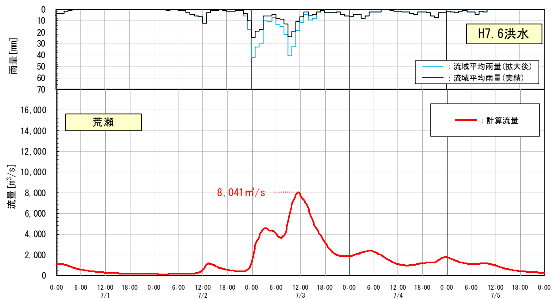
図 1-10-1 (3) 基本高水ハイドログラフ
