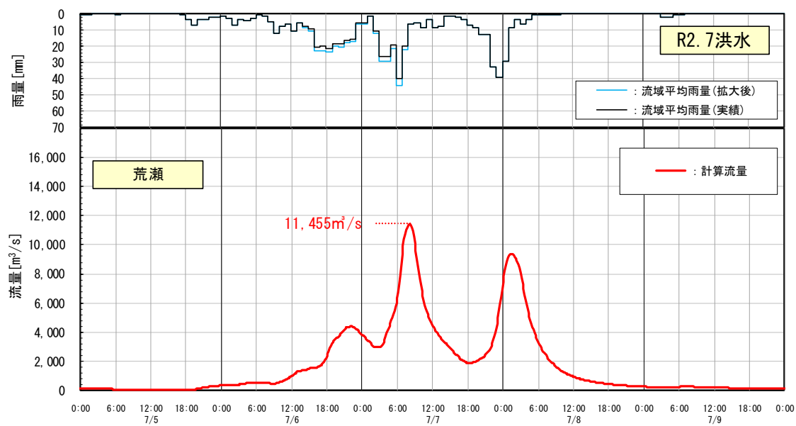
図 1-10-1 (6) 基本高水ハイドログラフ
