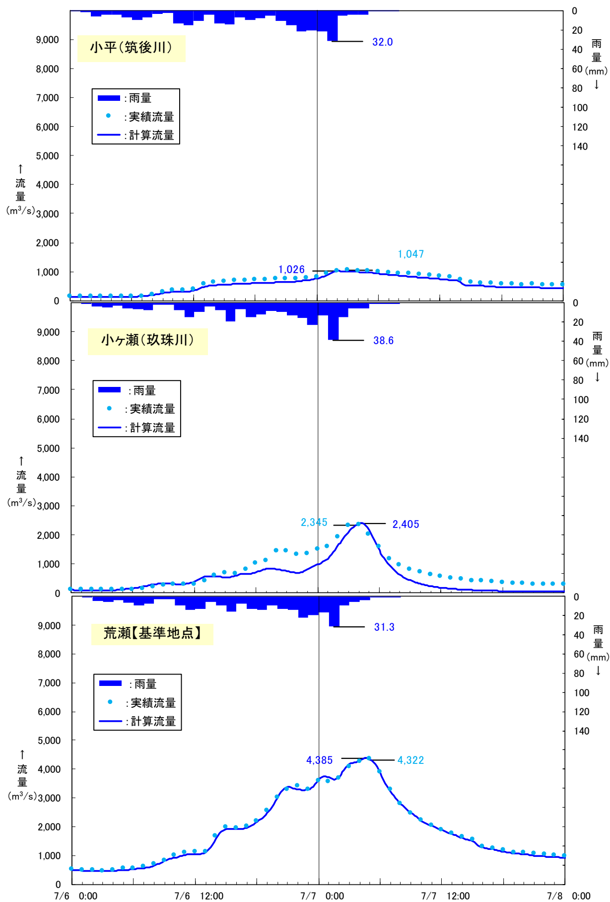
図 1-4-5 平成30年7月洪水再現計算結果
