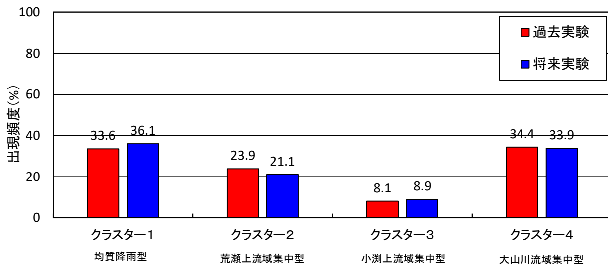
図 1-11-5 筑後川流域におけるアンサンブル予測降雨の出現頻度
