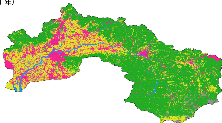
図 1-4-3 土地利用状況の変化
