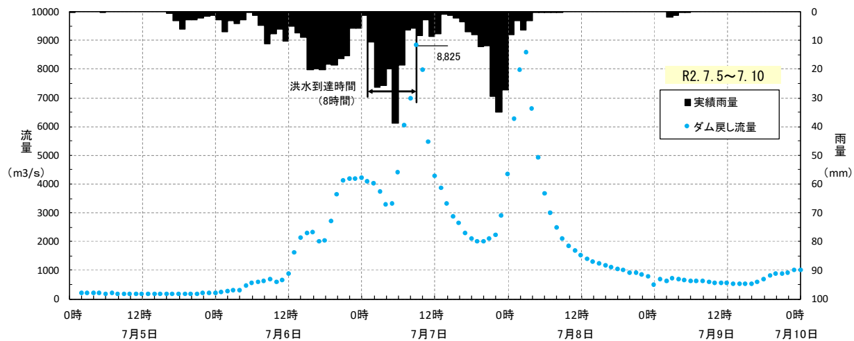
図 1-6-1 (4) Kinematic Wave法による洪水到達時間 (基準地点荒瀬)
