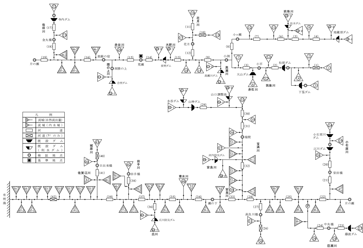
図 1-4-2 流出計算モデル模式図
