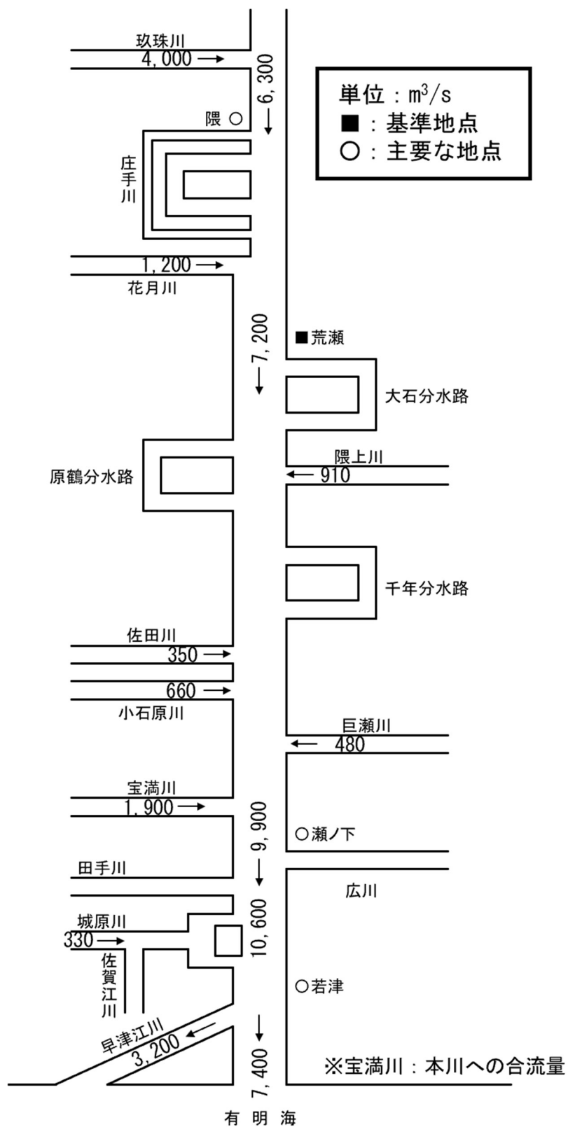
図 3-1 筑後川計画高水流量図
