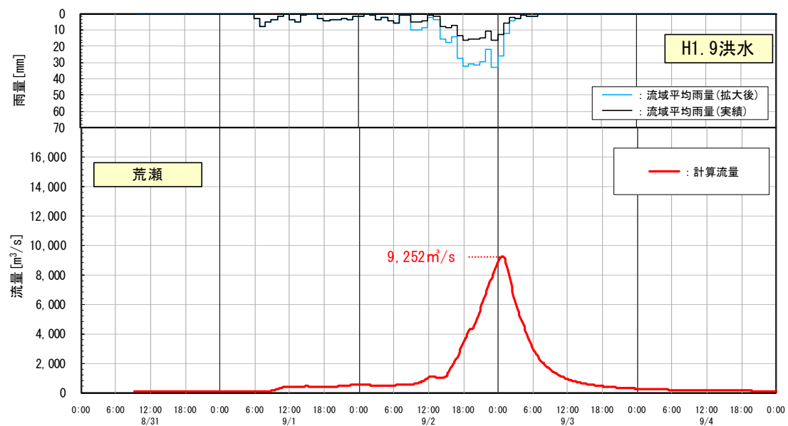
図 1-10-1 (2) 基本高水ハイドログラフ
