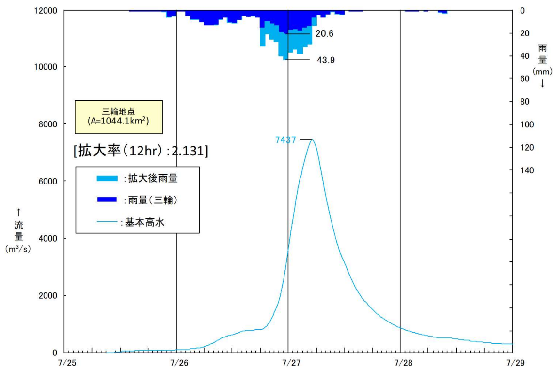
図 1.40(8) 基本高水ハイドロ(五ヶ瀬川:三輪 平成 11 年 7 月洪水 本川 W=1/100 降雨量変化倍率 1.1 倍後)
