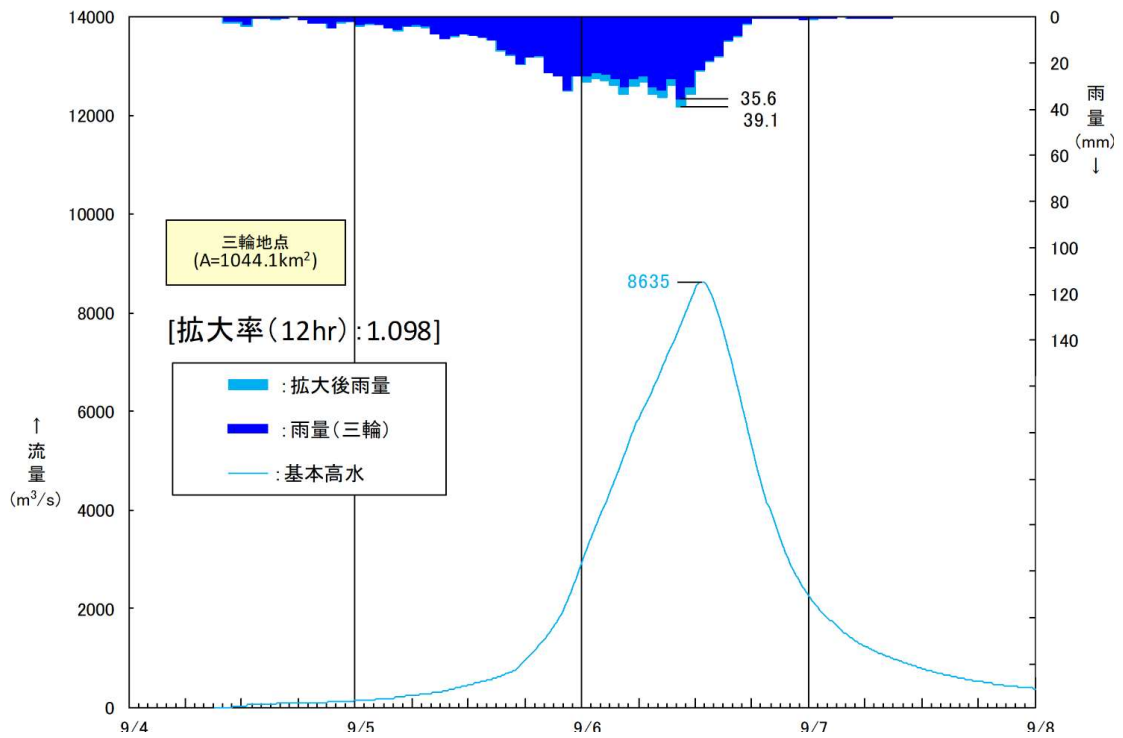
図 1.40(10) 基本高水ハイドロ(五ヶ瀬川:三輪 平成 17 年 9 月洪水 本川 W=1/100 降雨量変化倍率 1.1 倍後)
