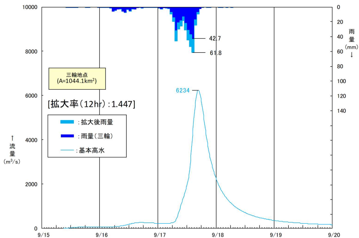
図 1.40(13) 基本高水ハイドロ(五ヶ瀬川:三輪 平成 29 年 9 月洪水 本川 W=1/100 降雨量変化倍率 1.1 倍後)
