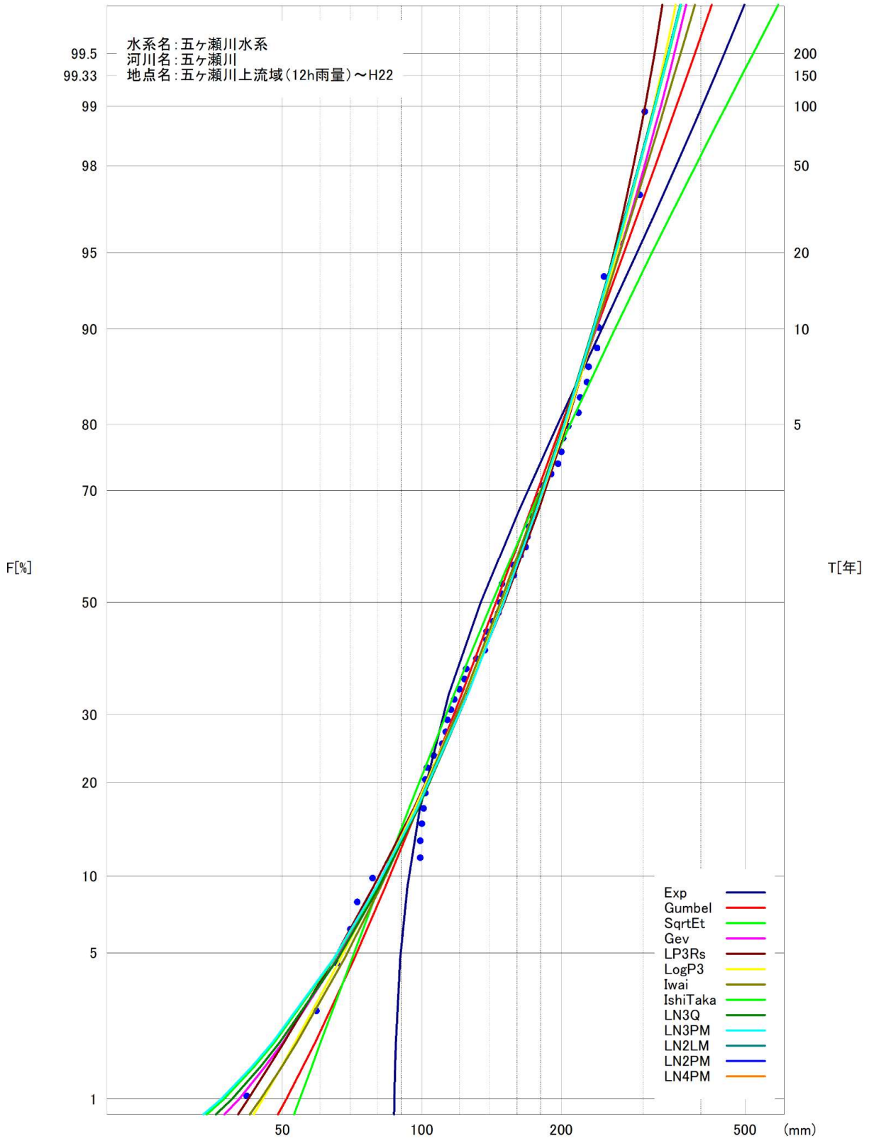
図 1.38(1) 雨量確率計算結果 (五ヶ瀬川上流域、12時間雨量、昭和29年~平成22年)
