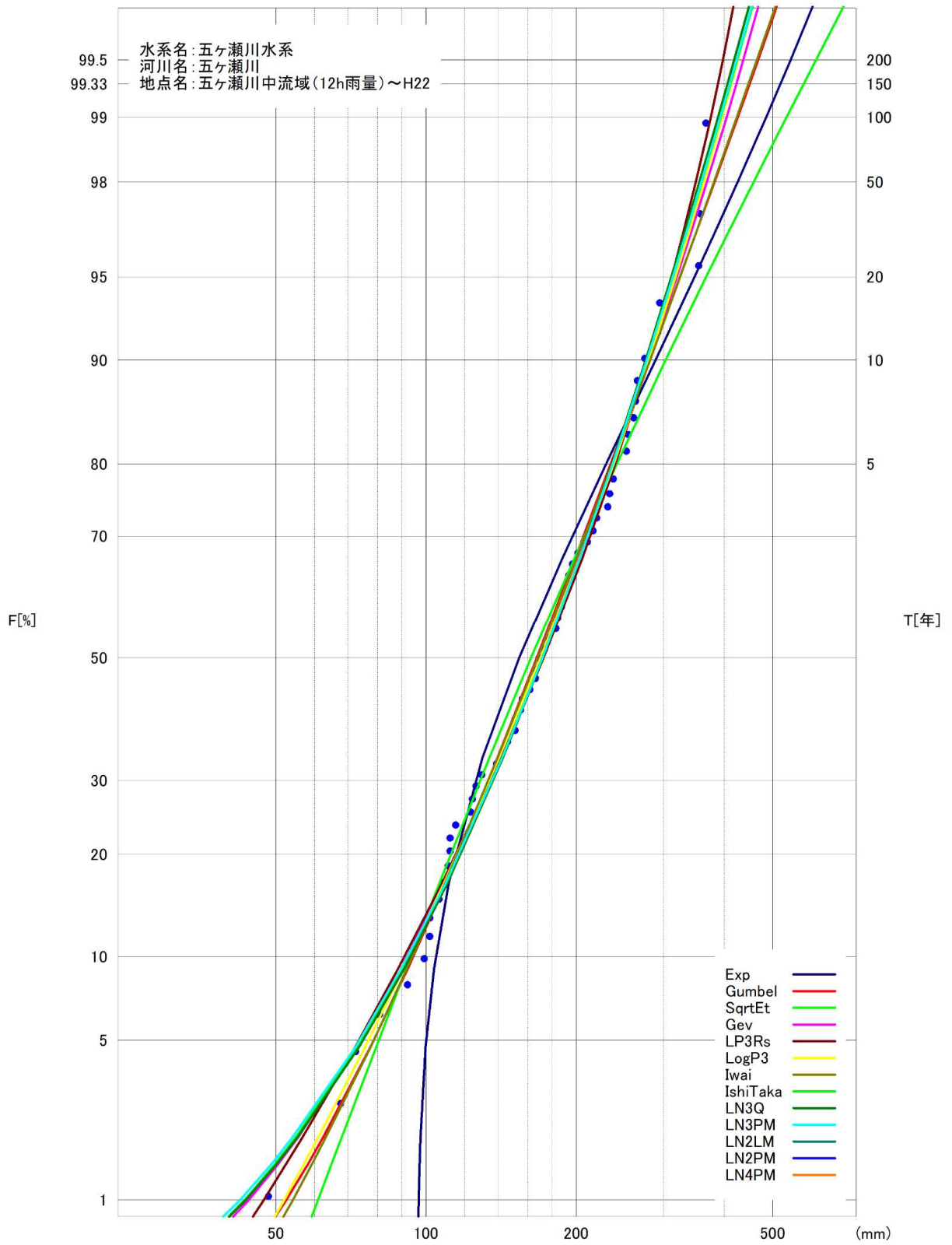
図 1.38(2) 雨量確率計算結果 (五ヶ瀬川中流域、12時間雨量、昭和29年~平成22年)
