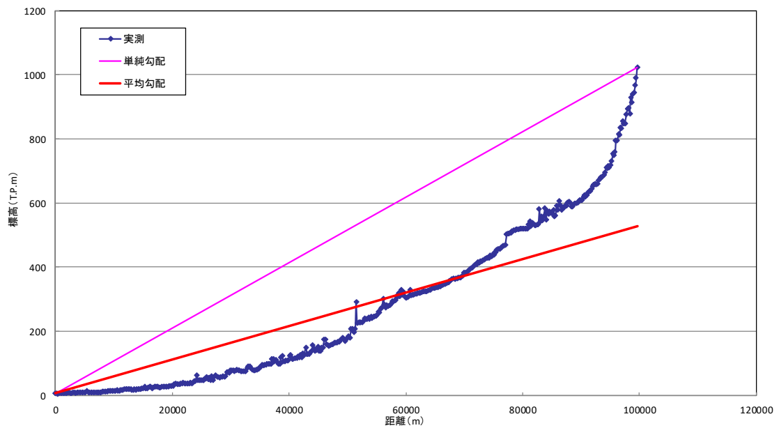
図 1.27 流路勾配、流路延長設定結果例 (三輪上流域)
