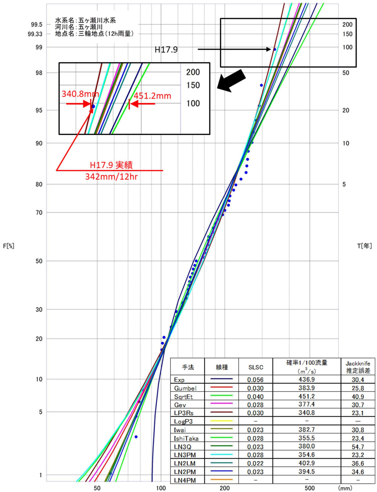
図 1-4 三輪地点における雨量確率評価 (昭和 29 年～平成 22 年 : 57 年間)
