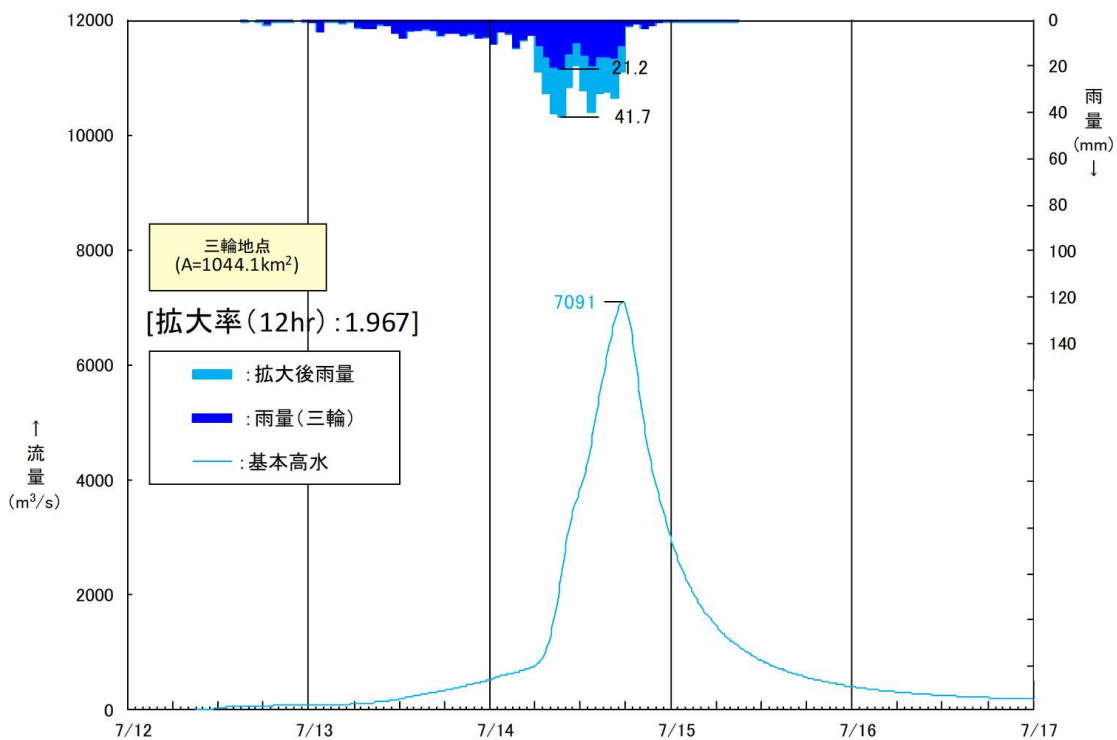
図 1.40(11) 基本高水ハイドロ(五ヶ瀬川:三輪 平成 19 年 7 月洪水 本川 W=1/100 降雨量変化倍率 1.1 倍後)
