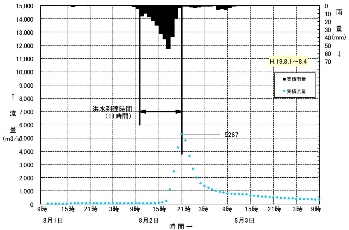
図 1.5(10) Kinematic Wave 法による洪水到達時間の検討 (H19.8 洪水)
