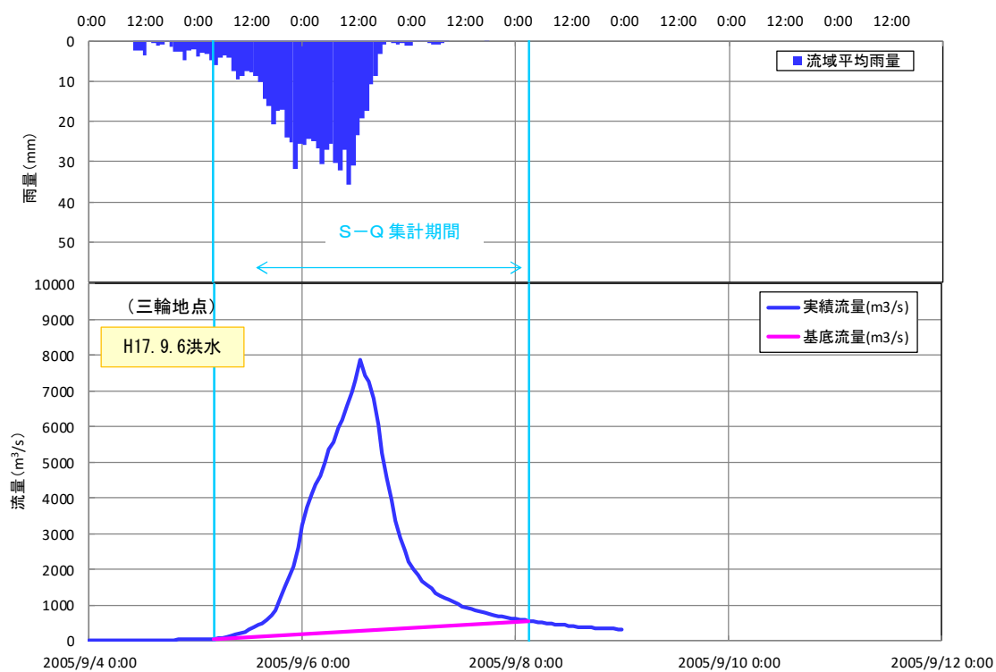
図 1.21 流域定数 K, P 設定洪水の実績波形図 (三輪地点)
