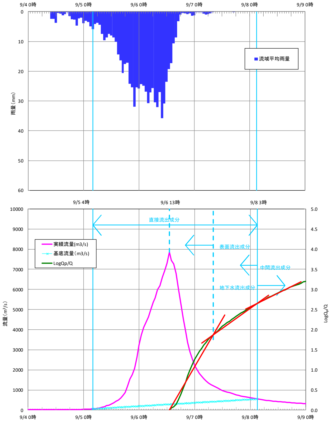
图 1.18 成分分離結果 (三輪地点 : H17.9 洪水)
