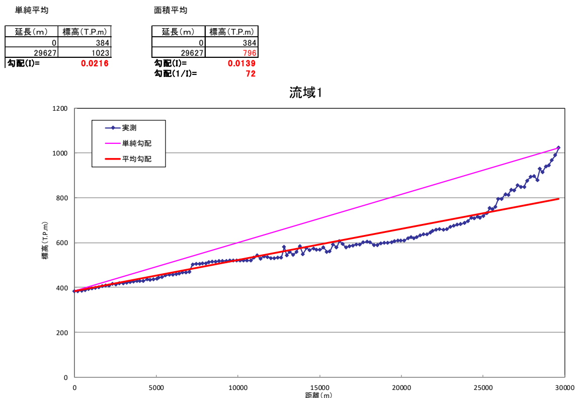
図 1.29 流域平均勾配の算定結果（流域 1）
