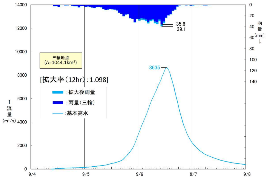
図 1.47 基本高水のハイドログラフ (昭和 46 年 8 月洪水 : 上) (平成 17 年 9 月洪水 : 下)
