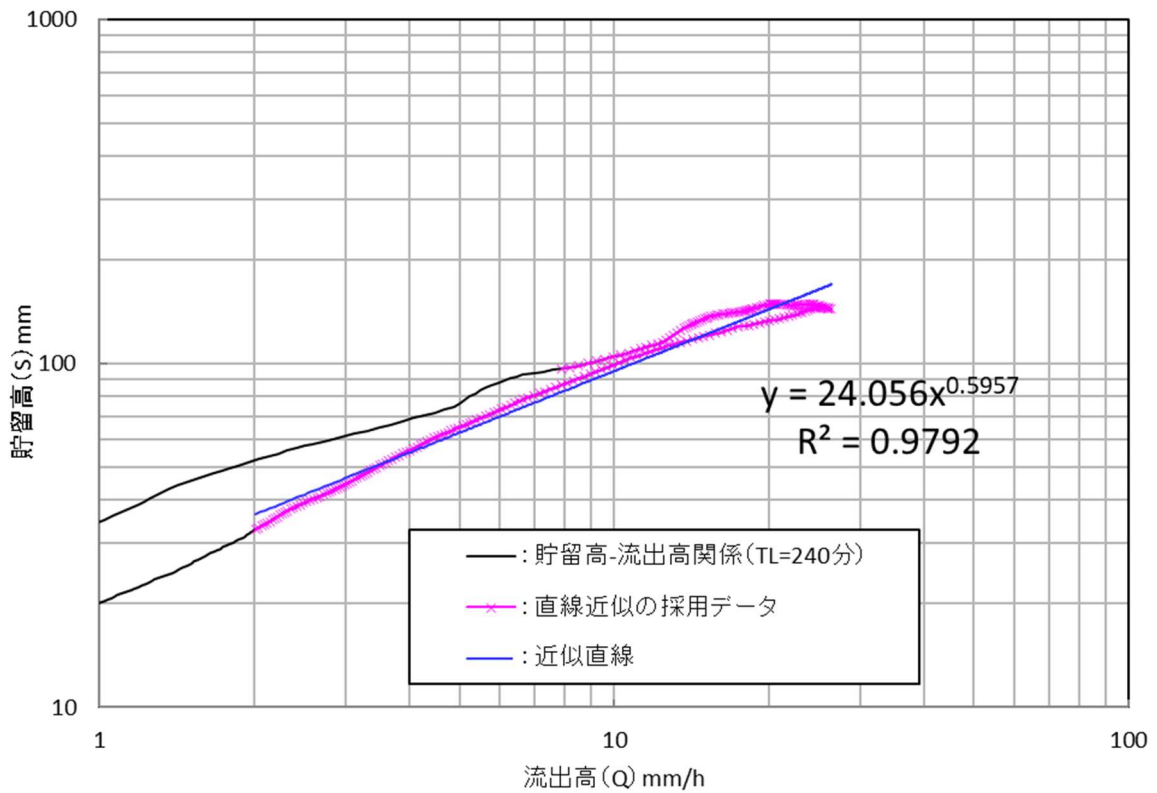
図 1.22 (2) 貯留高一流出高関係図 (三輪地点 H17.9 洪水)
