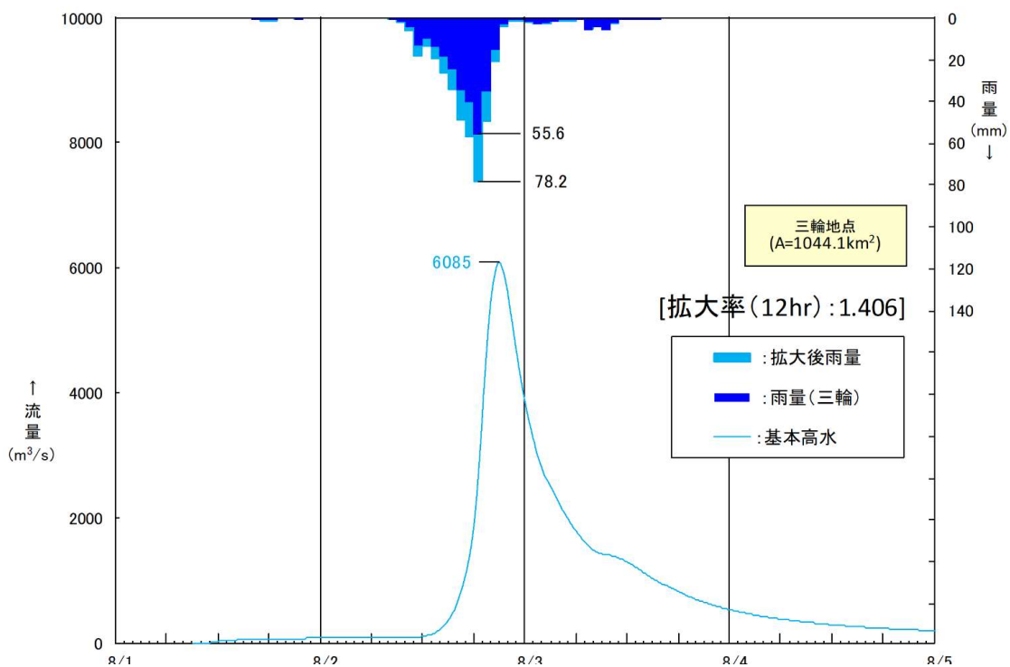
図 1.40(12) 基本高水ハイドロ(五ヶ瀬川:三輪 平成 19 年 8 月洪水 本川 W=1/100 降雨量変化倍率 1.1 倍後)
