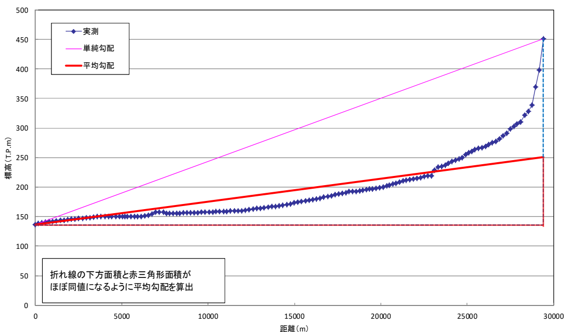
図 1-24 流域平均勾配の設定例
