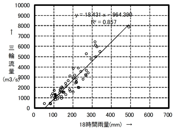
図 1.7(1) ピーク流量と流域平均時間雨量の相関図〔定義①〕
