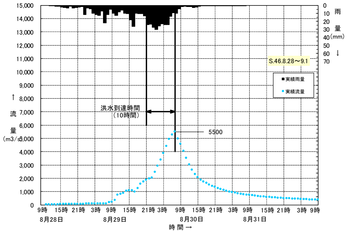
図 1.5(2) Kinematic Wave 法による洪水到達時間の検討 (S46.8 洪水)
