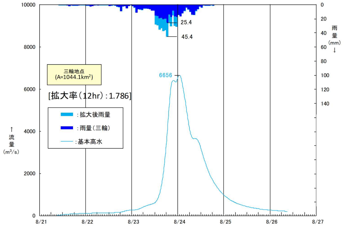
图 1.40(1) 基本高水ハイドロ(五ヶ瀬川:三輪 昭和 39 年 8 月洪水 本川 W=1/100 降雨量変化倍率 1.1 倍後)
