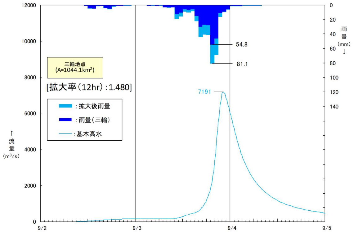
図 1.40(5) 基本高水ハイドロ(五ヶ瀬川:三輪 平成 5 年 9 月洪水 本川 W=1/100 降雨量変化倍率 1.1 倍後)
