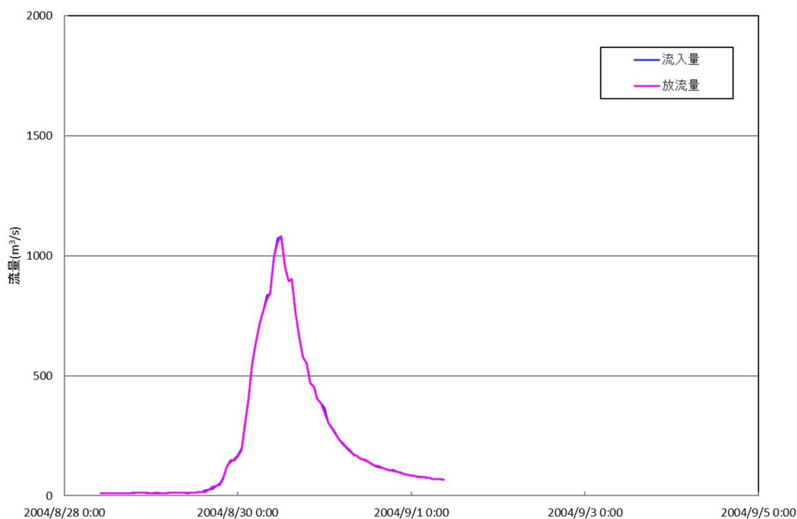
図 1.13 桑野内ダム流入量、放流量（平成 16 年 8 月洪水）
