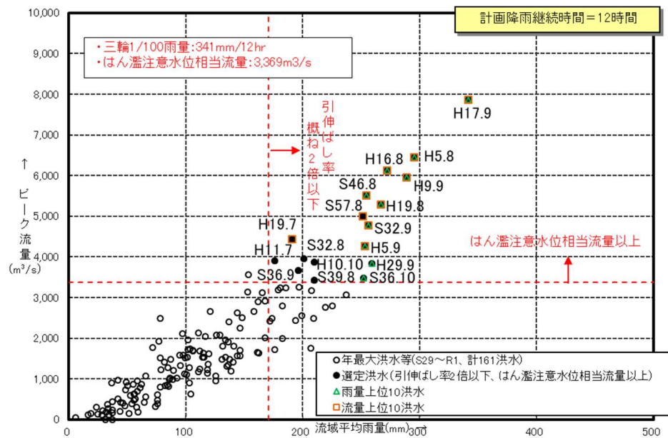
五ヶ瀬川三輪地点におけるピーク流量と流域平均雨量の関係
