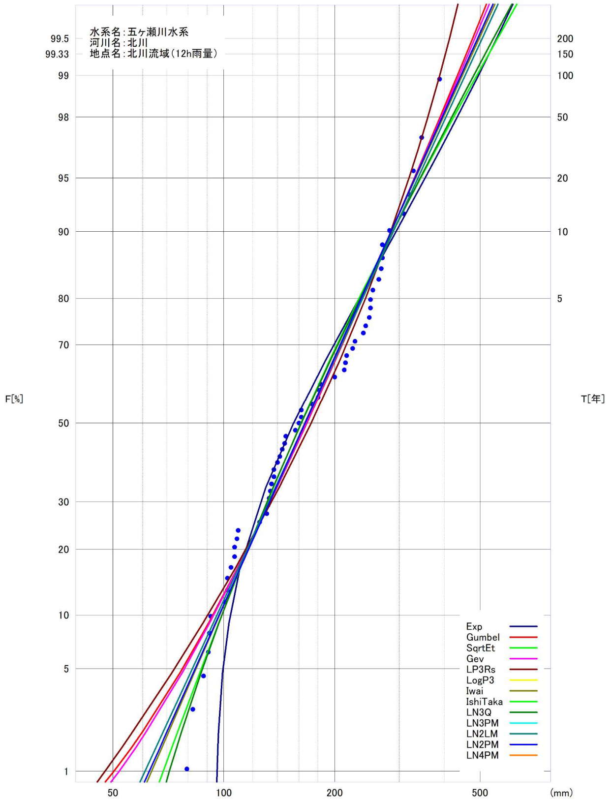
図 1.38(5) 雨量確率計算結果 (北川流域、12時間雨量、昭和29年～平成22年)
