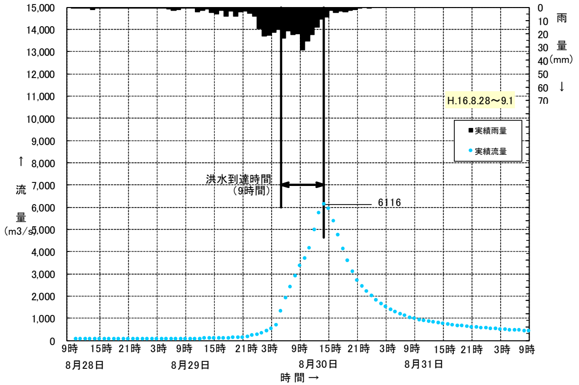
図 1.5(7) Kinematic Wave 法による洪水到達時間の検討 (H16.8 洪水)
