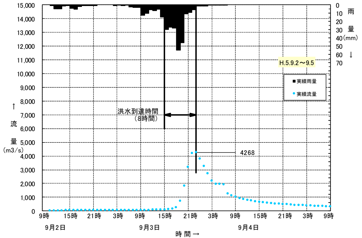
図 1.5(5) Kinematic Wave 法による洪水到達時間の検討 (H5.9 洪水)
