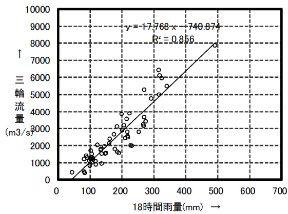
図 1.7(2) ピーク流量と流域平均時間雨量の相関図〔定義②〕
