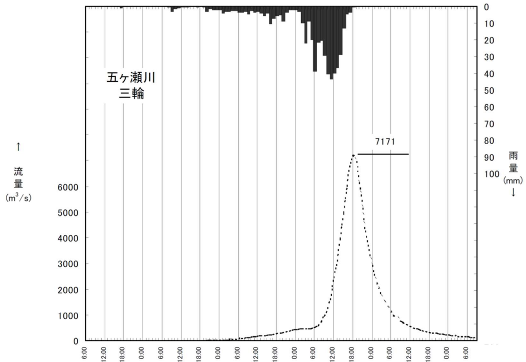
図 1-1 基本高水ハイドログラフ (平成9年9月型)
