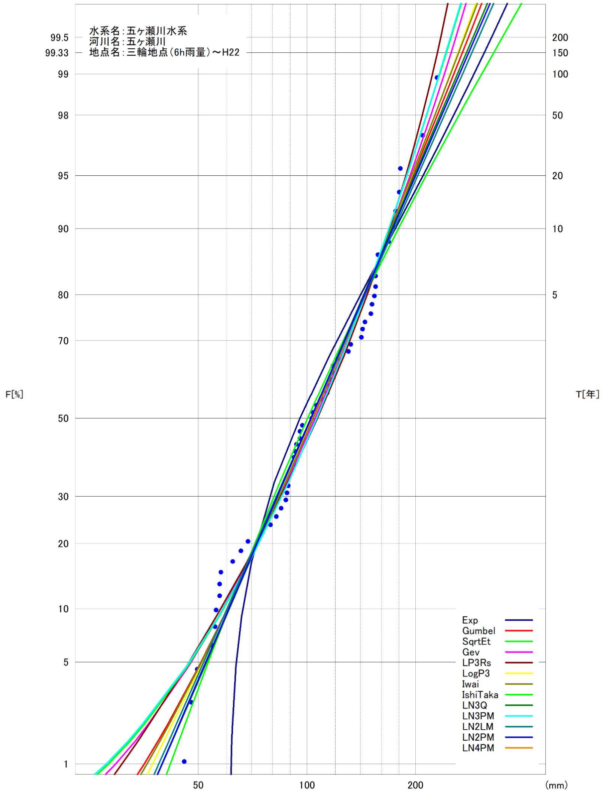
図 1.39 雨量確率計算結果 (三輪地点、6時間雨量、昭和29年~平成22年)
