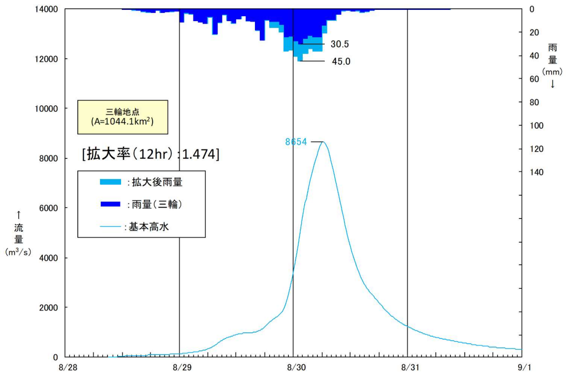
图 1.40(2) 基本高水ハイドロ(五ヶ瀬川:三輪 昭和 46 年 8 月洪水 本川 W=1/100 降雨量変化倍率 1.1 倍後)
