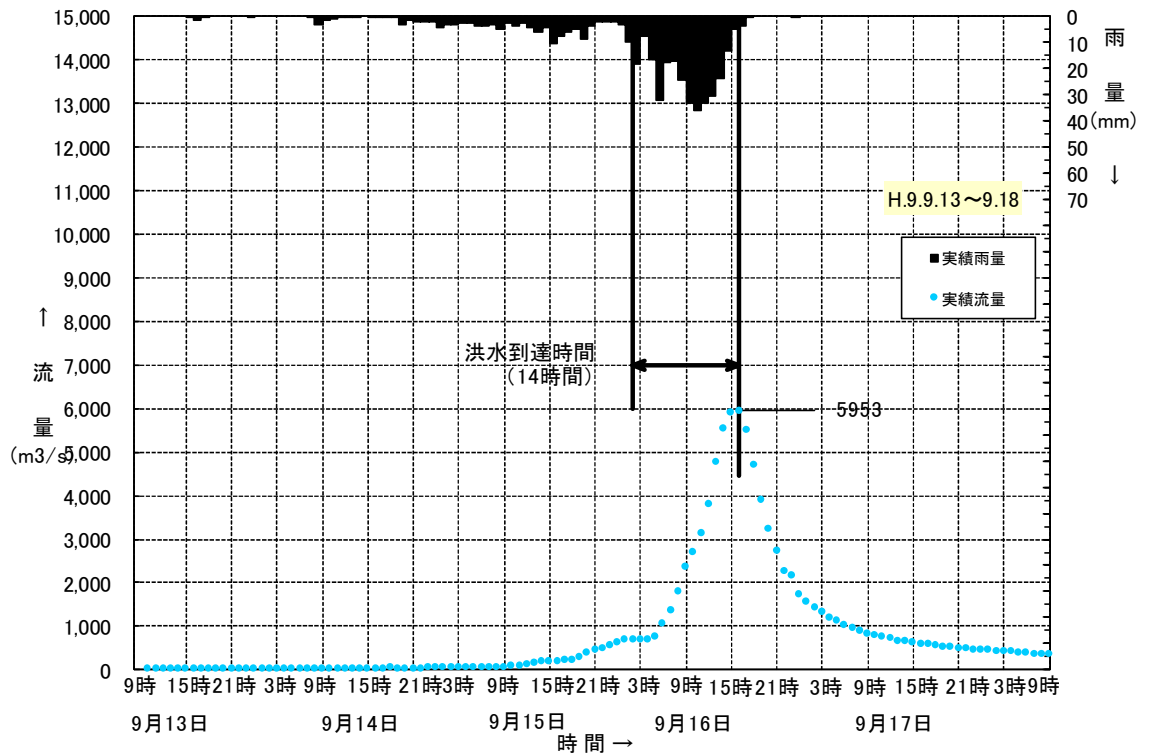
図 1.5(6) Kinematic Wave 法による洪水到達時間の検討 (H9.9 洪水)
