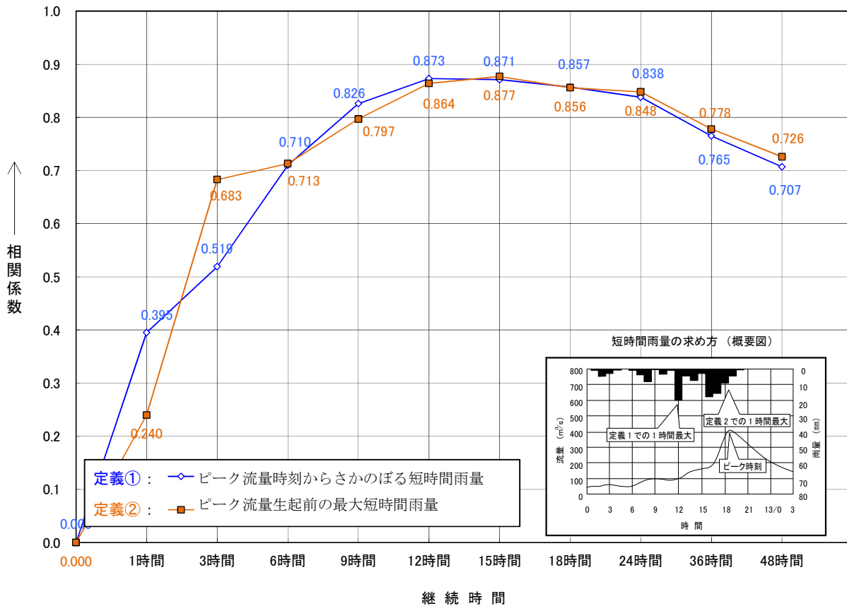
図 1.6 三輪地点ピーク流量と降雨継続時間の相関図 〔対象洪水：年最大流量発生洪水（S31年以降）〕
