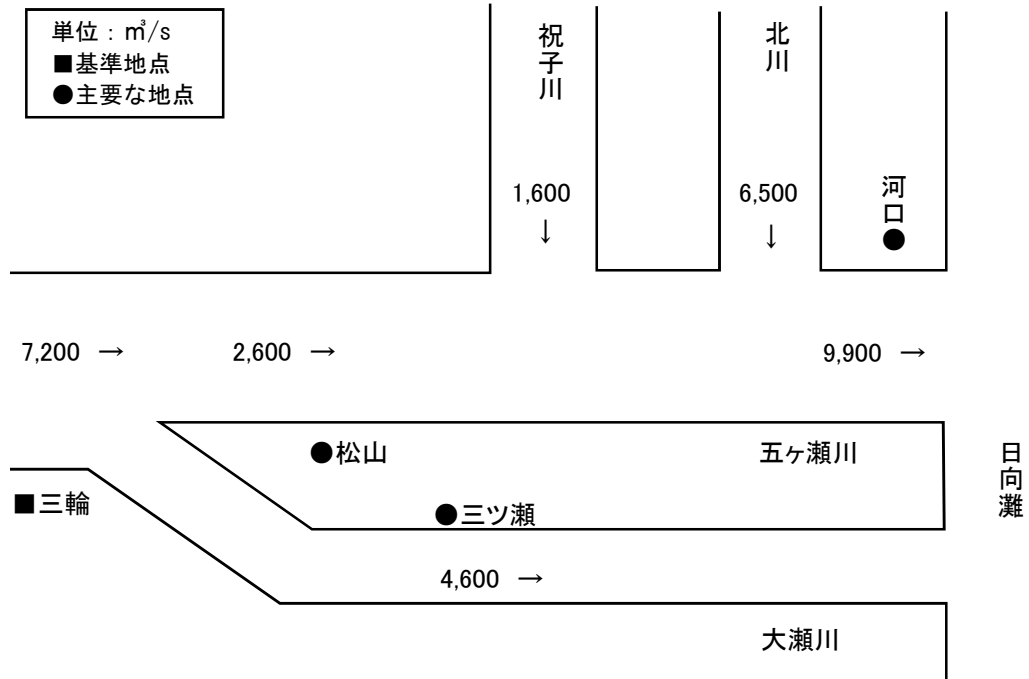
図 3-1 五ヶ瀬川計画高水流量図
