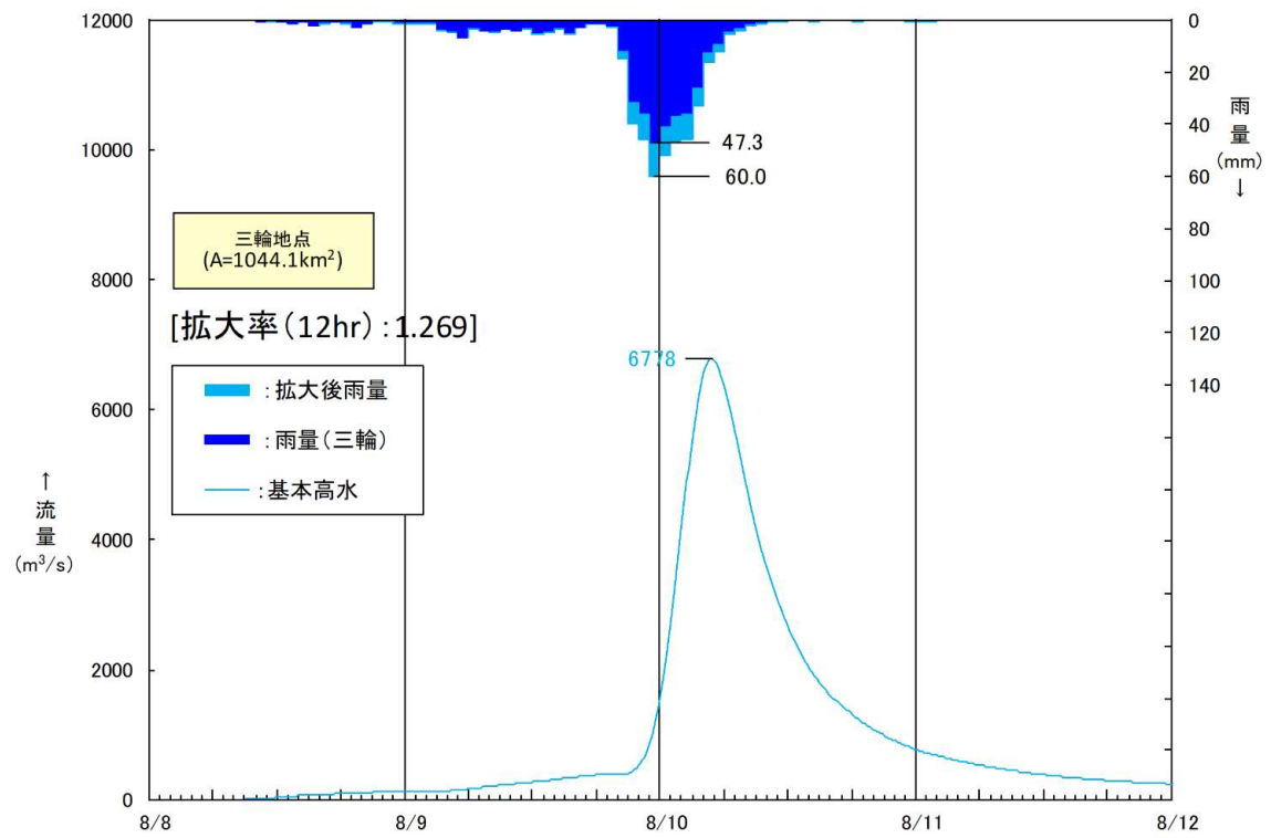
図 1.40(4) 基本高水ハイドロ(五ヶ瀬川:三輪 平成 5 年 8 月洪水 本川 W=1/100 降雨量変化倍率 1.1 倍後)
