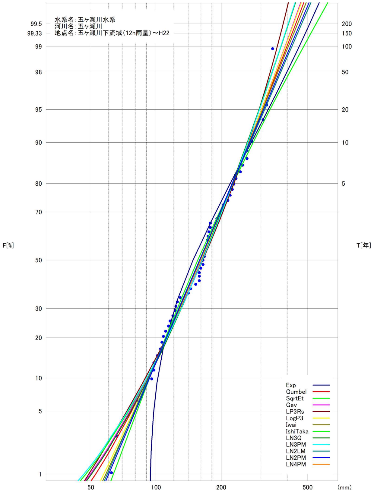
図 1.38(3) 雨量確率計算結果（五ヶ瀬川下流域、12時間雨量、昭和29年～平成22年）
