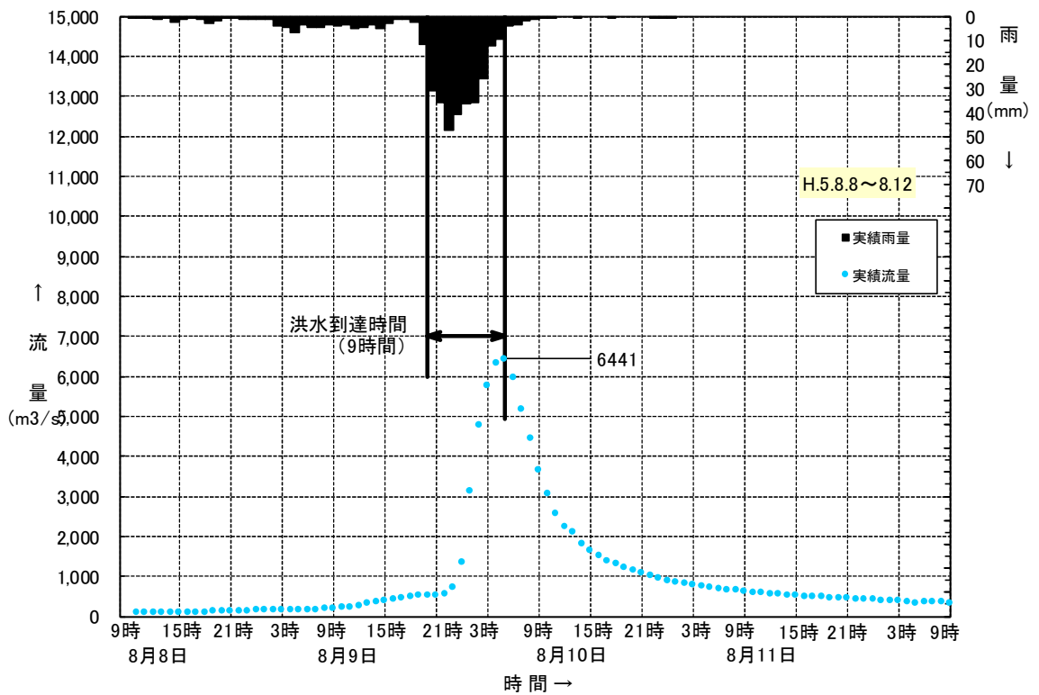
図 1.5(4) Kinematic Wave 法による洪水到達時間の検討 (H5.8 洪水)
