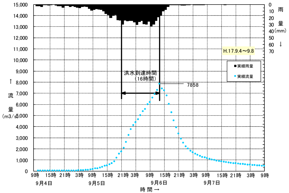
図 1.5(8) Kinematic Wave 法による洪水到達時間の検討 (H17.9 洪水)
