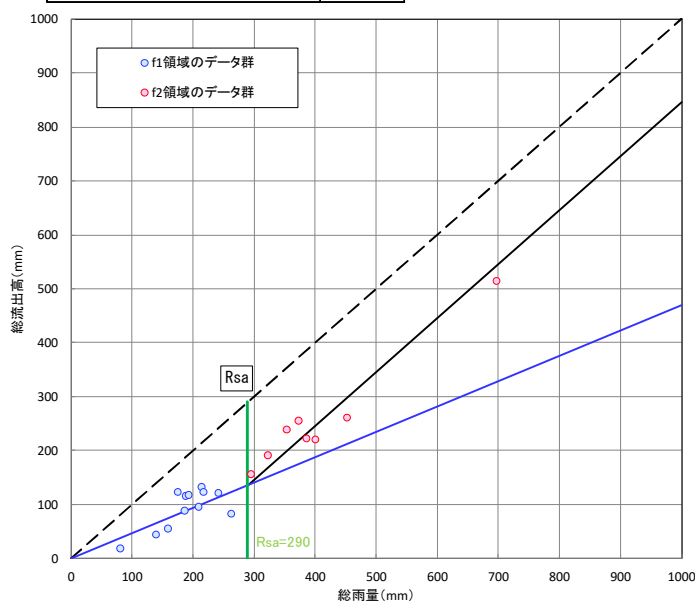
図 1.19 総雨量と総流出高の関係（三輪地点）
