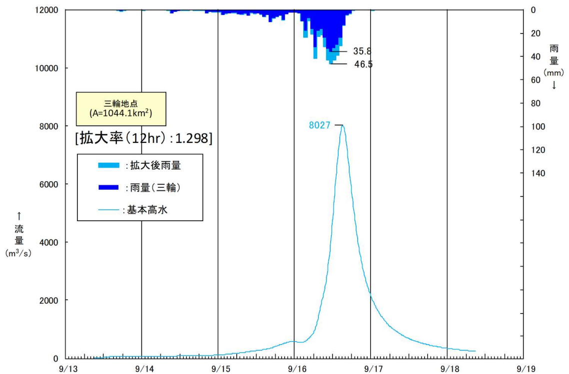
図 1.40(6) 基本高水ハイドロ(五ヶ瀬川:三輪 平成年 9 月洪水 本川 W=1/100 降雨量変化倍率 1.1 倍後)
