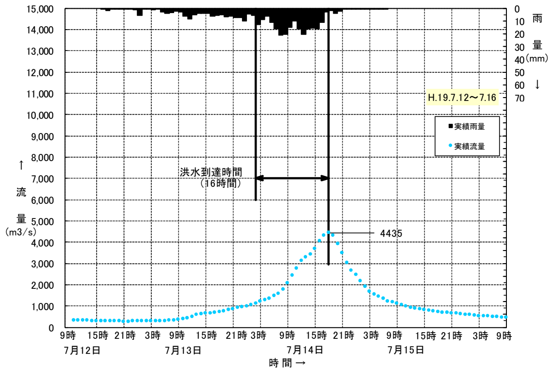
図 1.5(9) Kinematic Wave 法による洪水到達時間の検討 (H19.7 洪水)
