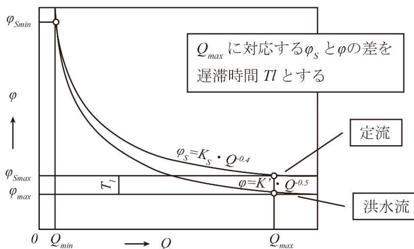
図 1.33 定流の貯留関数 \varphi_s と洪水流の貯留関数 \varphi の関係
