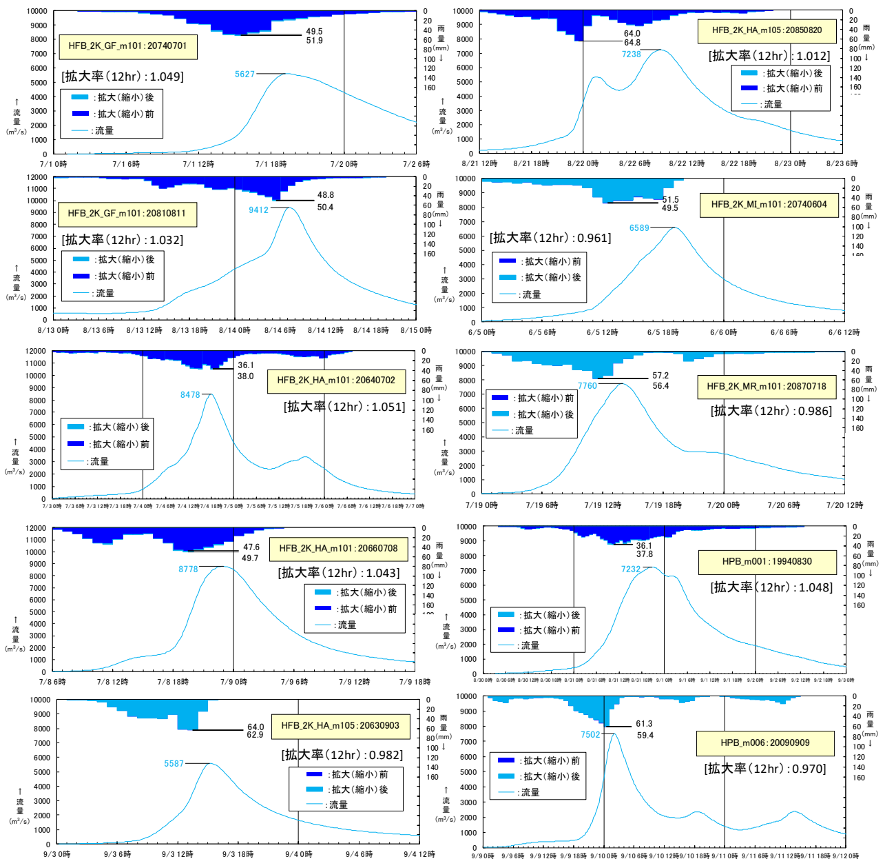
図 1.42 抽出した予測降雨波形群によるハイドログラフ
