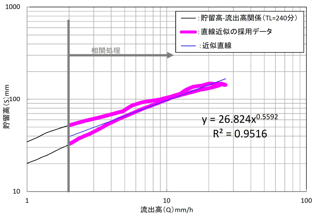
図 1.22(1) 流出高と貯留高の関係 (三輪：平成 17 年 9 月 6 日洪水)
