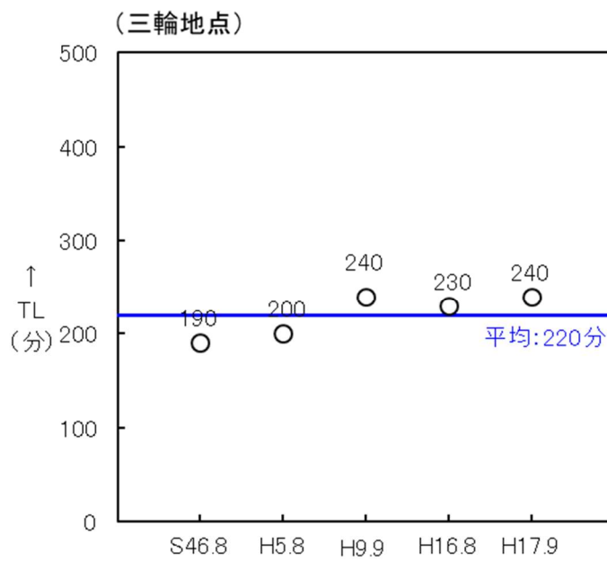
図 1.23 TL の設定状況 (各洪水と平均値の関係)
