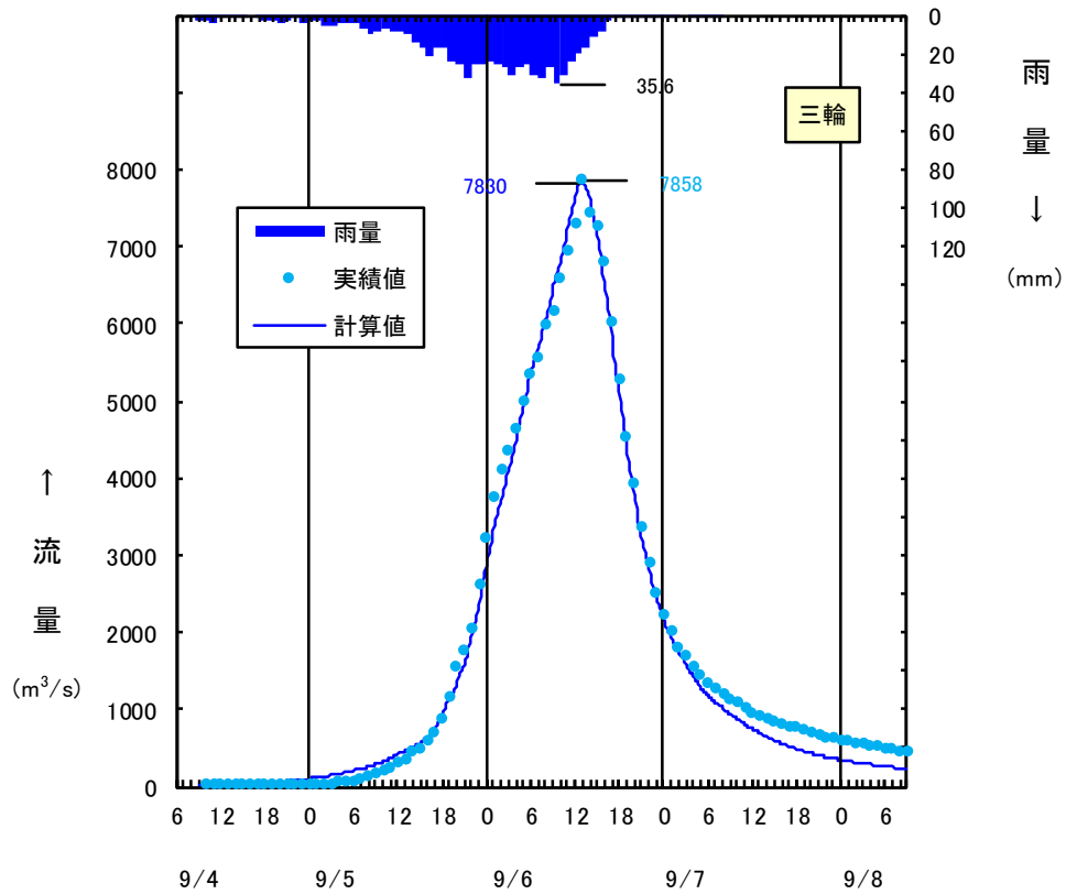
図 1-10 平成 17 年 9 月洪水再現計算結果 (三輪地点)
