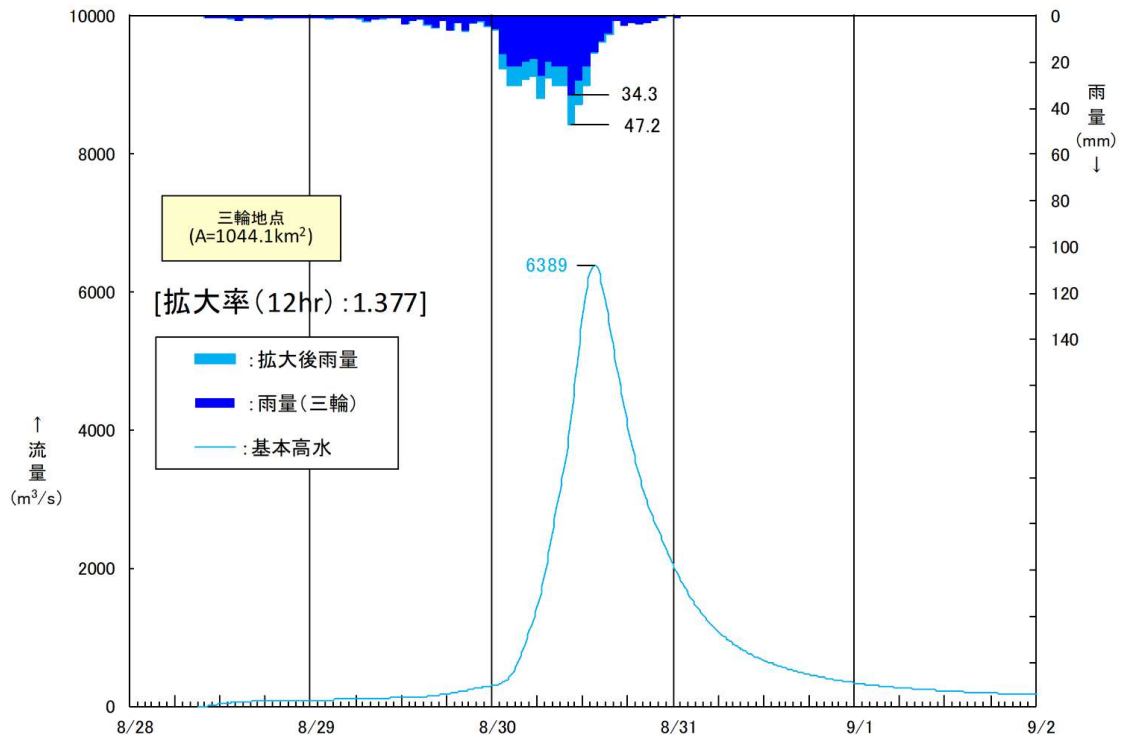
図 1.40(9) 基本高水ハイドロ(五ヶ瀬川:三輪 平成 16 年 8 月洪水 本川 W=1/100 降雨量変化倍率 1.1 倍後)
