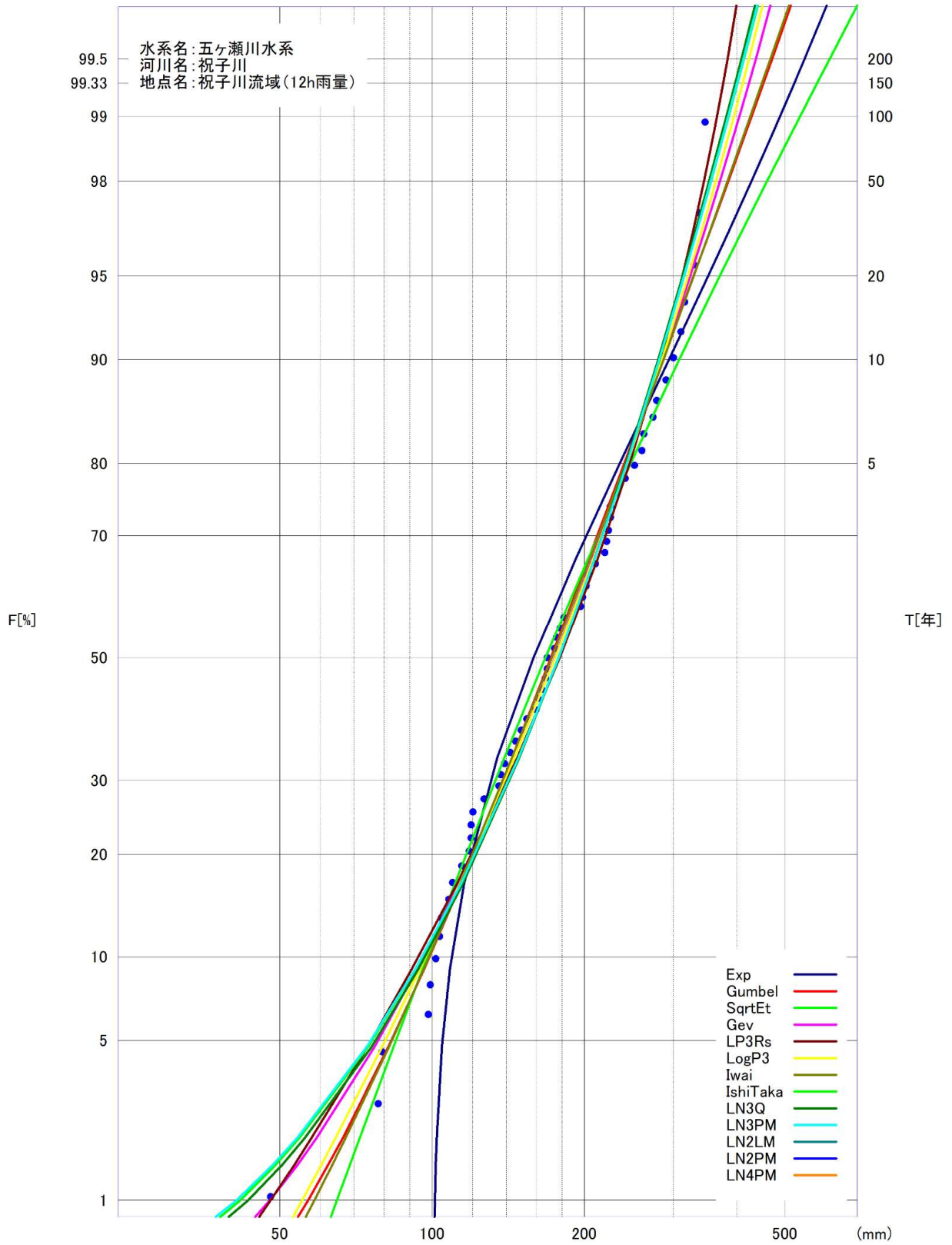
図 1.38(4) 雨量確率計算結果 (祝子川流域、12時間雨量、昭和29年～平成22年)
