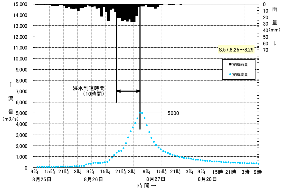
図 1.5(3) Kinematic Wave 法による洪水到達時間の検討 (S57.8 洪水)
