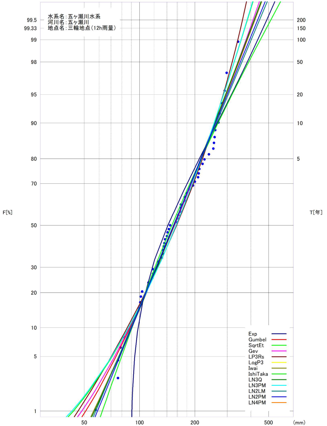
図 1.9 雨量確率計算結果 (三輪地点、12 時間雨量、昭和 29 年～平成 22 年)
