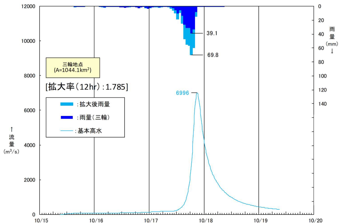
図 1.40(7) 基本高水ハイドロ(五ヶ瀬川:三輪 平成 10 年 10 月洪水 本川 W=1/100 降雨量変化倍率 1.1 倍後)
