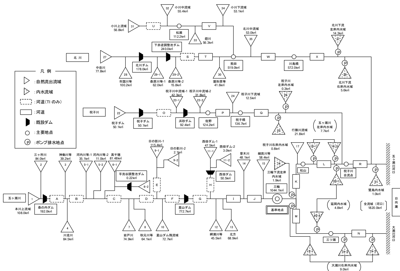
図 1.31 流出解析モデル図
