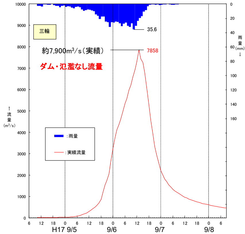
図 1.45 平成17年9月実績洪水結果(基準地点三輪)
