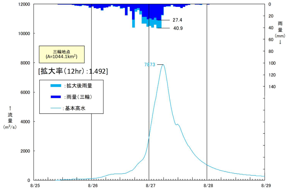
図 1.40(3) 基本高水ハイドロ(五ヶ瀬川:三輪 昭和 57 年 8 月洪水 本川 W=1/100 降雨量変化倍率 1.1 倍後)
