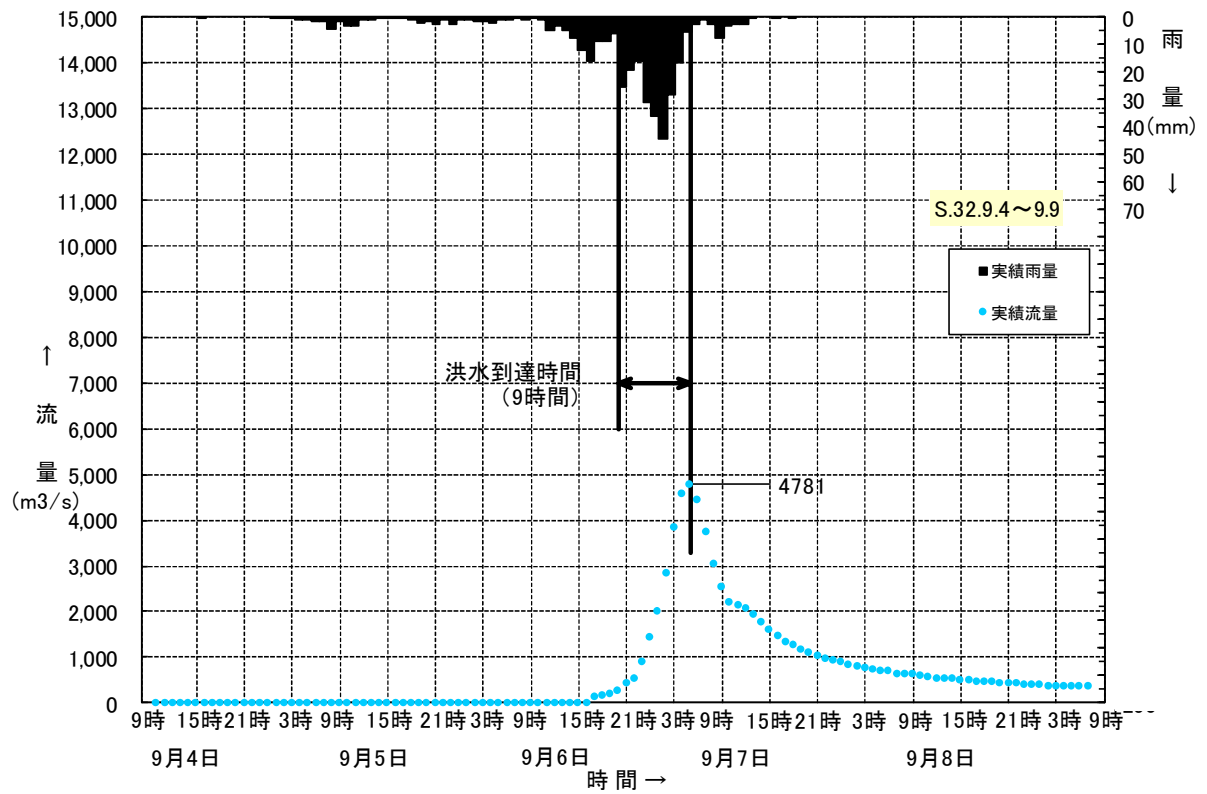
図 1.5(1) Kinematic Wave 法による洪水到達時間の検討 (S32.9 洪水)
