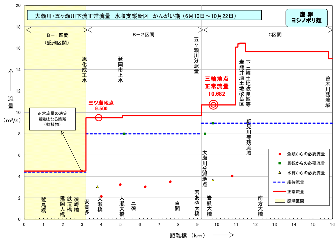
図 6-1(1) 大瀬川・五ヶ瀬川の正常流量（灌漑期：6/10～10/22（期間1））
