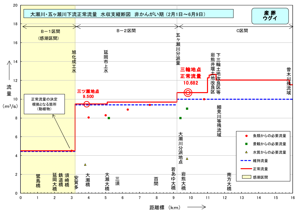
図 6-1 (3) 大瀬川・五ヶ瀬川の正常流量 (非灌漑期 : 2/1～6/9 (期間 3))
