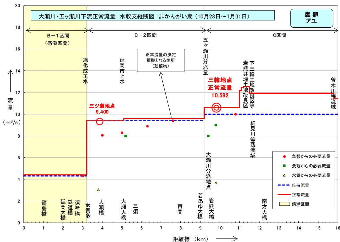
図 6-1 (2) 大瀬川・五ヶ瀬川の正常流量 (非灌漑期 : 10/23～1/31 (期間 2))
