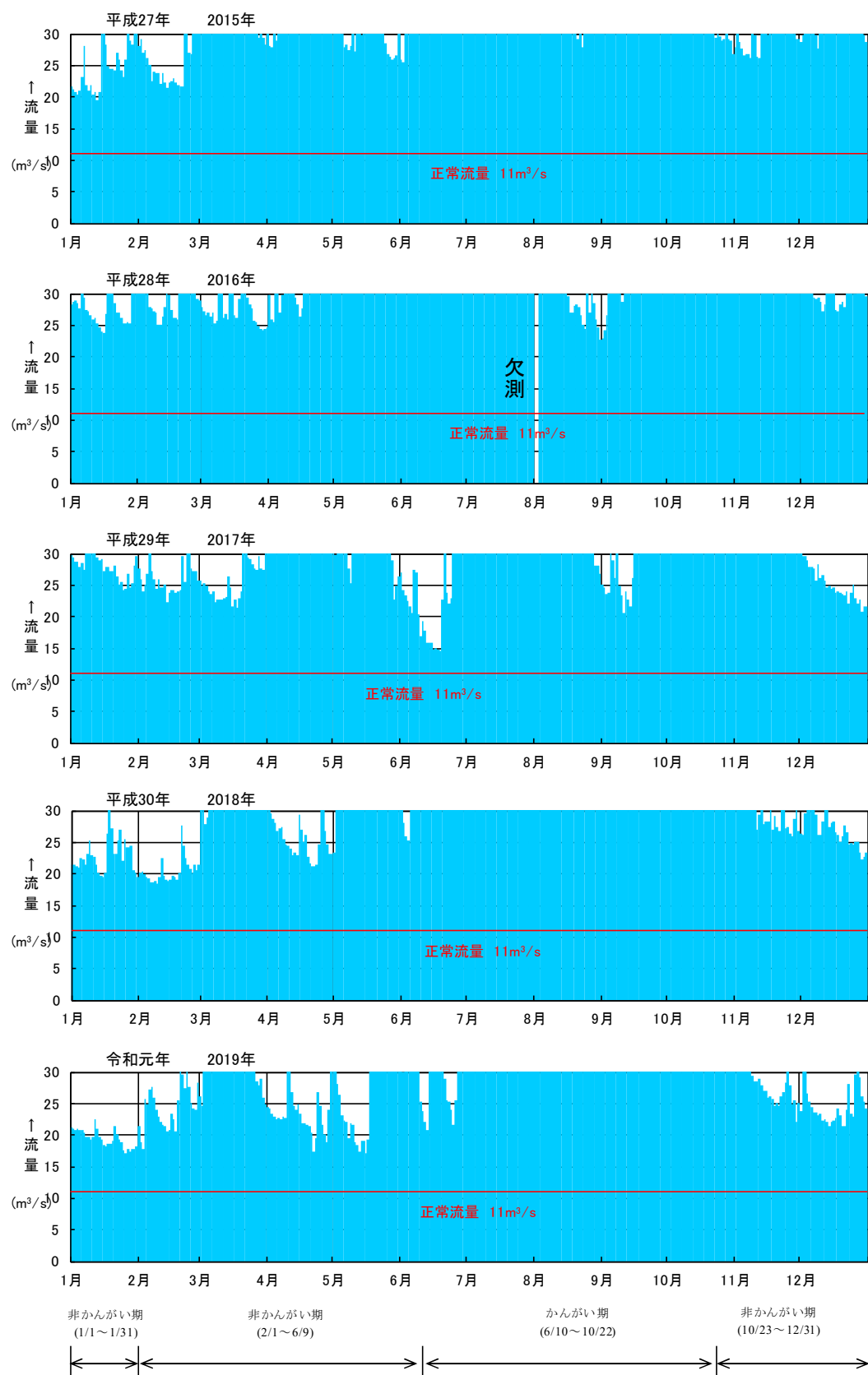
図 6-2 (2) 日平均流量図（三輪地点：平成 27 年～令和元年）
