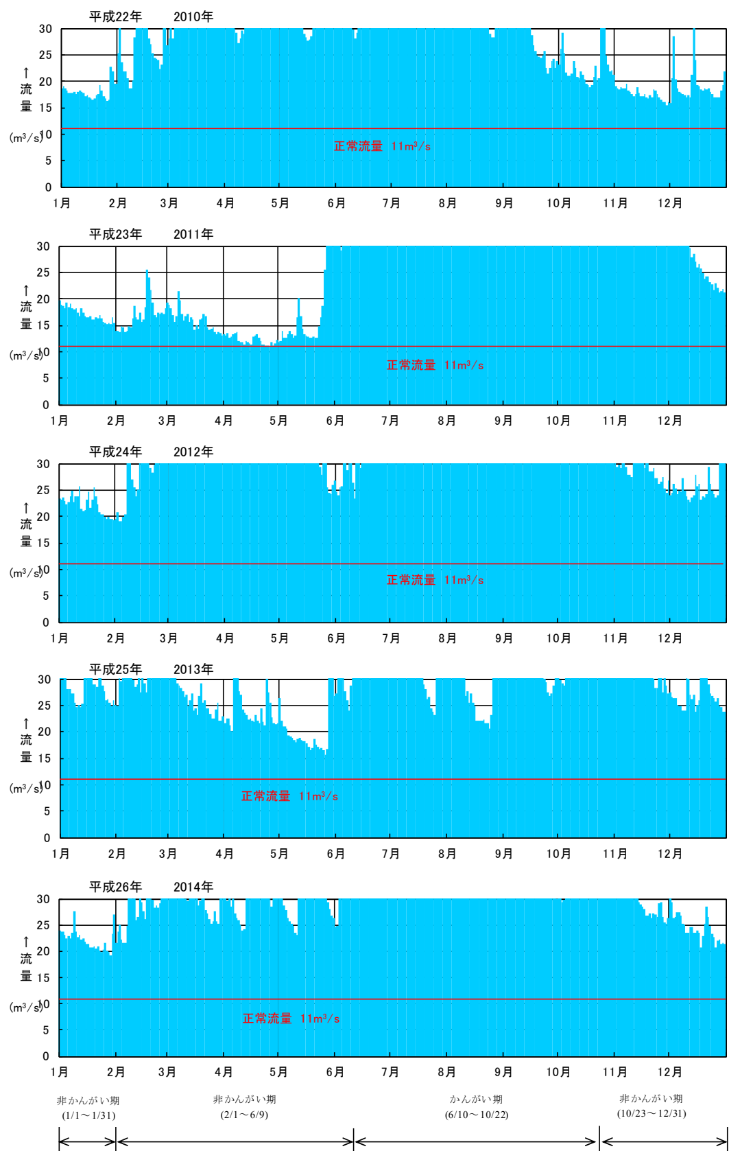
図 6-2(1) 日平均流量図（三輪地点：平成 22 年～平成 26 年）
