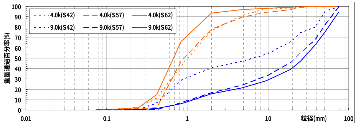
図 2.2.3 河床材料の経年変化
