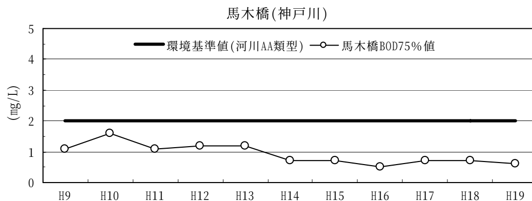
図 6.5 神戸川の水質経年変化 (BOD)
