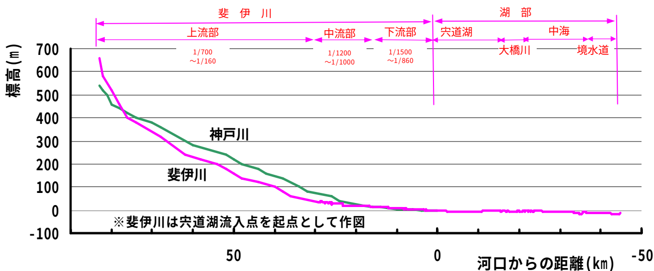
図 8.1.1 河道縦断面図(斐伊川、神戸川)
