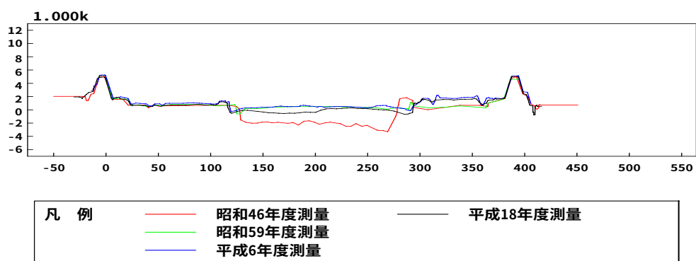
図 8.4.2 横断形状の経年変化 (1.0k)
