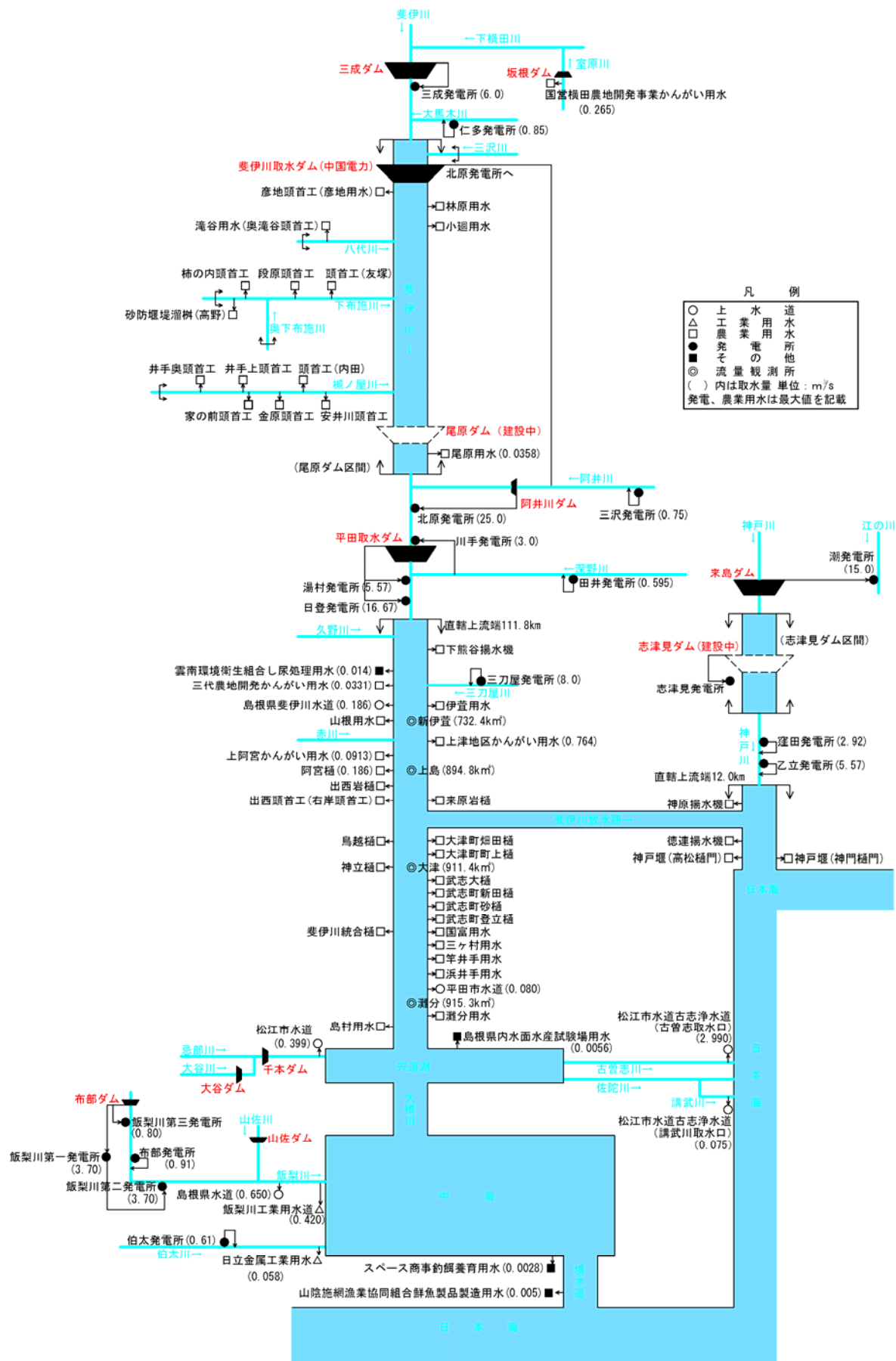
図 5.2.2 琵琶湖水系における主な取水
