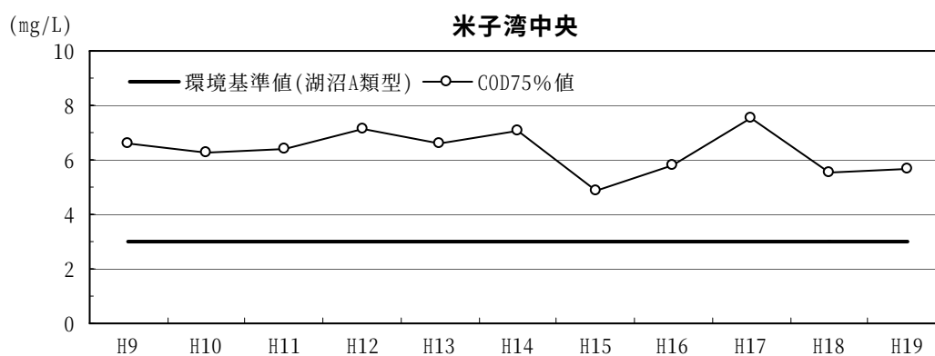
図 6.6 中海・宍道湖の水質経年変化 (COD)
