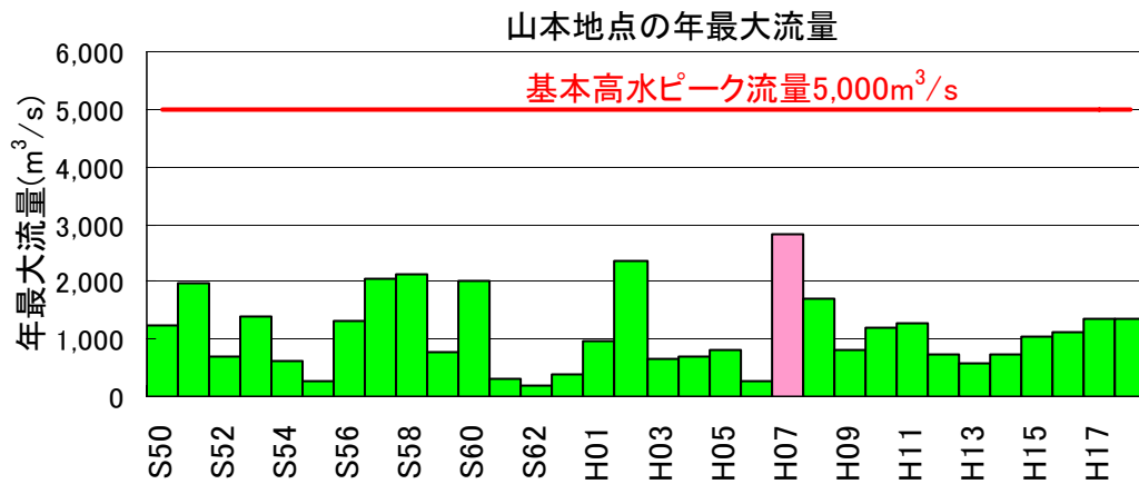
図4-1 年最大流量 (計算流量：山本地点)
