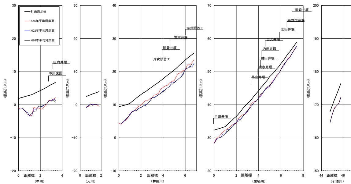
図－8.1(3) 中川・元川・林田川・栗栖川・引原川平均河床高縦断図
