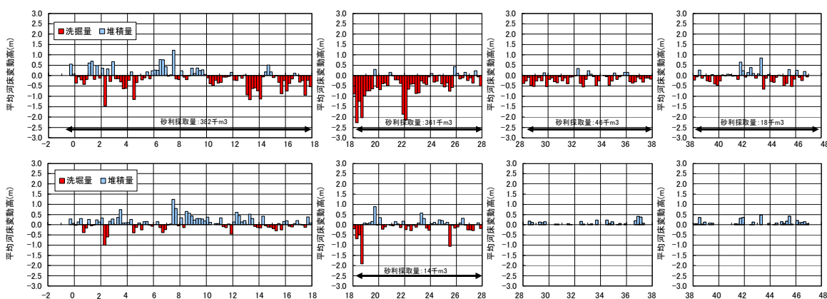
図－8.1(2) 揖保川における河床変動の状況(上図：S45～H02 下図：H02～H16)
