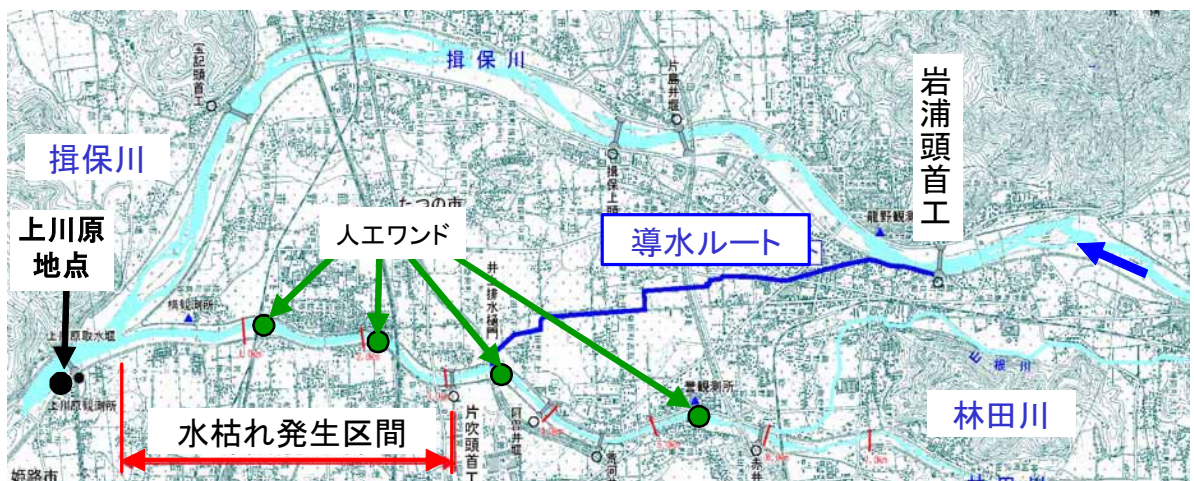
図－6.5 揖保川導水ルートと水枯れ区間
