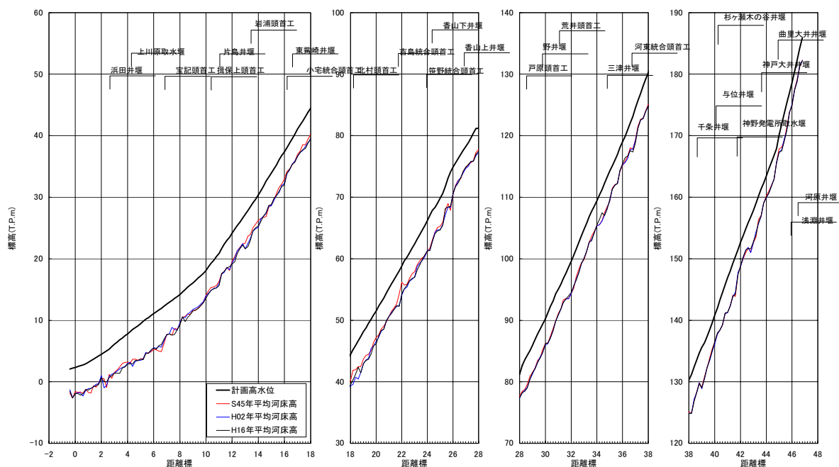
図－8.1(1) 揖保川平均河床高縦断面図
