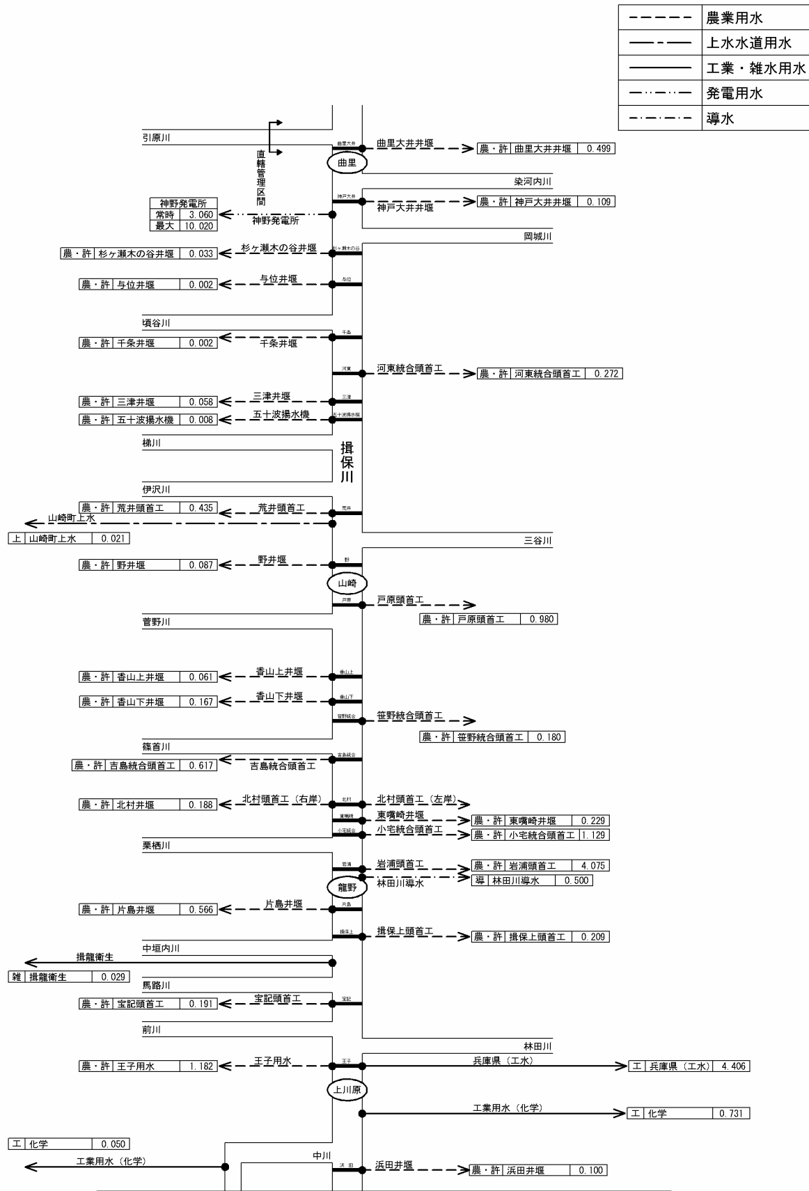
図-5.2 揖保川水系 水利模式図
