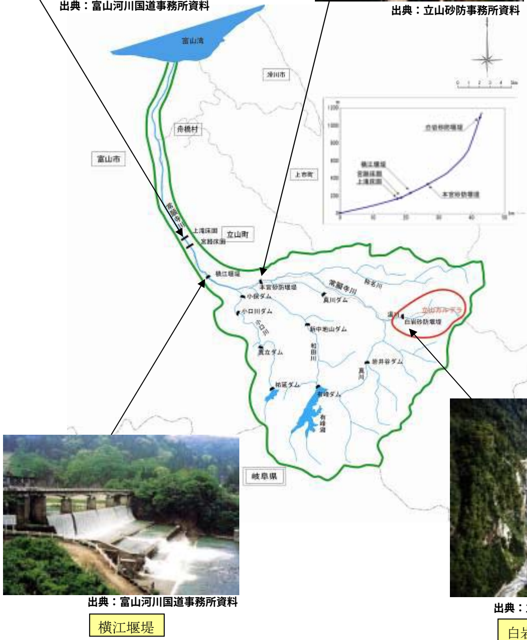
図 4-2-4 主要な河川関係構造物位置図
