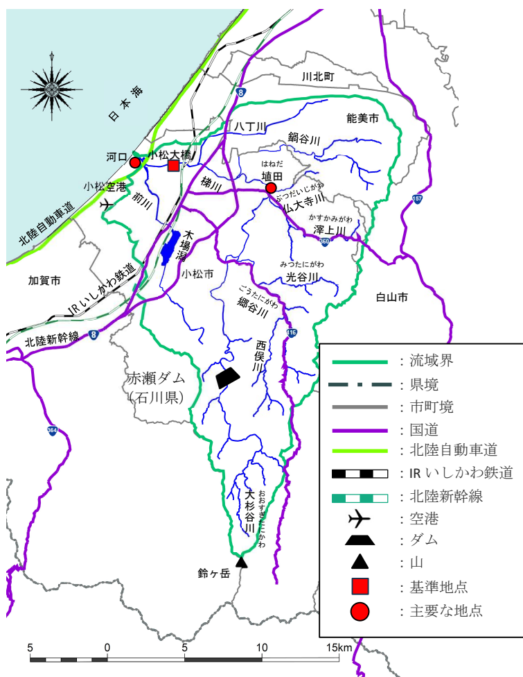
図 1-1 梯川流域図
