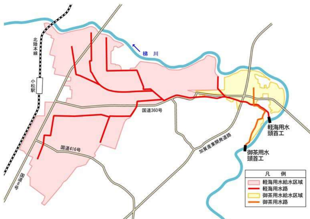
図 5-3 軽海用水及び御茶用水の給水区域図
