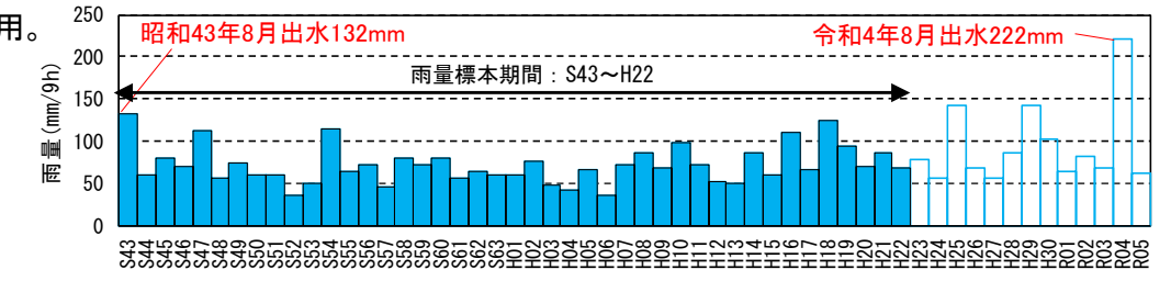
年最大9時間雨量(基準地点小松大橋上流域平均雨量)
