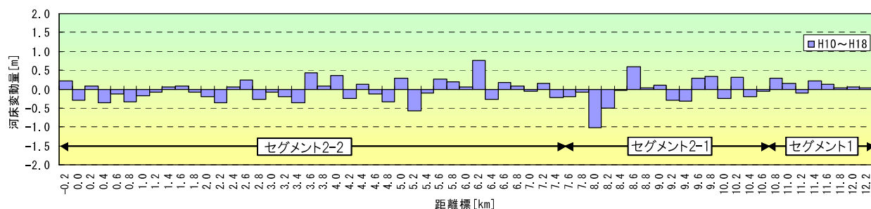
図 2-1 (4) 低水路内河床変動量経年変化図 (H10~H18)
