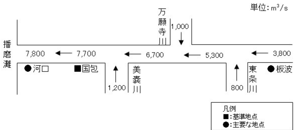
加古川計画高水流量図
