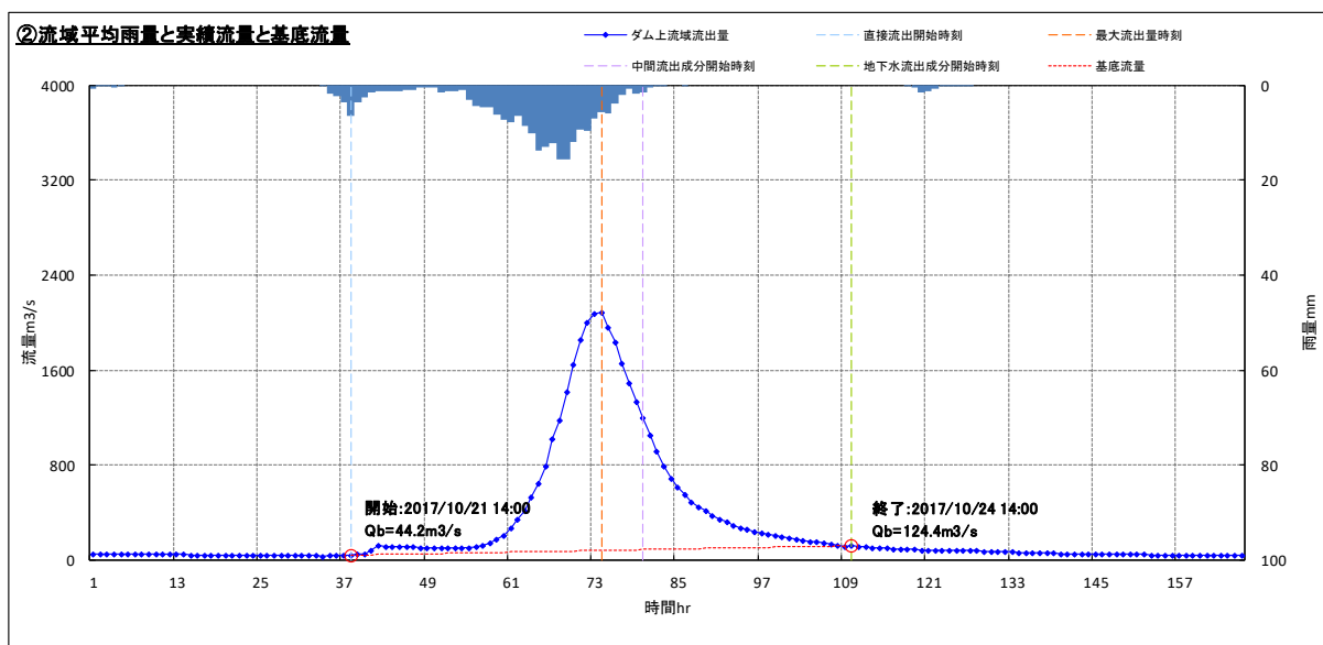
図一 1.4.14 貯留高－流出高関係図(船町地点：H29.10.22洪水)
