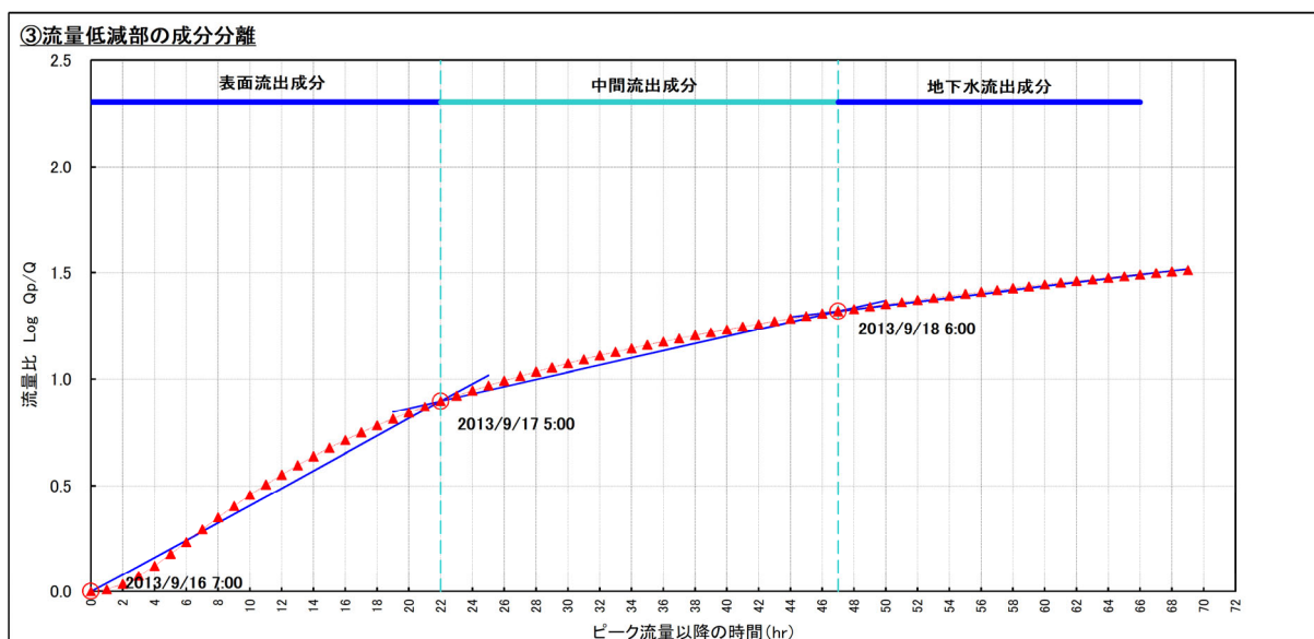
図－ 1.4.8 (2) 成分分離の事例（国包地点：H25.9.14洪水）
