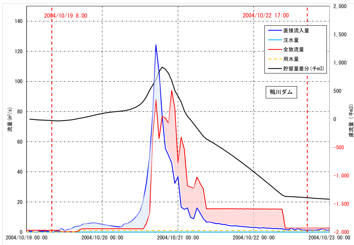
図一 1.4.9(4) ダム貯留高算定事例（鴨川ダム地点：H16.10.20洪水）
