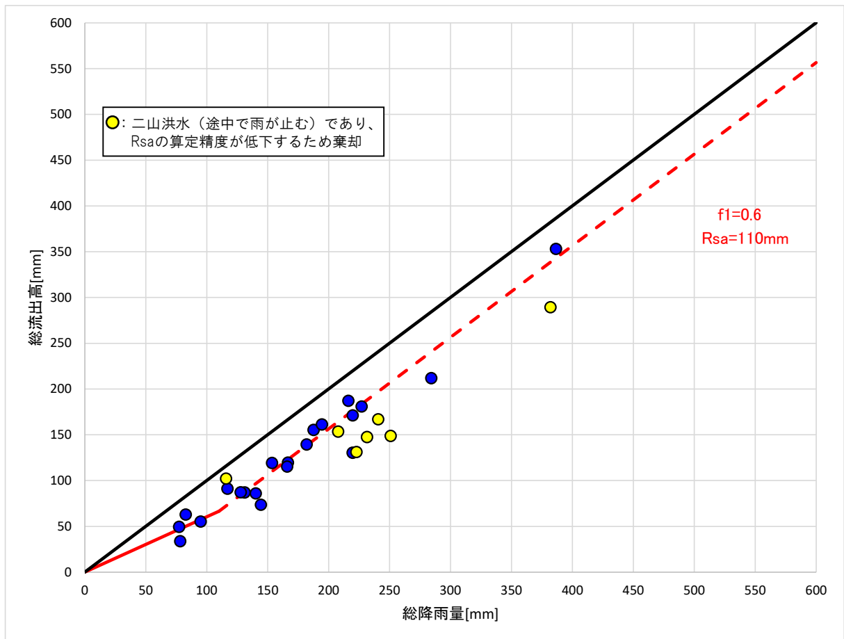
図－ 1.4.10 総降雨量と総流出高の関係（国包地点）
