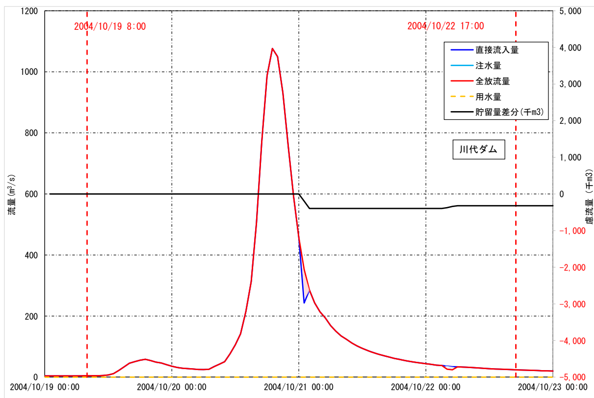
図一 1.4.9(3) ダム貯留高算定事例（川代ダム地点：H16.10.20洪水）
