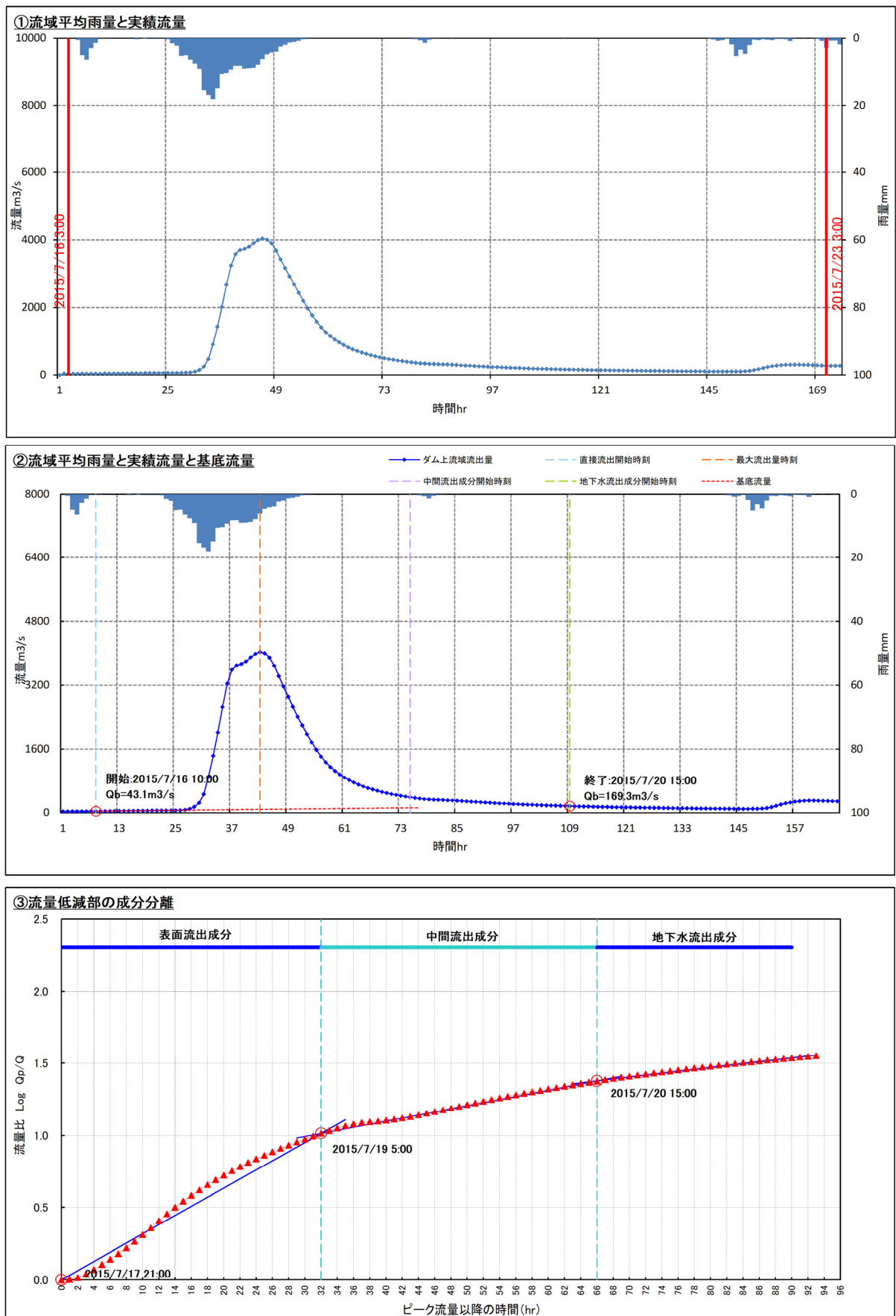
図－ 1.4.8(3) 成分分離の事例（国包地点：H27.7.16 洪水）
