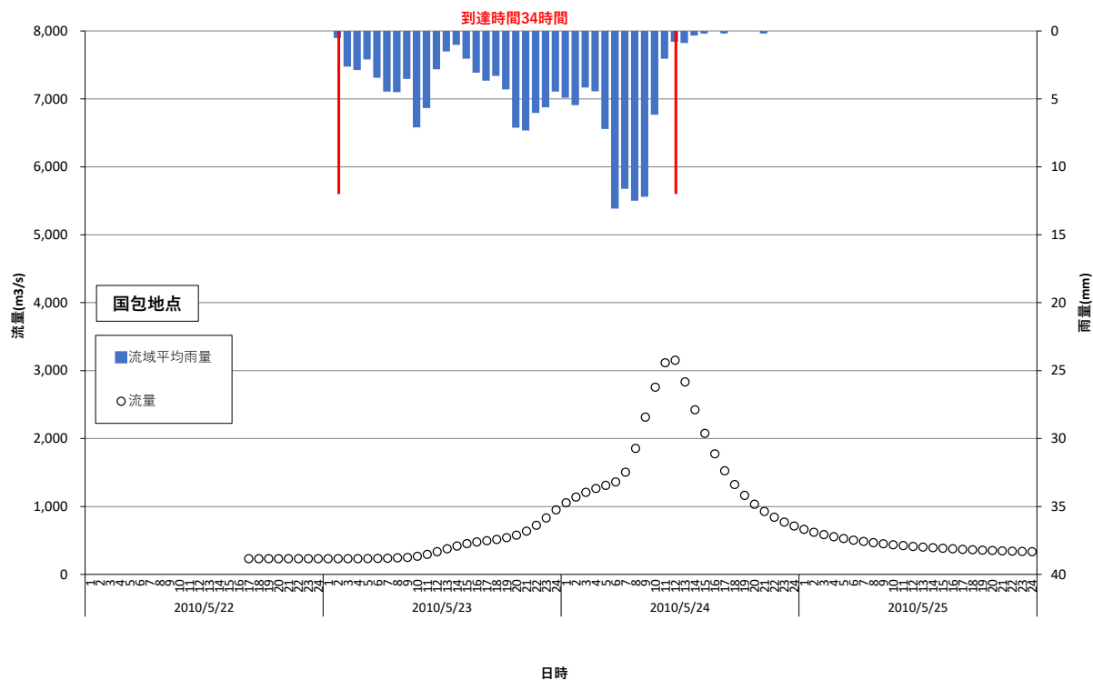
図－ 1.6.2(4) Kinematic Wave 法による洪水到達時間（国包地点 H220524 洪水）
