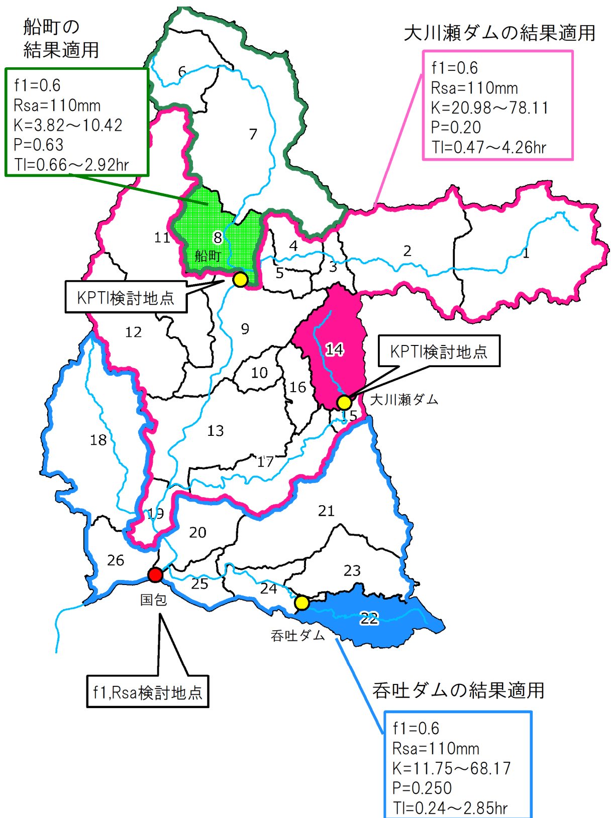
図ー 1. 4. 18 加古川流域における流域定数の設定状況
