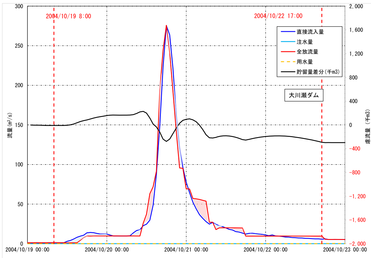
図一 1.4.9(2) ダム貯留高算定事例 (大川瀬ダム地点 : H16.10.20 洪水)
