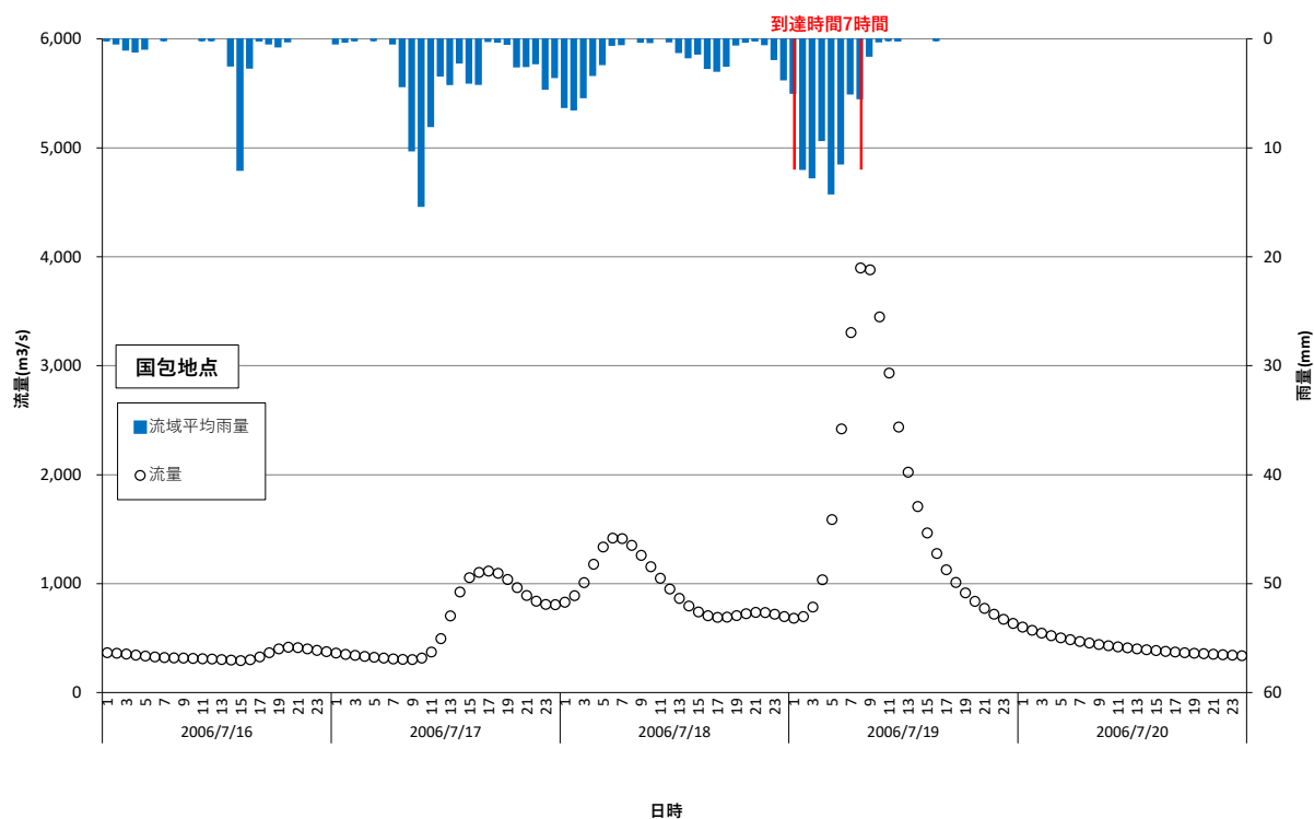
図－ 1.6.2(3) Kinematic Wave 法による洪水到達時間（国包地点 H180719 洪水）
