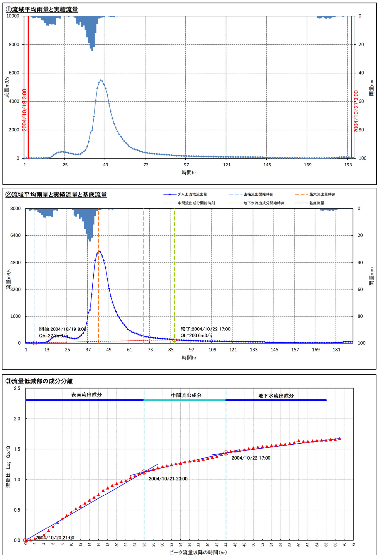
図－ 1.4.8 (1) 成分分離の事例（国包地点：H16. 10. 20 洪水）
