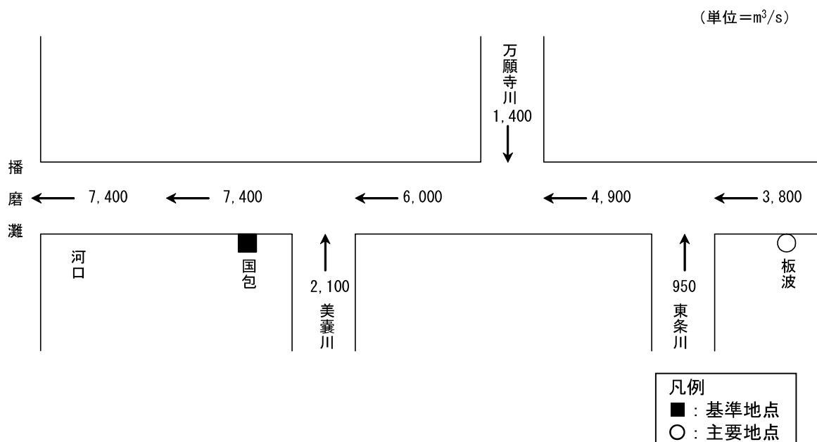
図 6-1 加古川計画高水流量図
