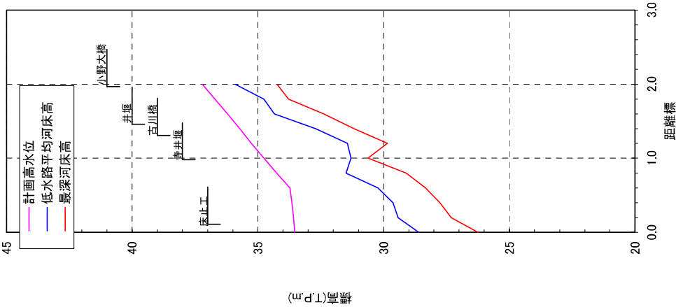
東条川 河道区分縦断面図
