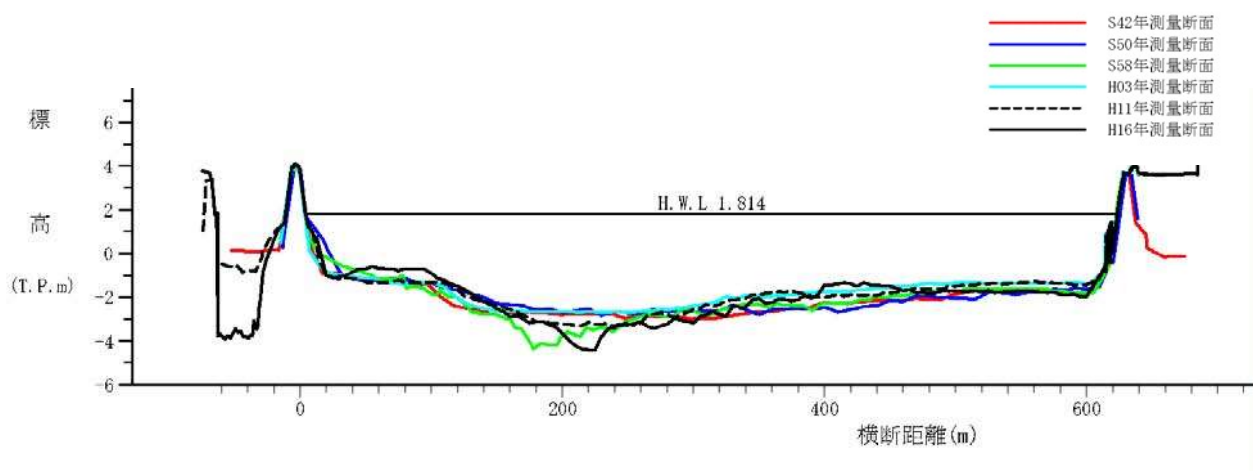
図 3-2 河口部 (0k0) の横断図
