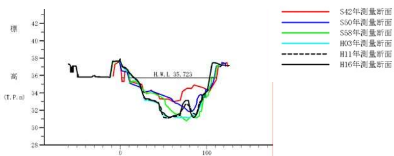
図 2-5 (5) 東条川（古川橋上流 1k4）横断面図
