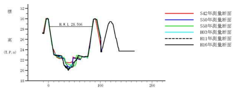
図 2-5 (4) 万願寺川（阿形橋上流 0k2）横断面図
