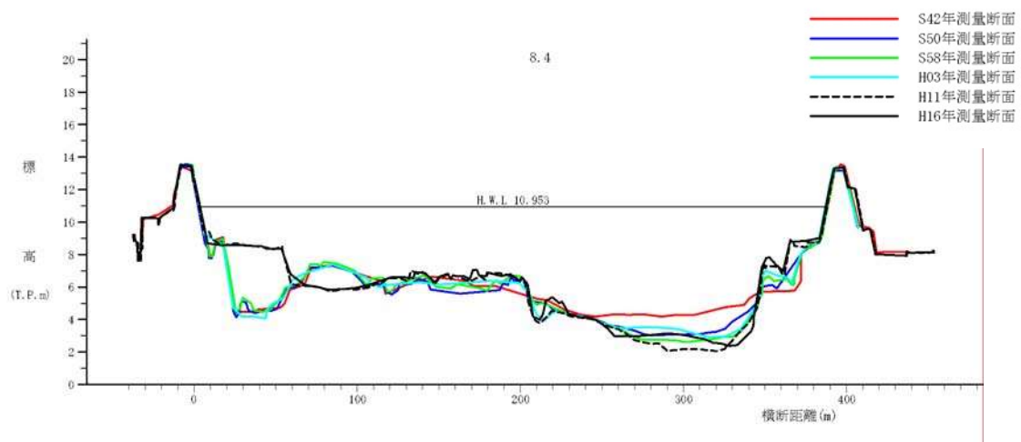
図 2-5 (2) 加古川 下流部（平荘橋上流 9k4）横断図
