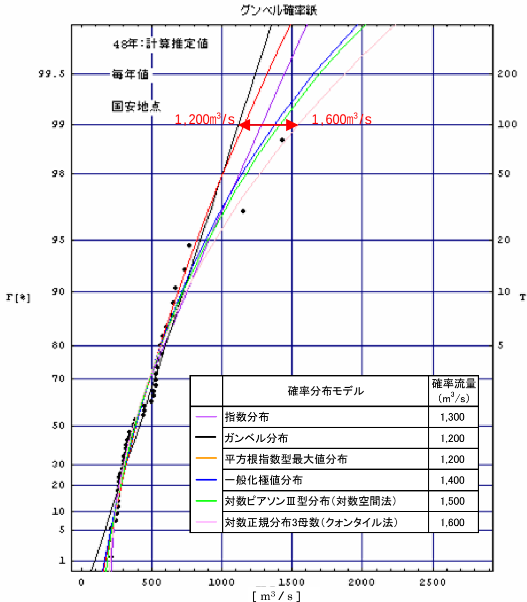
図4 - 9 基準地点国安における流量確率図（S30～H14：48 ケ年）
