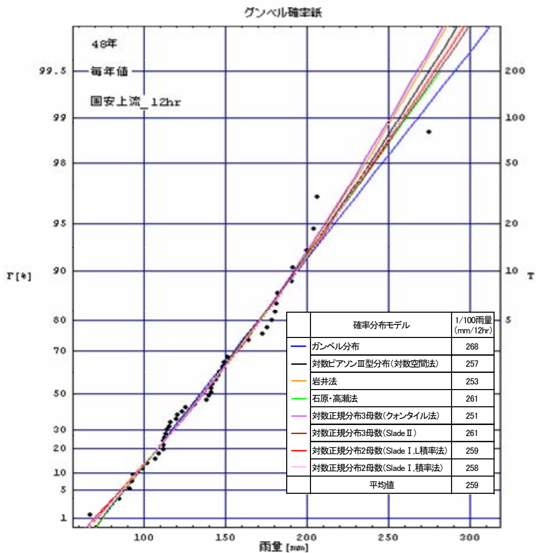
図 4 - 6 基準地点国安における雨量確率図 (S30～H14: 48 ケ年)
