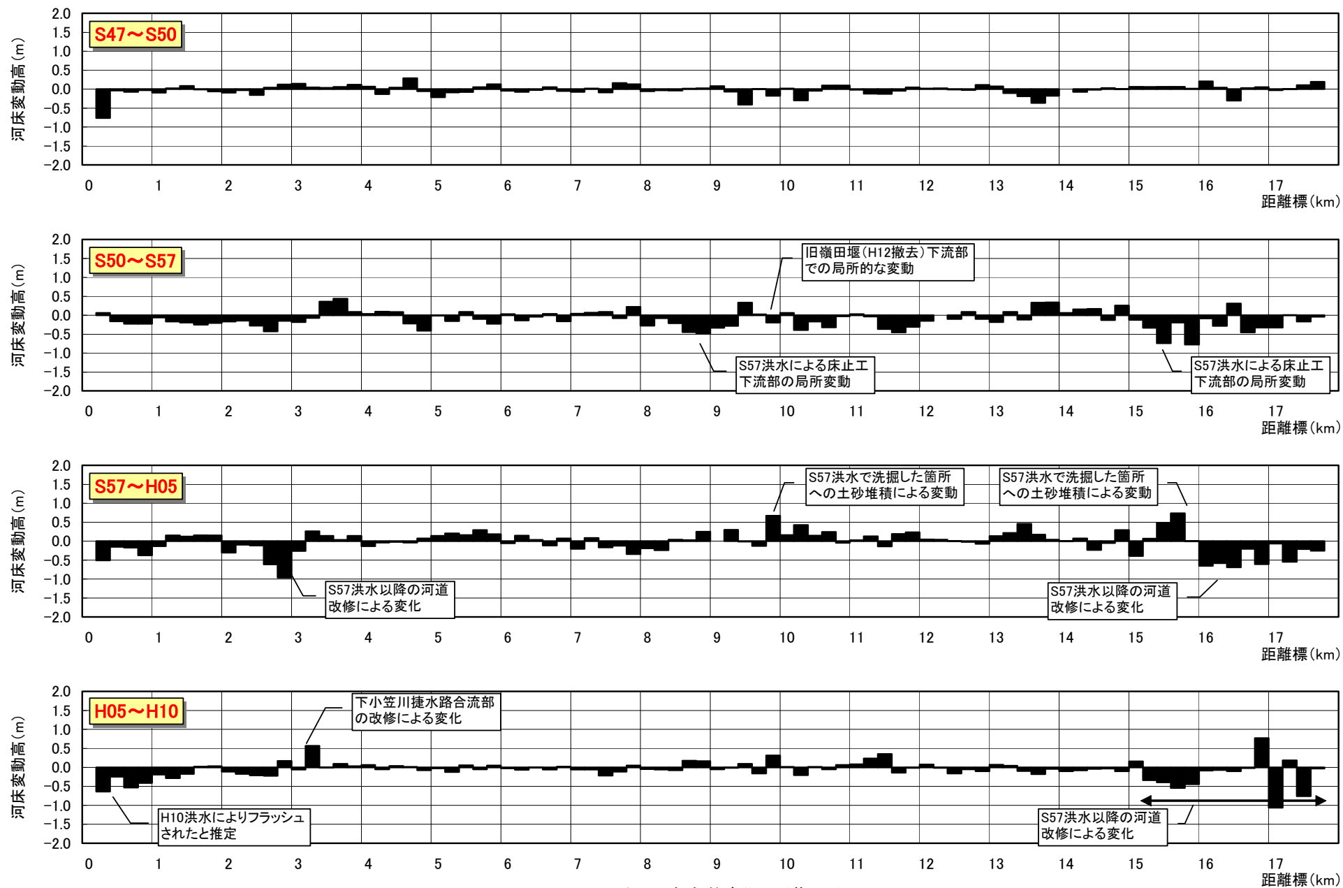
図2-7 河床変動の経年的変化 (菊川)
