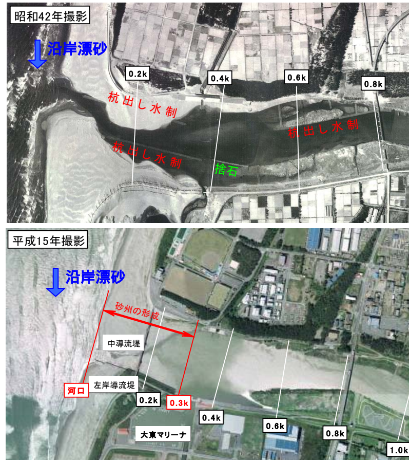
図 3-1 河口部の変遷
