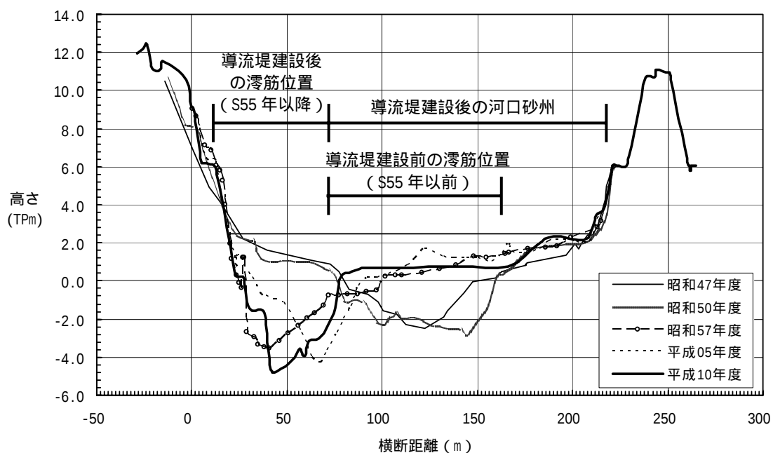
図 3-2 河口部 (0.2k) の横断図
